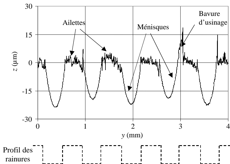
Figure 1.7 : Visualisation des ménisques par microscopie confocale [10]
