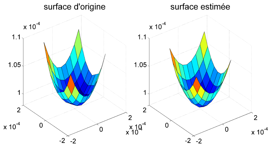
Figure 5.13 : Identification des ménisques à une paraboïde (les distances sont en mètres)
