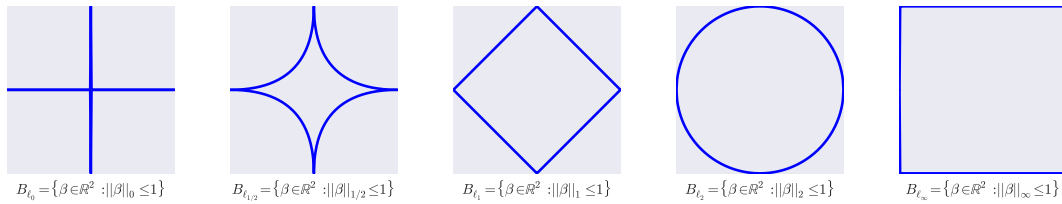
Fig. 1.1 – Boule unité de \mathbb{R}^2 pour les normes \ell_0, \ell_{1/2}, \ell_1, \ell_2 , et \ell_{+\infty} .
