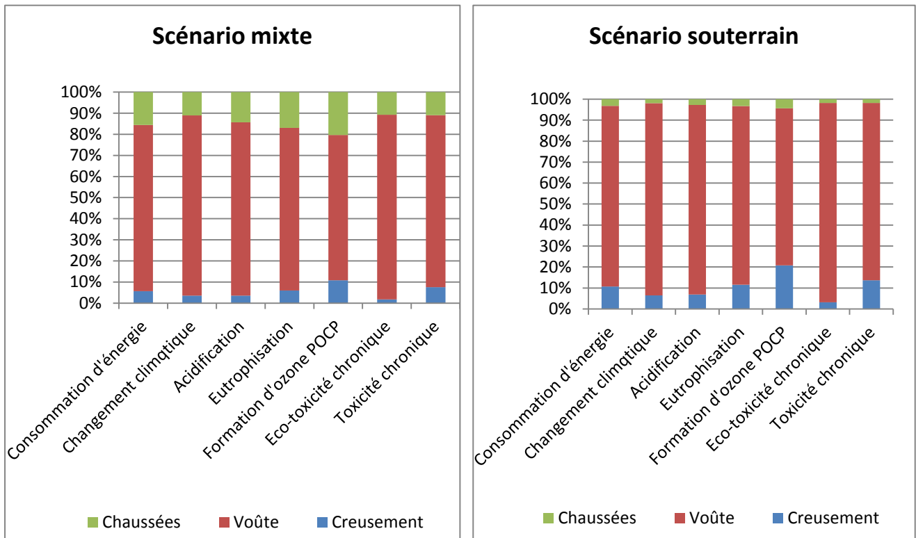
Figure 42 : Contribution des différentes opérations dans la phase de construction - ECORCE
