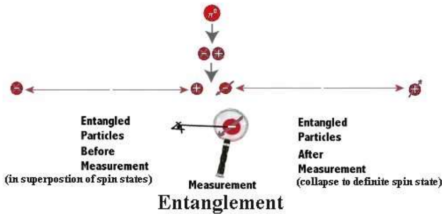
Figure 17 : Schéma représentant l'expérience de pensée d'EPR (extrait de https://quantumweird.wordpress.com/category/epr-pairs/ le 15/05/14)
