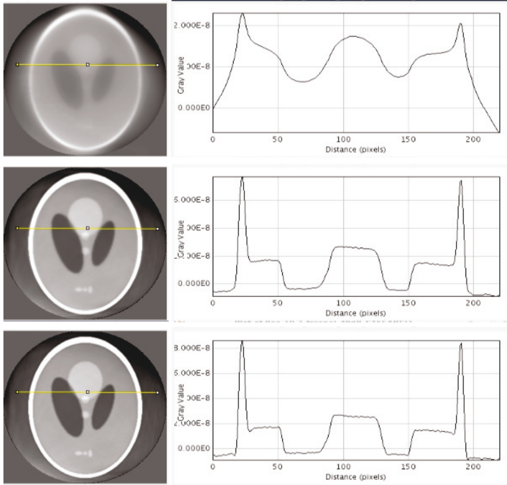
Figure 13: Cartes estimées du décrément de l'indice de réfraction \delta_n à partir de données simulées (modèle de contraste de Fresnel) et bruitées ; la phase est supérieure à 2\pi . Les cartes résultantes (à gauche), et un profil (à droite) sont présentés à la (a) première, (b) vingtième, (c) quarantième itération de l'algorithme proposé.
