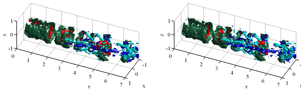
Figure 0.5.8: Isovaleurs de la vitesse axiale à 1.05V_0 (en rouge), où V_0 est la vitesse de sortie du jet, isovaleur de la composante azimuthale de la vorticité \omega_\theta = 2 (vert), isovaleurs de la composante axiale de la vorticité \omega_z = 1.2 (cyan) et \omega_z = -1.2 (bleu) pour tomo-SMART ( Gauche ) et pour PVR-SMART ( Droite ).
