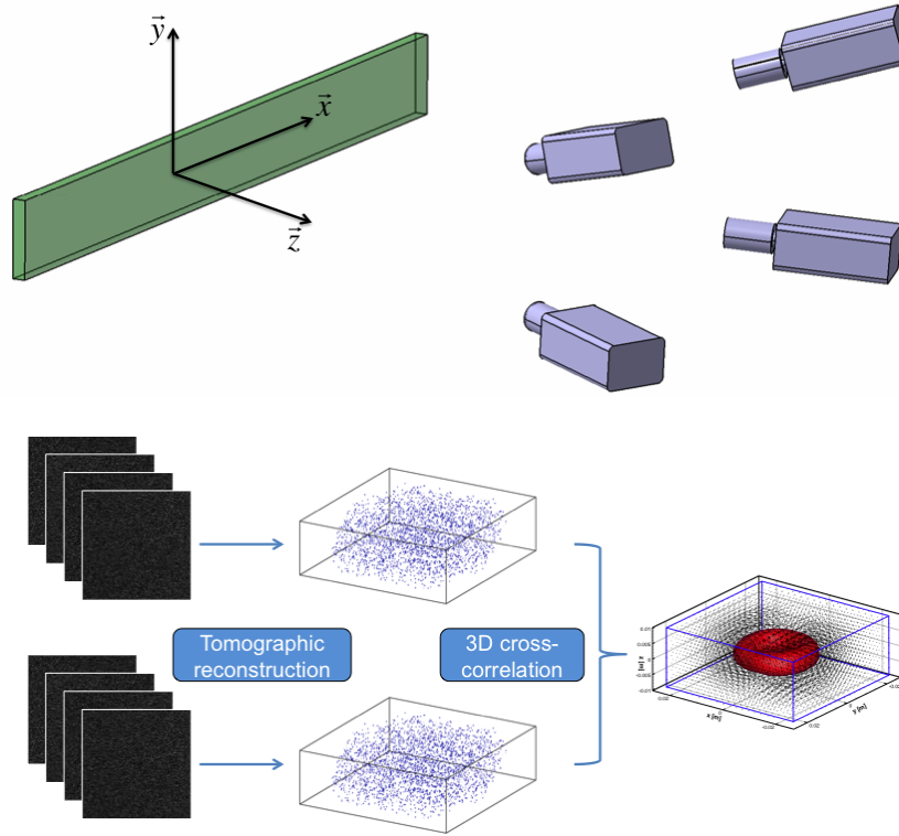
Figure 0.1.1: Principe du dispositif expérimental ( haut ) et des étapes algorithmiques ( bas ) de la PIV tomographique .
