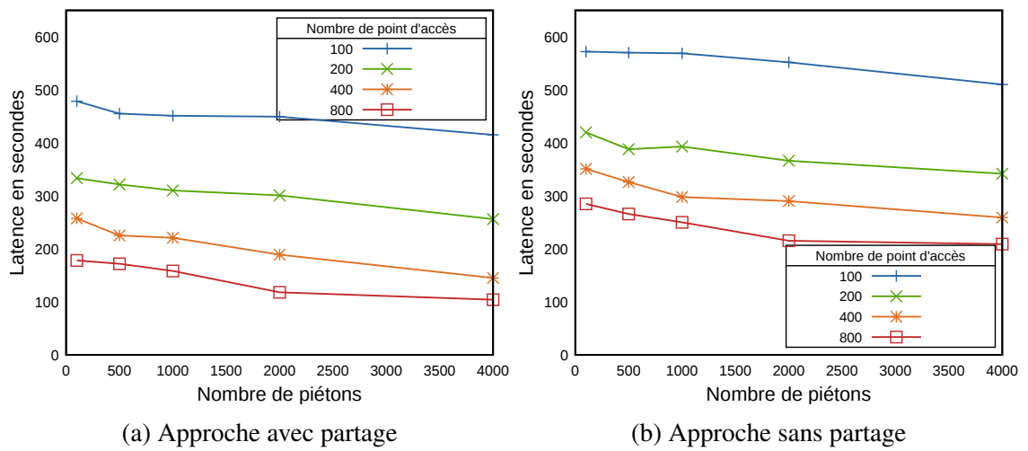
FIGURE 9.7 – latence moyenne des couples requête/réponse
