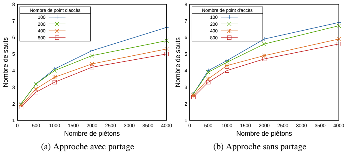
FIGURE 9.8 – Nombre de sauts moyen des couples requête/réponse
