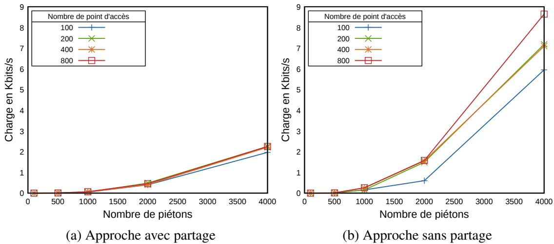
FIGURE 9.9 – charge moyenne par nœud par seconde
