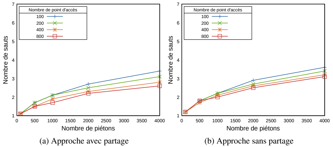
FIGURE 9.6 – Nombre de sauts moyen des réponses
