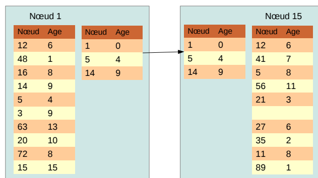
FIGURE 5.4 – Exemple d'une opération d'échange de nœuds
