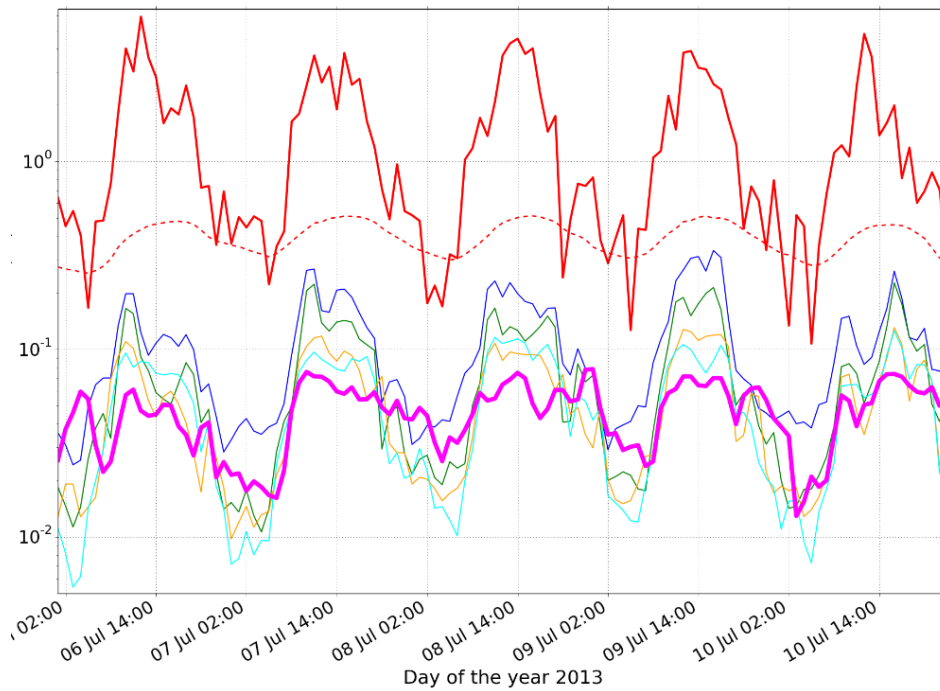
Figure 4-8 : série temporelle de SDV [ \text{min}^{-1} ] pour 5 cibles (cf figure précédente). La courbe magenta en gras correspond à la Tour Eiffel.
