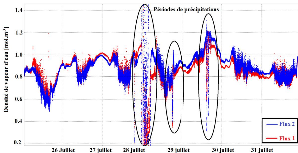
Figure 7-2 : Impact des précipitations sur la mesure de densité de vapeur d'eau [mol.m -3 ] du 25 au 31 juillet. Trois événements précipitants (encadrés en noir) se déclenchent pendant cette période, le 28 et le 29 juillet, perturbant fortement les mesures des deux capteurs licor-7500.
