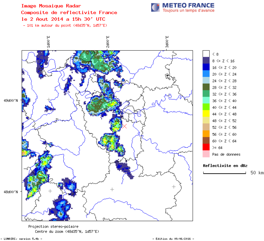
Figure 7-13 : Réflectivité radar autour du SIRTÀ (croix rouge) le 02/08 à 15h30 UTC. Les cellules orageuses se déplacent dans un flux de SSO.
