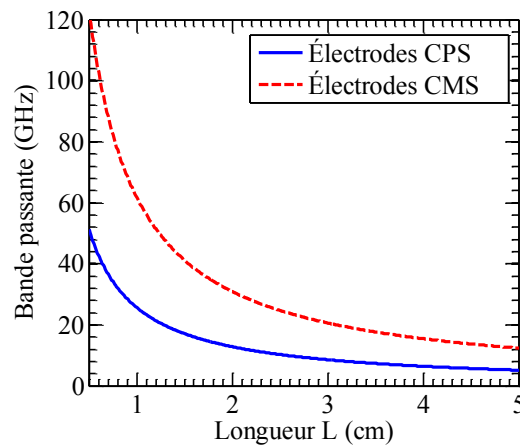
Figure 2.30 – Bande passante du déflecteur en fonction de sa longueur. Seule la désadaptation des vitesses de phase entre ondes optique et HF est prise en compte pour tracer les courbes avec l'équation 2.28. \epsilon_{HF} = 5,44 pour le déflecteur commandé par électrodes CPS et \epsilon_{HF} = 3,50 pour le déflecteur commandé par électrodes CMS.
