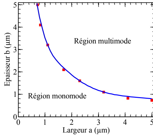
Figure 2.11 – Domaines monomode et multimode en fonction des dimensions du cœur pour un guide qui confine la lumière et dont l'écart d'indice entre cœur et gaine est \Delta n = 0,07 .
