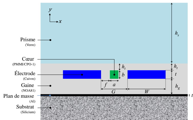
Figure 2.29 – Coupe transversale du déflecteur EO avec un plan de masse métallique pour écranter le wafer Si.
