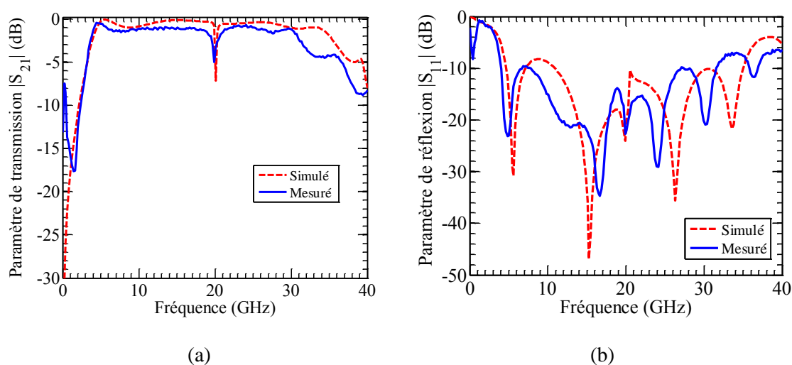
Figure 3.16 – Paramètres-S mesurés et simulés de la transition GCPW-CMS-GCPW sur substrat RO3003™ dont les paramètres géométriques sont dans le Tableau 3.1 ; a) |S_{21}| et b) |S_{11}| .
