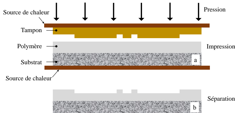
Figure 4.8 – Schéma de principe de la nano-impression thermique (T-NIL).
