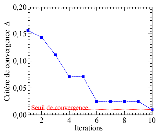
Figure A.3 – Décroissance du coût \Delta en fonction du nombre d'itérations. Dans cet exemple, le paramètre S_{21} est mesuré sur une ligne GCPW réalisée sur un substrat en polymère BCB (cf. Figure A.4).
