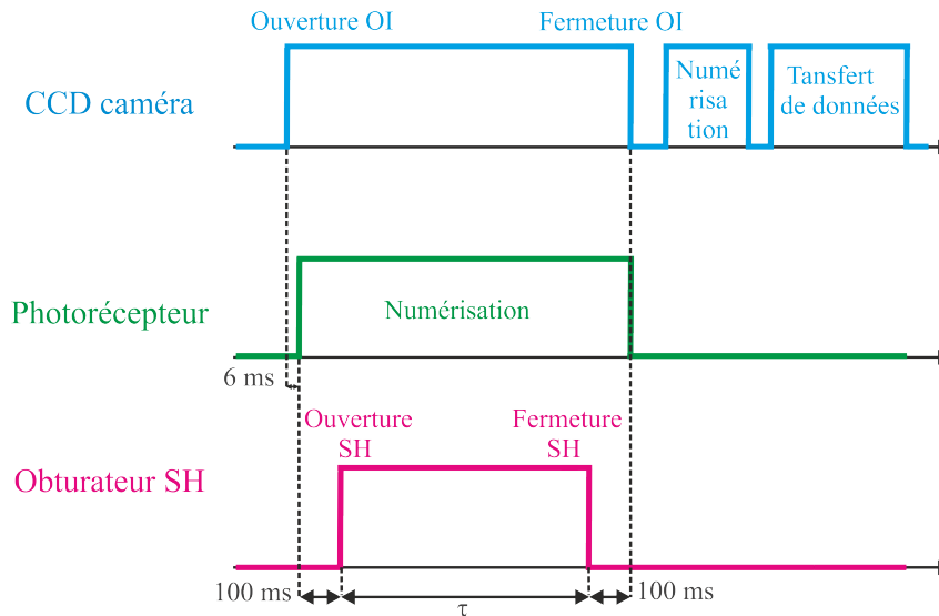
FIGURE 3.24 – Chronogramme d'une acquisition élémentaire réalisée par l'instrument SALSA
