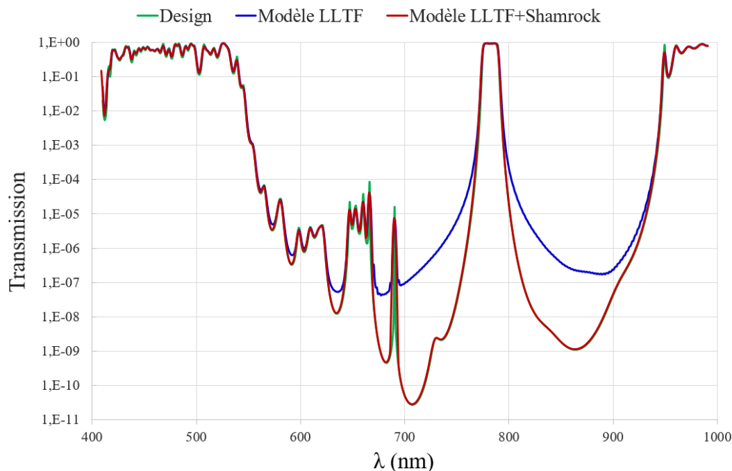
FIGURE 3.45 – Transmission spectrale du filtre F_1 Transmission théorique définie par le design, courbe verte ; transmission simulée correspondant à un simple étage de filtrage (LLTF), courbe bleue ; transmission simulée correspondant aux deux étages de filtrage (LLTF+Shamrock), courbe rouge
