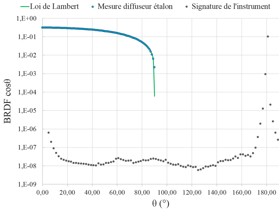
FIGURE 3.65 – Dynamique de mesure de l’instrument en mode diffusomètre sur la plage angulaire [5° - 190°] à la longueur d’onde de 700 nm Courbe verte, loi de LAMBERT; points bleus, mesure du diffuseur étalon; points noirs, signature de l’instrument
