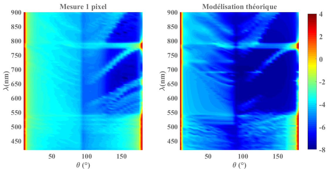
FIGURE 4.24 – Représentation en fausses couleurs de la dépendance spectrale et angulaire de l'indicatrice de diffusion du filtre F 1 graphe de gauche, mesures expérimentales ; graphe de droite, modélisation théorique
