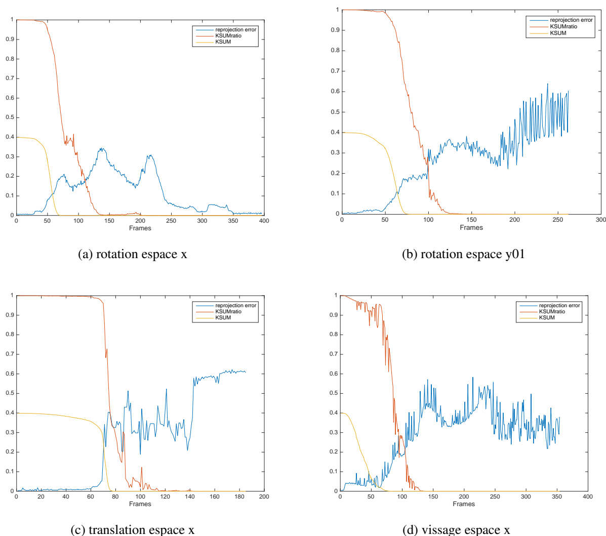
FIGURE 3.10 – Application du KSUM et KSUMratio sur les valeurs de l’erreur de reprojection enregistrées suivant différents mouvements des pièces.
