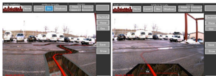
FIGURE 2.7 – Smart Vidente pour l'ingénierie civile. [Schall et al., 2013]
