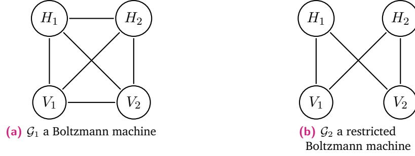
Fig. 2.22. Two UGs \mathcal{G}_1, \mathcal{G}_2 such that I(\mathcal{G}_1) \neq I(\mathcal{G}_2) but I(\mathcal{G}_1)^\emptyset_H = I(\mathcal{G}_2)^\emptyset_H .
