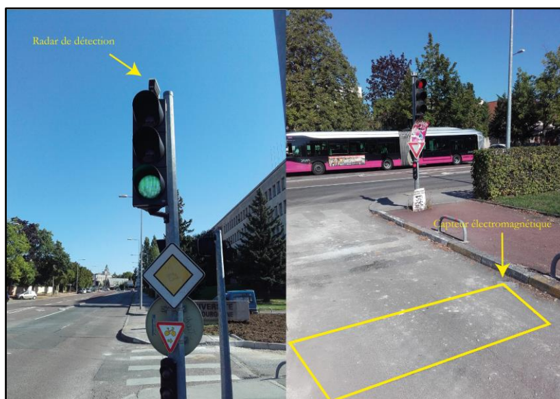
Figure 1.24 : Illustration des dispositifs de détection autonomes pour les feux tricolores sur un même carrefour entre le Boulevard Gabriel et l'Avenue Alain Savary (à gauche : un radar de détecteur de présence ; à droite : un capteur électromagnétique)
