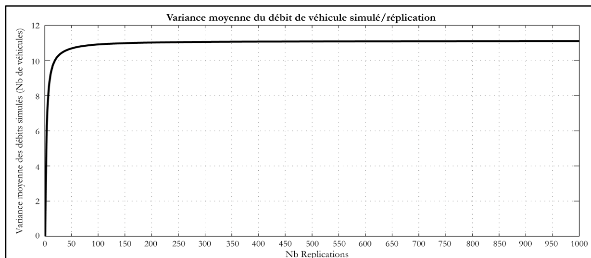
Figure 2.34 : Analyse de la réplification de SCAUP par le signal de variance moyen de débit de véhicules simulés (1000 réplifications)
