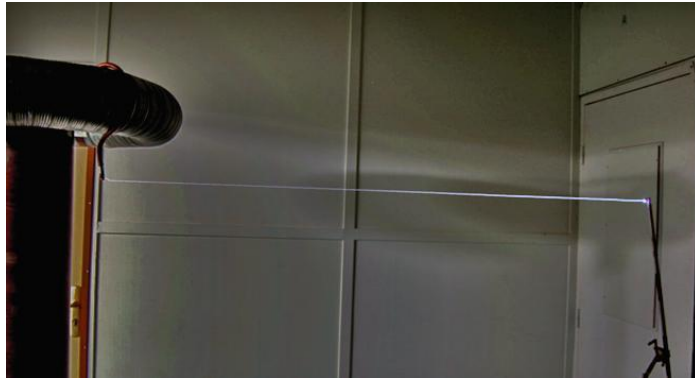
Figure 4.14 : Photographie d’une décharge Tesla de 1,7 m de long guidée par un faisceau laser filamenté. Le laser vient de la gauche.
