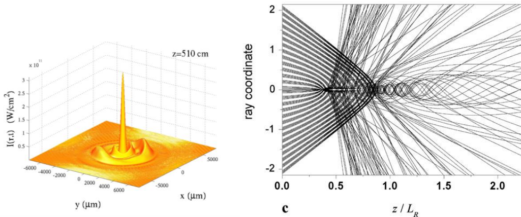
Figure 1.3 : A gauche : profil d’intensité dans un faisceau au cours de la filamentation. A droite : Calcul de tracé de rayon d’une impulsion filamentée illustrant le rôle du bain d’énergie et les cycles de refocalisation [Geints2012].
