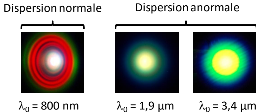
Figure 2.6 : Photographie de l’émission conique visible mesurée en sortie de filaments de quelques puissances critiques dans la silice pour trois longueurs d’onde différentes.
