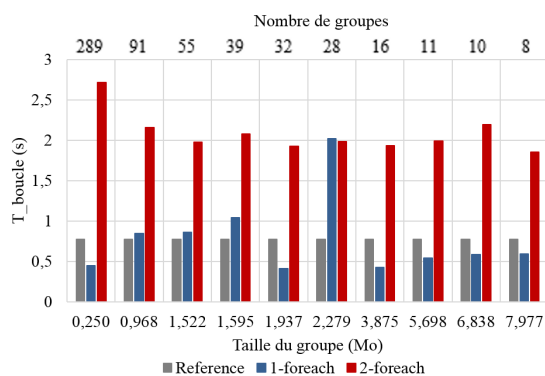
FIGURE 6.4 – Variation du temps d’exécution de la boucle élémentaire en fonction de la taille du groupe avec 16 threads pour une simulation du jeu de données Mara_mdm
