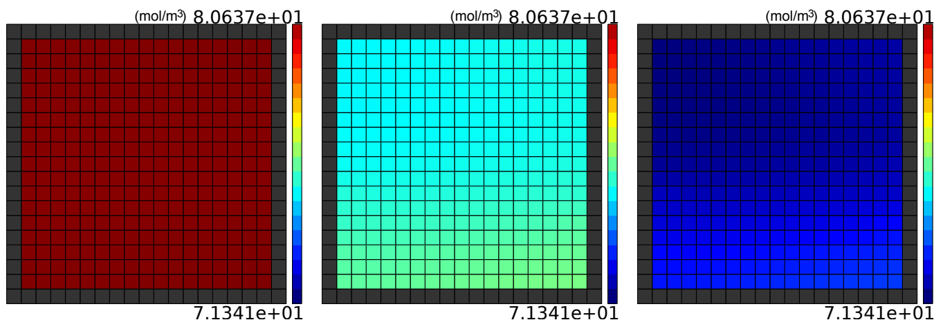
FIGURE 5.45 – Évolution de la répartition de densité molaire de H_2 dans la couche catalytique en fonction du courant (du plus bas (5A) au plus haut (40A))
