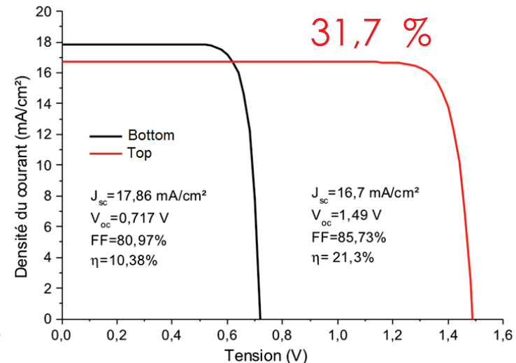
Configuration classique
