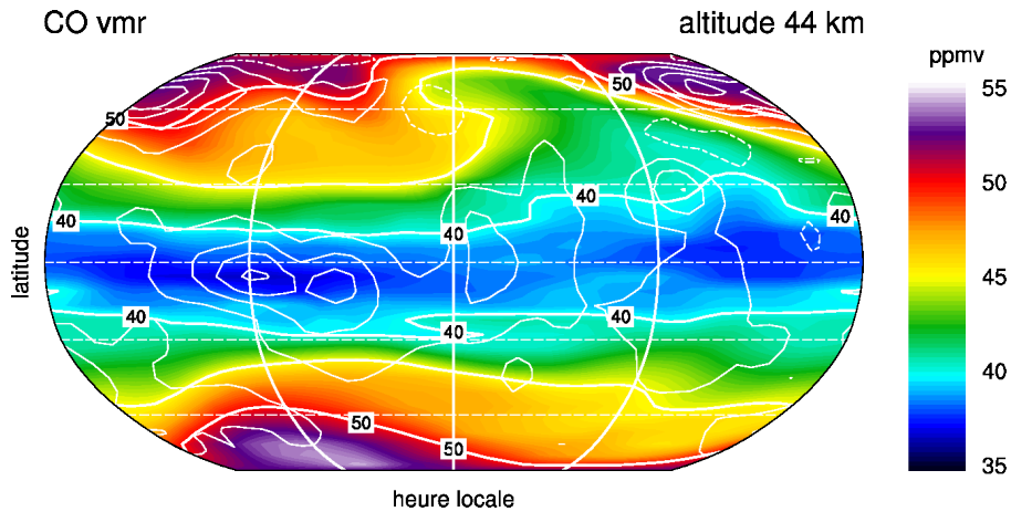
FIGURE 8.10 – Carte à 44 km du rapport de mélange de CO après de 100j vénusiens simulés où CO est initialisé à 25 ppmv dans l’atmosphère profonde. La carte est centrée au midi local
