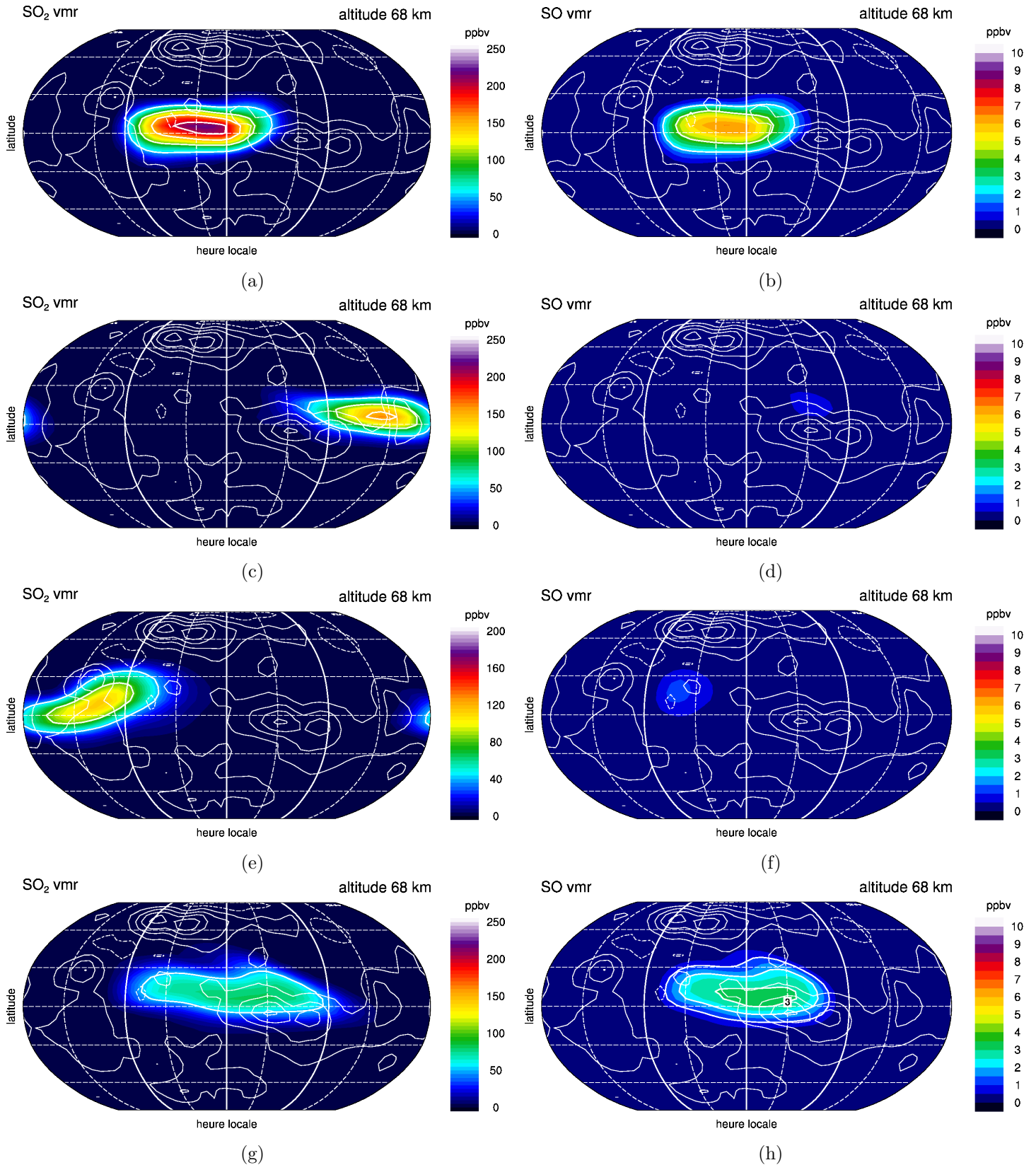
FIGURE 8.68 – Cartes à 68 km du rapport de mélange de SO 2 et SO lors d'un épisode d'instabilité équatoriale. La première carte est calculée après 92,5 jours vénusiens simulés. Chaque carte est prise à un intervalle d'un quarantième de jour vénusien, donc environ 3 jours terrestres. Les cartes sont centrées sur le midi local. Les méridiens en blanc représentent d'Ouest en Est le coucher, le midi et le lever de Soleil.
