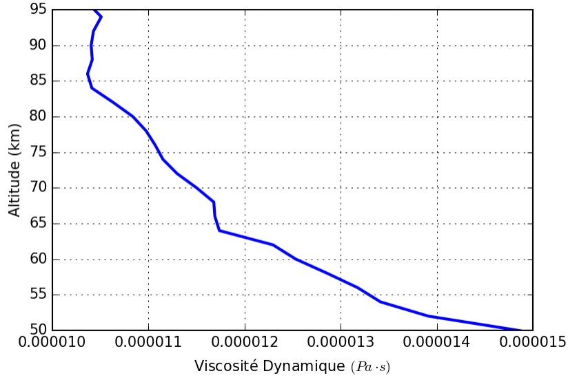
FIGURE 5.5 – Profil vertical de la viscosité dynamique exprimée à partir de Jones (1924) et des données de Johnston and Grilly (1942) pour le CO 2 .
