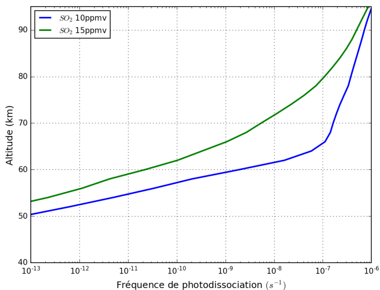
FIGURE 8.32 – Profils verticaux des fréquences de photodissociation ( \text{s}^{-1} ) de HCl calculées avec une initialisation de \text{SO}_2 dans l'atmosphère profonde égale à 10 ppmv (bleu) ou 15 ppmv (vert).
