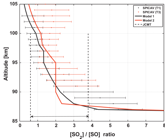
FIGURE 8.72 – Profils verticaux du rapport [SO 2 ]/[SO] mesuré avec SPICAV par Belyaev et al. (2012) . (T1) et (T3) correspondent à deux profils de température différents pour l'analyse des données. Model 1 et Model 2 sont les résultats du modèle 1D de Zhang et al. (2012) .
