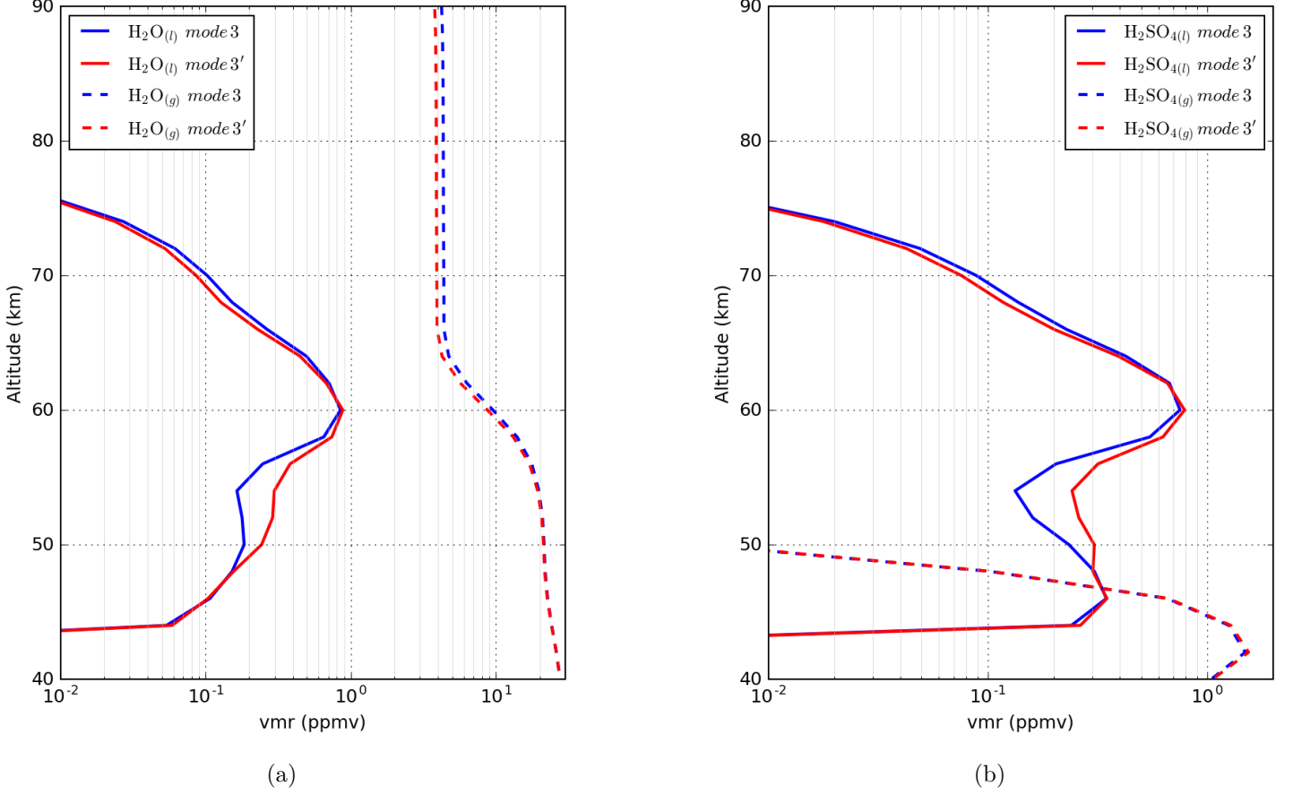
FIGURE 7.14 – Profils verticaux des phases liquides et gazeuses de \text{H}_2\text{O} (à gauche) et \text{H}_2\text{SO}_4 (à droite). Tous les résultats sont issus de simulations avec une initialisation en \text{SO}_2 dans l'atmosphère profonde de 10 ppmv. Le mode 3' consiste en un cœur solide recouvert d'une pellicule d'acide sulfurique. Le cœur représente environ 98,5% de la masse de la gouttelette.
