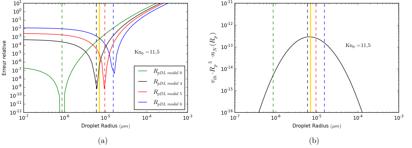
FIGURE B.3 – Détermination de R_{p\star} pour une distribution à Knudsen caractéristique de 11,54. (a) représente l'erreur relative entre le calcul de l'intégrande théorique et celui issu du développement limité en R_{pDL\ mode\ X} . Les traits pleins sont l'erreur relative et les pointillés verticaux marquent la valeur du R_{pDL\ mode\ X} choisie. (b) représente la valeur de l'intégrande selon le rayon. La ligne verticale pleine et dorée représente la valeur du rayon pour lequel l'intégrande est maximale.
