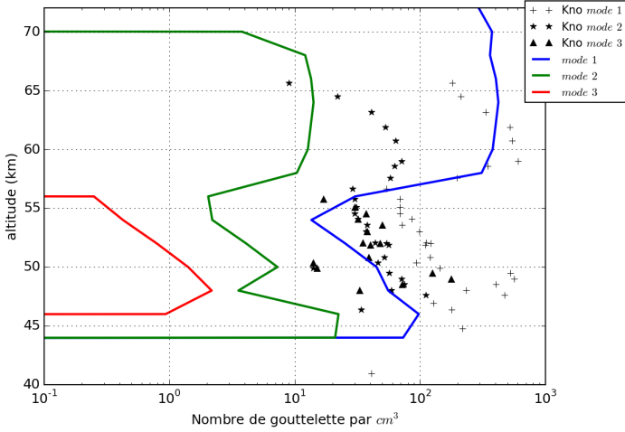
(c) Simulation initialisée avec 20 ppmv de \text{SO}_2
