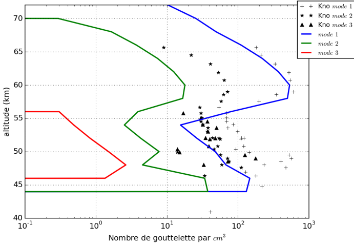
(a) Simulation initialisée avec 10 ppmv de \text{SO}_2
