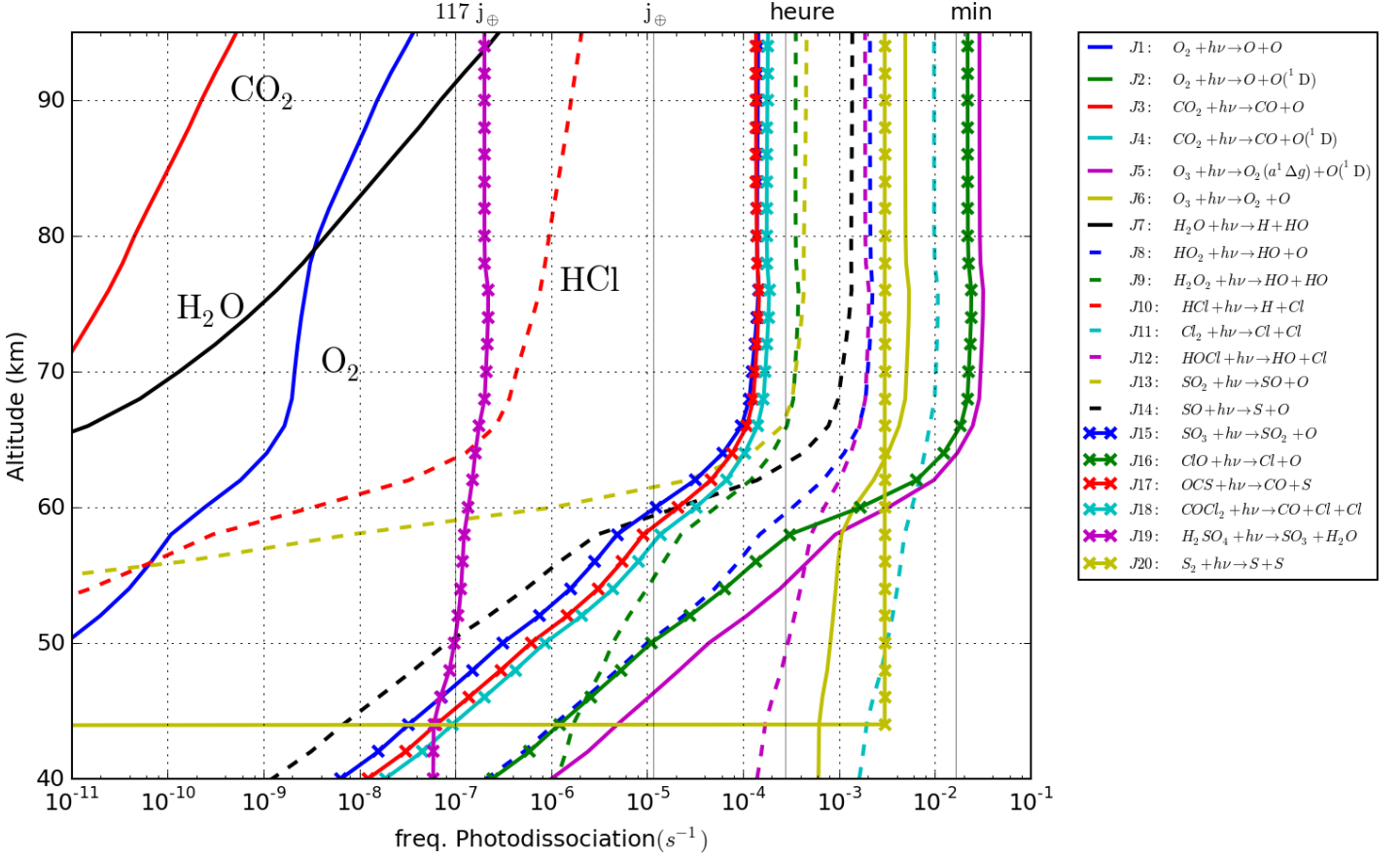
FIGURE 4.1 – Fréquences de photodissociation pour un angle solaire zénithal \zeta = 45^\circ . Les profils de [CO_2] et [SO_2] utilisés sont une moyenne diurne calculée à partir d'une simulation 3D de plus 100 jours vénusiens. Les traits fins grisés verticaux correspondent à l'inverse d'un temps caractéristique. Ainsi, de gauche à droite on a la fréquence qui correspond à l'inverse de la durée du jour vénusien (117 j ⊕ ), au jour terrestre, à l'heure et à la minute.
