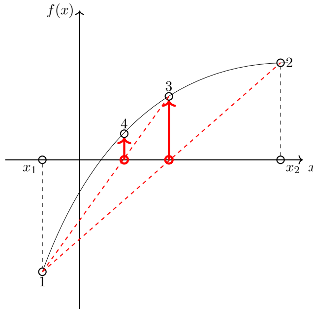
FIGURE A.1 – Schématisation de la méthode "false position". Les points 1 et 2 délimitent l'intervalle où la fonction f(x) a une seule et unique racine. la première interpolation entre ces deux points mènent au point 3. La méthode "false position" garde en mémoire le point précédent si celui-ci est de signe différent du point nouvellement interpolé. De fait, on garde en mémoire le point 1 et on interpole alors entre 1 et 3 et non entre 2 et 3. Ceci nous permet de rester dans l'intervalle [x_1, x_2] et d'encadrer tout le temps la racine. la seconde interpolation nous mène au point 4. On réitère ce processus jusqu'à ce que le point interpolé soit aussi proche de 0 que désiré.
