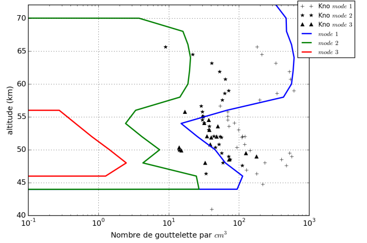
(b) Simulation initialisée avec 15 ppmv de \text{SO}_2
