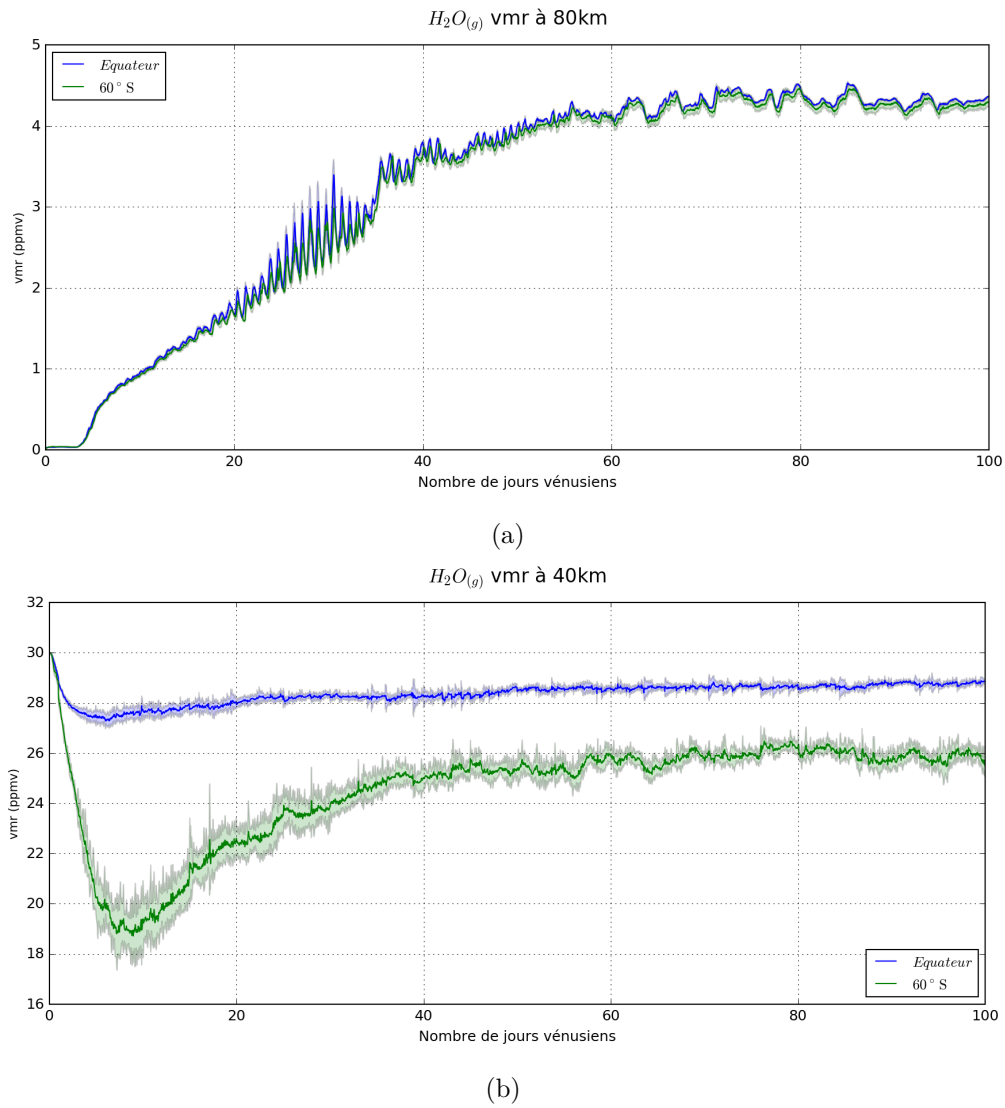
FIGURE 8.46 – Variation temporelle de la moyenne globale du rapport de mélange de H_2O_{(g)} calculée par le modèle à (a) 80 km et (b) 40 km. H_2O est initialisé à 30 ppmv dans l’atmosphère profonde. Les enveloppes colorées représentent la déviation standard en longitude des valeurs du rapport de mélange de H_2O .
