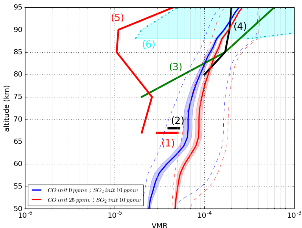
FIGURE 8.16 – Profils du rapport de mélange moyen global de CO. Les enveloppes colorées représentent la déviation standard pondérée en latitude de la moyenne zonale et les tirets fins les minimums/maximums du rapport de mélange de CO. Les observations de CO sont : (1) VEX/VIRTIS Irwin et al. (2008) ; (2) Connès et al. (1968) et Krasnopolsky (2010b) ; (3) Lellouch et al. (1994) ; (4) Clancy et al. (2012) ; (5) VEX/SOIR Vandaele et al. (2008) ; (6) VEX/SOIR Vandaele et al. (2016) min/max.
