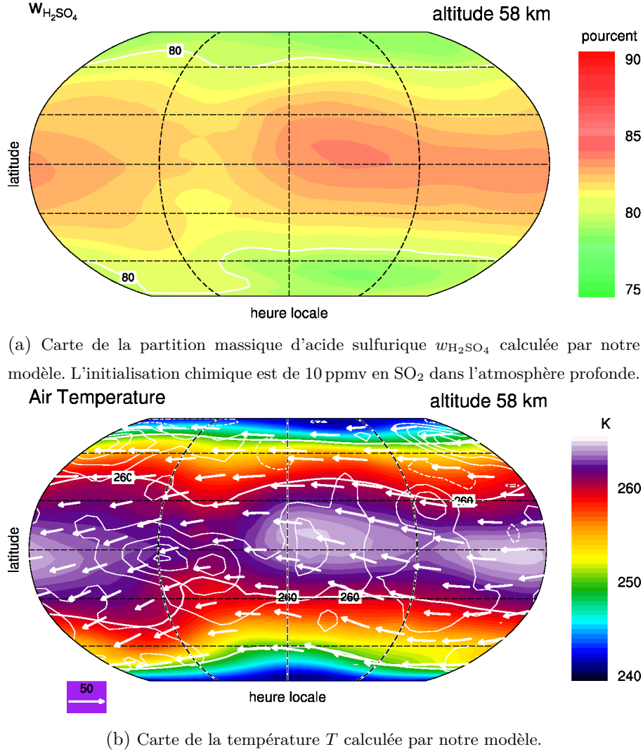
FIGURE 7.7 – Comparaison de la fraction massique d'acide sulfurique w_{\text{H}_2\text{SO}_4} et de la température calculée par le GCM à 58 km.
