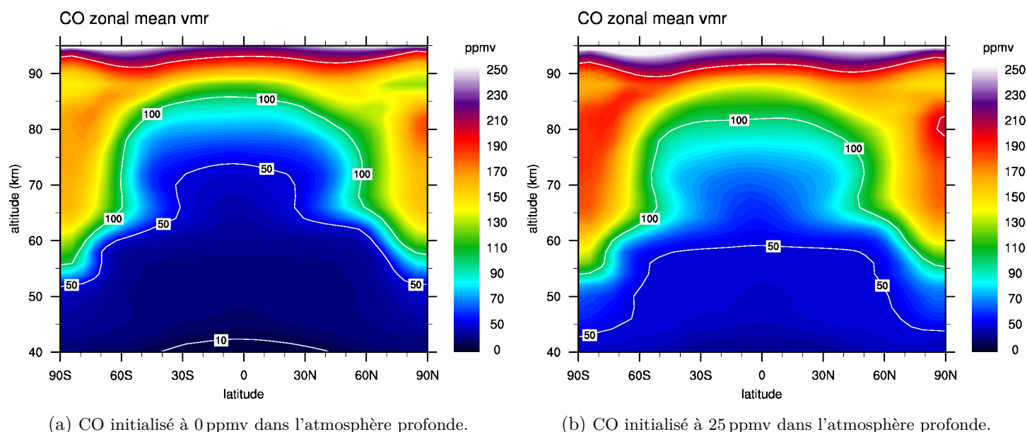
FIGURE 8.5 – Moyenne zonale de CO après 100 jours vénusiens simulés selon différentes initialisations du rapport de mélange de CO dans l'atmosphère profonde.
