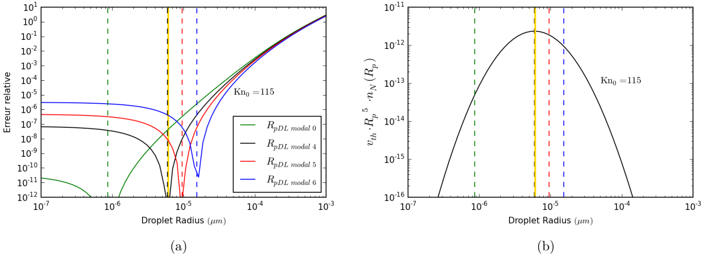
FIGURE B.4 – Détermination de R_{p\star} pour une distribution à Knudsen caractéristique de 115,4. (a) représente l'erreur relative entre le calcul de l'intégrande théorique et celui issu du développement limité en R_{pDL\ mode\ X} . Les traits pleins sont l'erreur relative et les pointillés verticaux marquent la valeur du R_{pDL\ mode\ X} choisie. (b) représente la valeur de l'intégrande selon le rayon. La ligne verticale pleine et dorée représente la valeur du rayon pour lequel l'intégrande est maximale.
