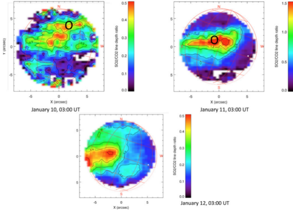
FIGURE 8.66 – Variation sur court terme de l’abondance en \text{SO}_2 au-dessus du sommet nuageux. La figure représente l’évolution du rapport de profondeur des lignes spectroscopiques de \text{SO}_2 et \text{CO}_2 observées à 24 h d’intervalle depuis la Terre par Encrenaz et al. (2012) grâce à l’instrument TEXES, un spectromètre imageur dans l’IR à haute résolution de la NASA. Le 10 Jan et 12 Jan, le \text{SO}_2/\text{CO}_2 line depth ratio égal à 0.45 correspond à un rapport de mélange de \text{SO}_2 de 60 ppbv et le 11 Jan, 1.5 à un rapport de mélange égal à 100 ppbv.
