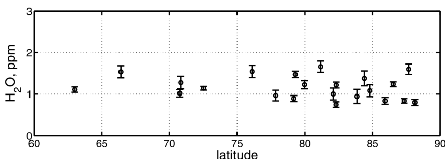
FIGURE 8.53 – Variation en latitude du rapport de mélange de \text{H}_2\text{O}_{(g)} , moyenné entre 75 à 112 km, observé par Fedorova et al. (2008) avec l'instrument SOIR à bord de la sonde Venus Express .
