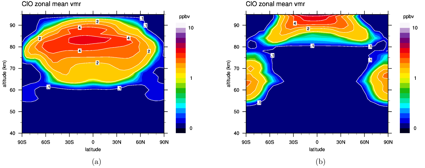
FIGURE 8.40 – Moyennes zonales de ClO selon différentes initialisations de l'atmosphère profonde en SO 2 après 100 jours vénusiens simulés. (a) simulation où SO 2 est initialisé à 10 ppmv et (b) à 15 ppmv.
