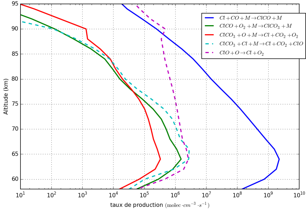
FIGURE 3.5 – Taux de productions des réactions impliquées dans les cycles (3.9) et (3.10). Avec en traits pleins les réactions qui forment le cycle (3.9) et en pointillés les deux réactions supplémentaires qui font appel à ClO comme espèce intermédiaire. Les constantes de réactions sont celles utilisées par Yung and DeMore (1982). Les concentrations des espèces utilisées pour calculer le taux de production sont issues de notre modèle chimique couplé au GCM et moyennées sur une journée vénusienne.
