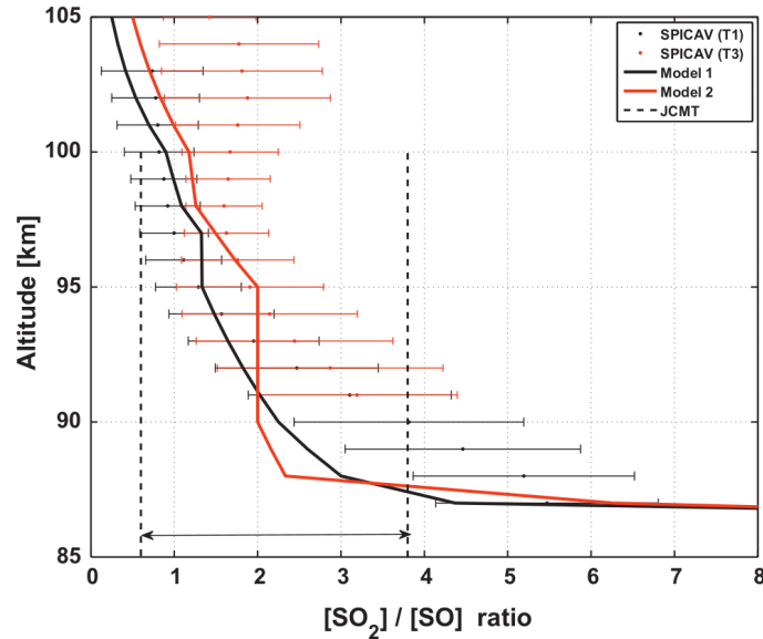
FIGURE 8.72 – Profils verticaux du rapport [SO 2 ]/[SO] mesuré avec SPICAV par Belyaev et al. (2012) . (T1) et (T3) correspondent à deux profils de température différents pour l'analyse des données. Model 1 et Model 2 sont les résultats du modèle 1D de Zhang et al. (2012) .
