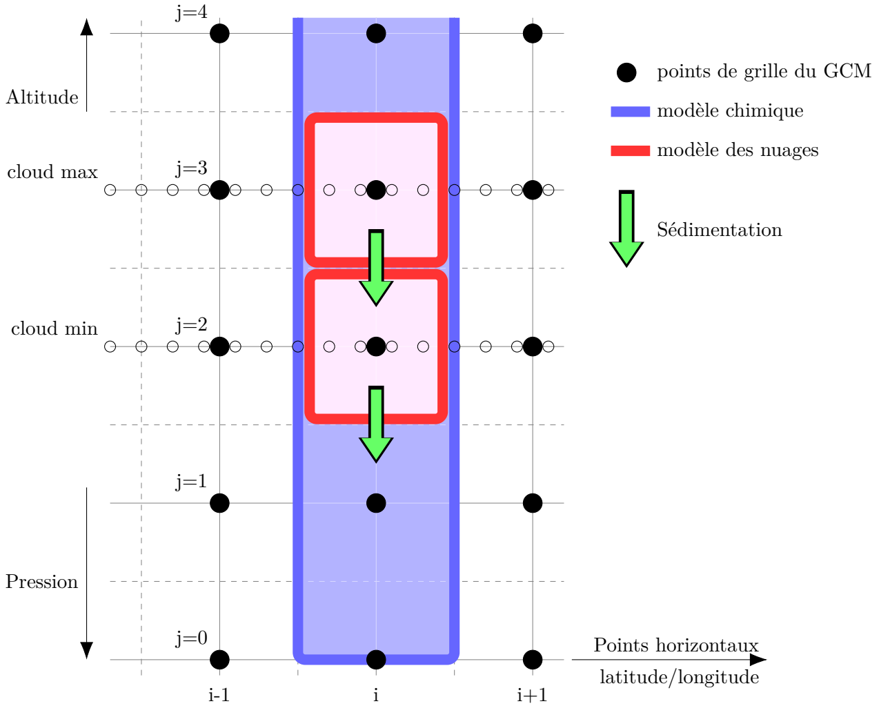
FIGURE 6.1 – Représentation du fonctionnement des modèles des nuages et de la chimie de Vénus. En chaque point horizontal i , le modèle chimique calcule sur toute la colonne d'atmosphère l'évolution des traceurs chimiques due à la chimie pendant le pas de temps défini par la partie physique du GCM. Entre les niveaux, fixés par l'utilisateur, cloud min et cloud max , le modèle des nuages de Vénus calcule la partition massique en acide sulfurique des gouttelettes w_{\text{H}_2\text{SO}_4} et les parties condensées \text{H}_2\text{O}_{(l)} et \text{H}_2\text{SO}_{4(l)} . Ensuite, la sédimentation est calculée à chaque point j de la grille comme la somme des flux de sédimentation de la couche j et de la couche du dessus, j + 1 .
