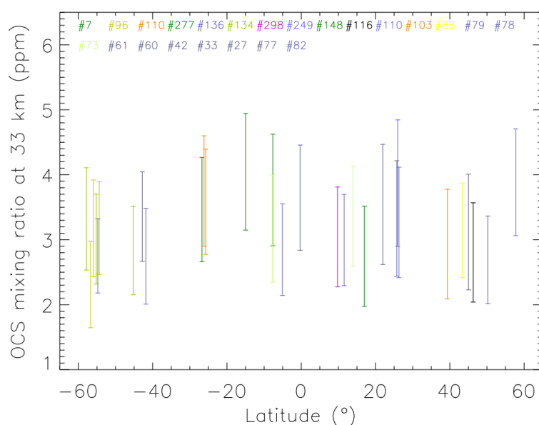
FIGURE 8.75 – Variation en latitude de l'abondance de OCS, mesures dans l'infrarouge de VIRTIS (Marcq et al., 2008). Les abondances trouvées correspondent à des altitudes sous la couche nuageuse vénusienne, aux alentours de 33 km du côté nuit.
