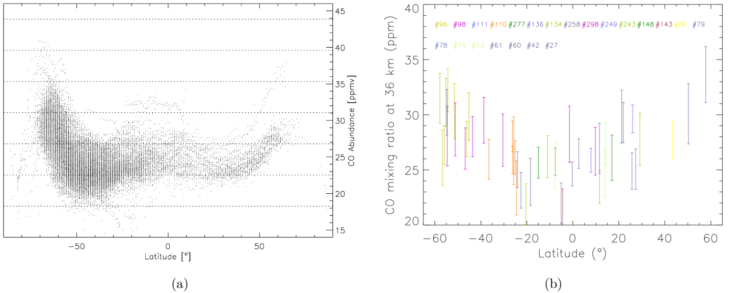
FIGURE 8.7 – Rapport de mélange de CO observé à ~ 36 km. (a), résultats de Tsang et al. (2009) et (b) résultats de Marcq et al. (2008) qui utilisent tous deux les données de l'instrument VIRTIS à bord de Venus Express .
