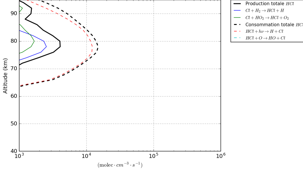
FIGURE 8.33 – Profils verticaux des termes de production et de perte de HCl avec une atmosphère profonde initialisée à 15 ppmv en \text{SO}_2 . Seules les réactions prépondérantes sont affichées.
