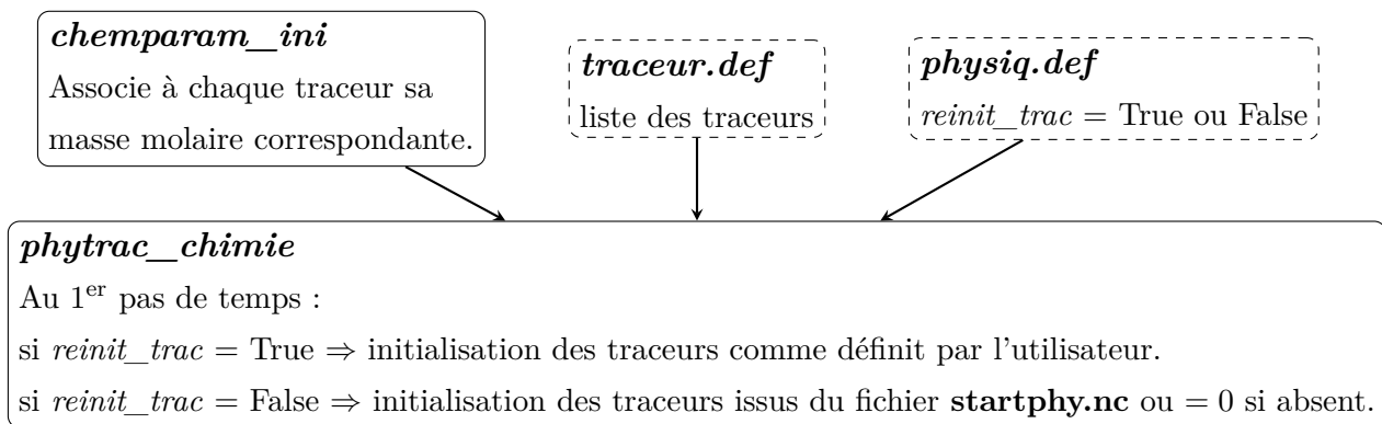
FIGURE 6.3 – Schématisation de l'initialisation des traceurs dans phytrac_chimie . traceur.def est un fichier texte qui liste les traceurs de la chimie-microphysique et physiq.def est un fichier texte qui gère les valeurs de certaines constantes et arguments logiques. chemparam_ini est une sous-routine qui initialise au premier pas de temps les masses molaires des espèces chimiques. startphy.nc est un fichier de sauvegarde de variables physiques et des traceurs de la précédente simulation.
