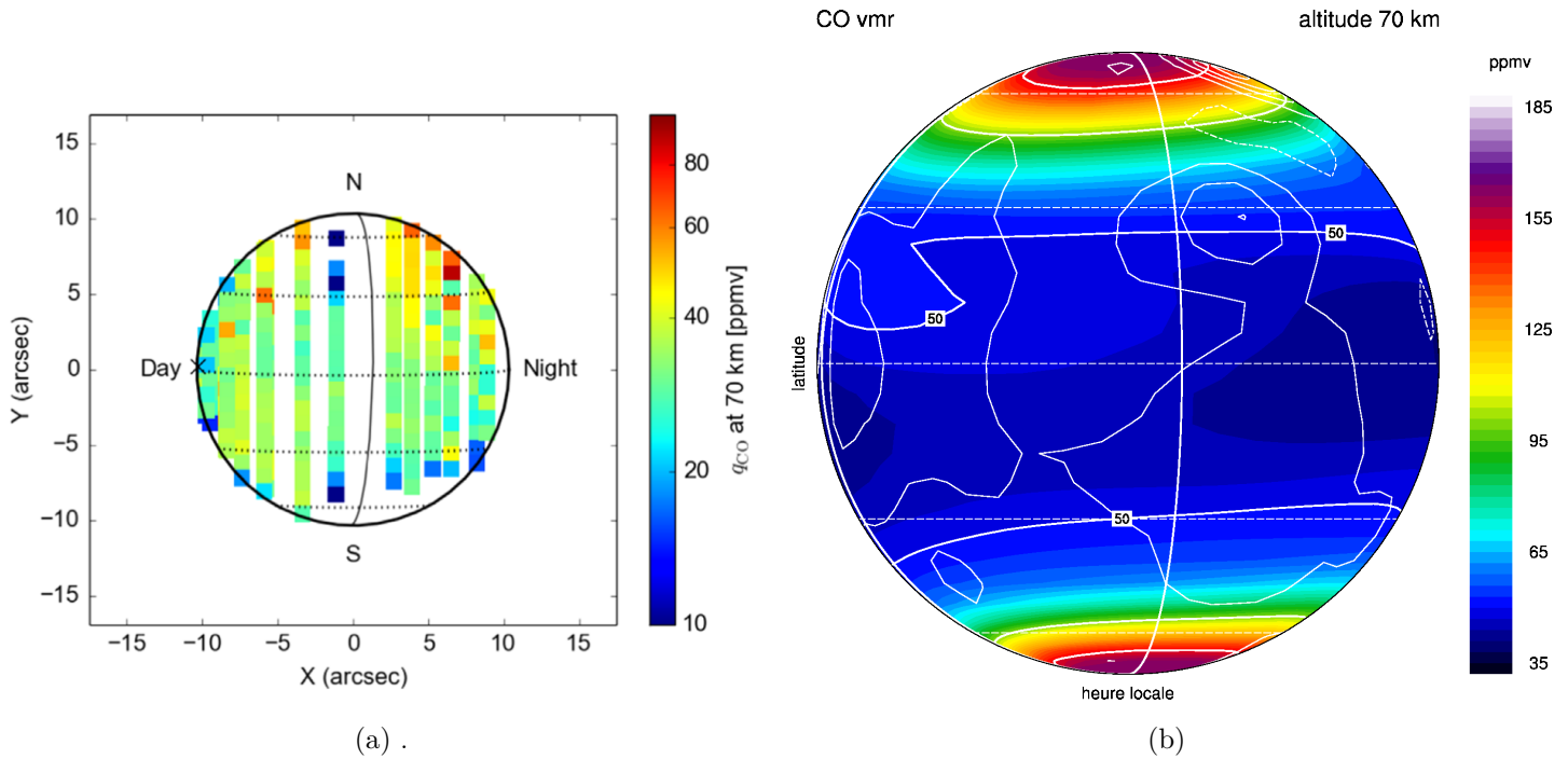
FIGURE 8.11 – Cartes en projection orthographique du rapport de mélange de CO à 70 km. La carte (a) provient des observations depuis la Terre avec le spectromètre CSHELL dans la bande 4,53 \mu\text{m} par Marcq et al. (2015) . La carte (b) est le rapport de mélange de CO calculé après 100j vénusiens simulés par notre modèle avec CO et SO 2 initialisés respectivement à 0 ppmv et 10 ppmv dans l'atmosphère profonde. Le terminateur est symbolisé par une ligne blanche pleine et est positionné afin de correspondre aux observations de la figure (a).
