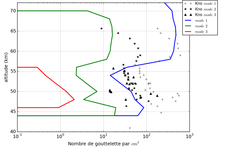
(d) Simulation initialisée avec 30 ppmv de \text{SO}_2
