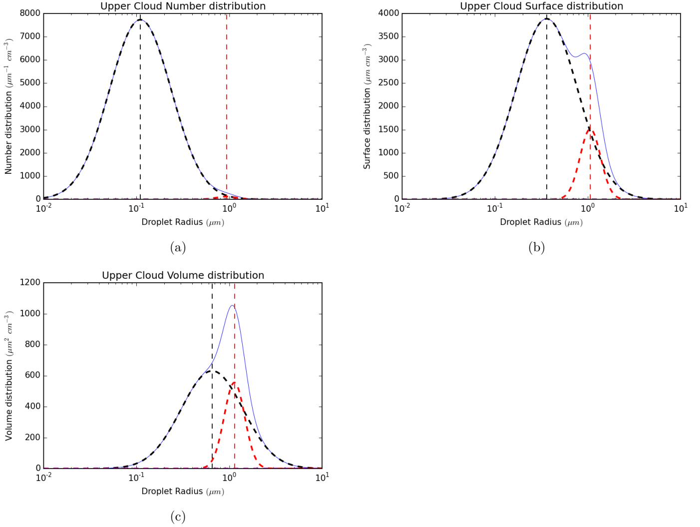
FIGURE 5.2 – Distribution de gouttelettes calculées pour les modes et la répartition en masse données par Knollenberg and Hunten (1980) pour le nuage supérieur ( \approx 60 km – 70 km d’altitude). Deux mode sont présents, le mode 1 et le mode 2 . Les distributions multi-modales en nombre (a), en surface (b) et en volume (c) affichent toutes les mode 1 (noir), mode 2 (rouge) et mode 3 (vert) en pointillés. Les pointillés verticaux montrent le rayon modal (le plus fréquent) de chaque mode. La courbe bleue représente la somme de tous les modes .
