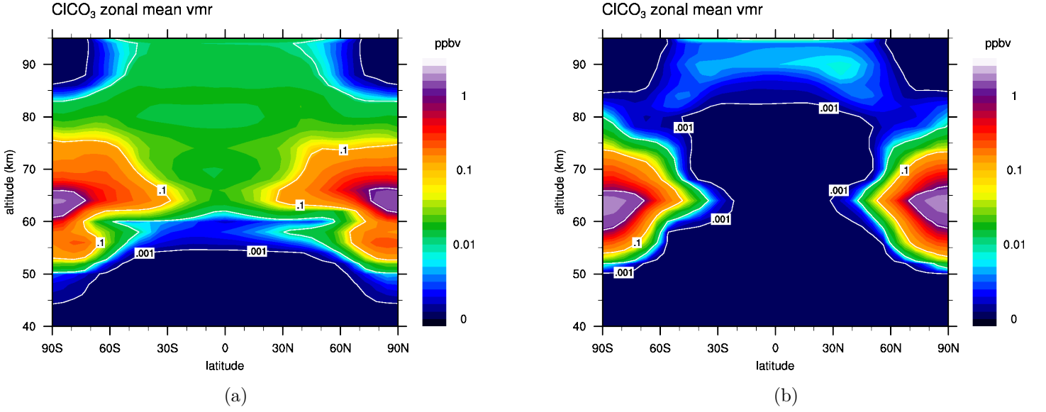
FIGURE 8.42 – Moyennes zonales de \text{ClCO}_3 selon différentes initialisations de l’atmosphère profonde en \text{SO}_2 après 100 jours vénusiens simulés. (a) simulation où \text{SO}_2 est initialisé à 10 ppmv et (b) à 15 ppmv.
