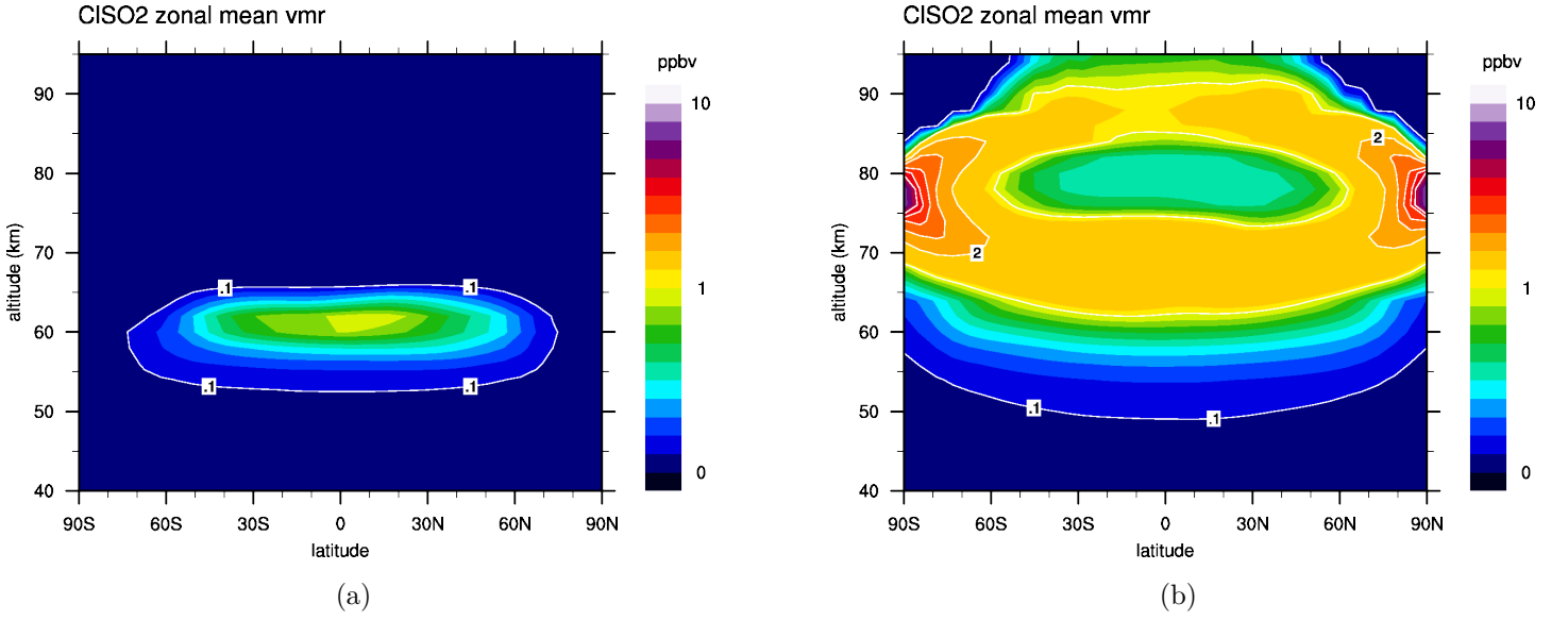
FIGURE 8.43 – Moyennes zonales de ClSO 2 selon différentes initialisations de l'atmosphère profonde en SO 2 après 100 jours vénusiens simulés. (a) simulation où SO 2 est initialisé à 10 ppmv et (b) à 15 ppmv.
