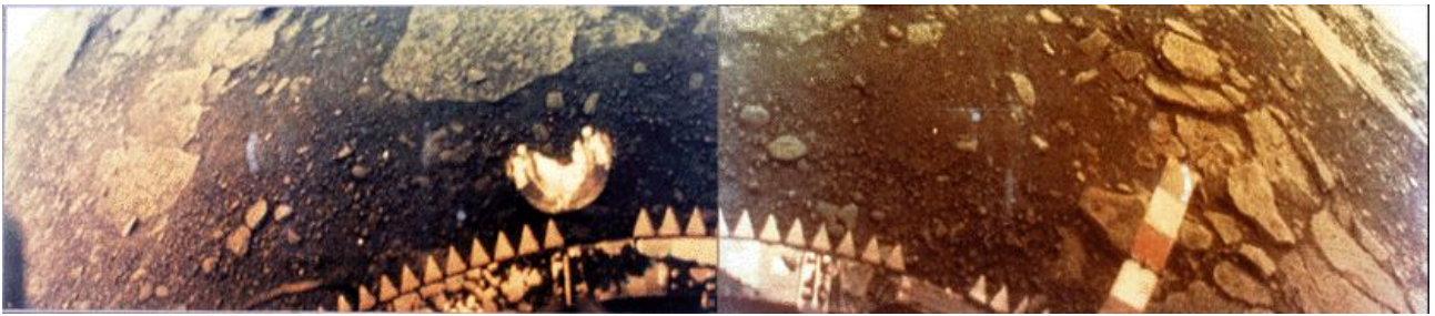
FIGURE 1.5 – Photo panoramique prise par la sonde Venera 13 à la surface de Vénus, mars 1982.
