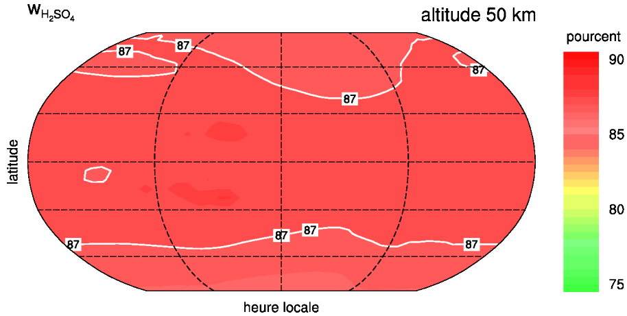
FIGURE 7.1 – Carte de la fraction d'acide sulfurique w_{H_2SO_4} dans les gouttelettes à 50 km. La simulation utilisée a été initialisée avec 10 ppmv en SO_2 dans l'atmosphère profonde. La carte est centrée sur le midi local.
