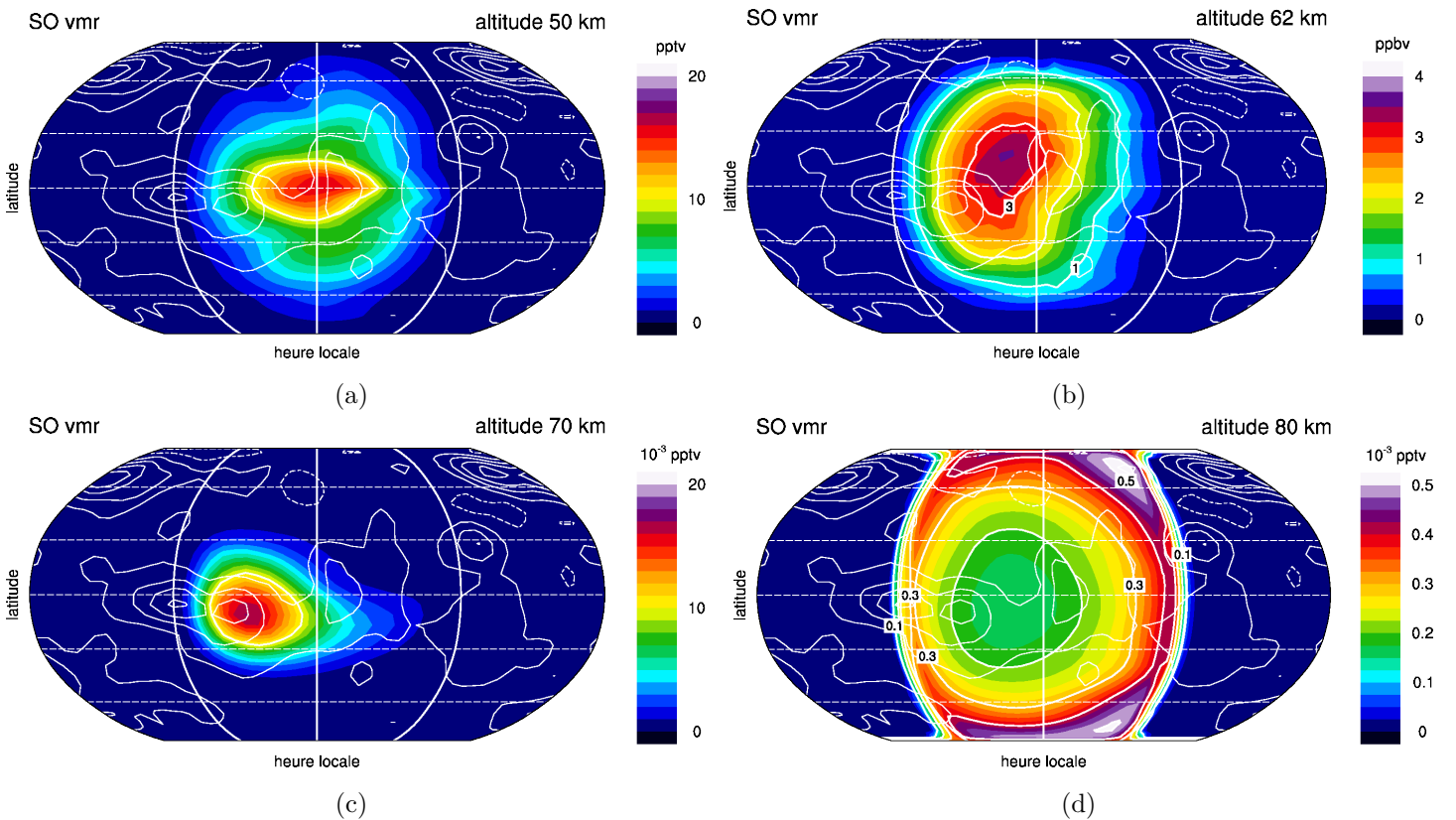
FIGURE 8.69 – Cartes de SO de 50 à 80 km. La simulation utilisée est initialisée à 10 ppmv de SO 2 dans l'atmosphère profonde. Les cartes sont centrées sur le midi local.
