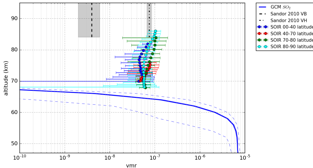
FIGURE 8.62 – Profils verticaux des moyennes zonales et pondérées en latitude du rapport de mélange de \text{SO}_2 . La simulation a été initialisée avec 10 ppmv de \text{SO}_2 dans l’atmosphère profonde. Les enveloppes colorées sont les écart-types pondérés sur la latitude de la moyenne zonale. Les mesures faites depuis la Terre de \text{SO}_2 dans le domaine sub-millimétrique, valeurs les plus hautes (VH) et basses (VB), de Sandor et al. (2010) sont affichées avec leur marge d’erreur. Les mesures de \text{SO}_2 dans l’infrarouge effectuées par SOIR à bord de Venus Express de Mahieux et al. (2015a) selon des tranches en latitude sont également reproduites avec leur marge d’erreur.
