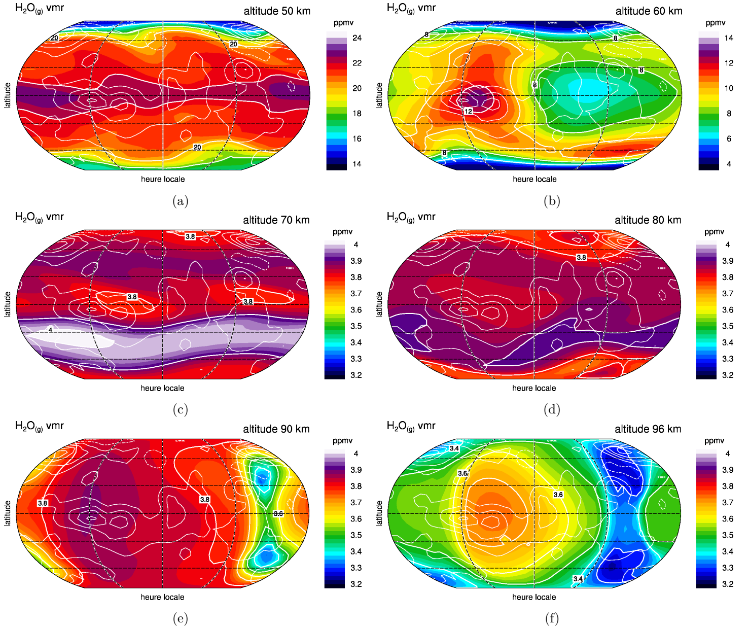
FIGURE 8.48 – Cartes de la vapeur d'eau H_2O_{(g)} de 50 à 96 km. La simulation est initialisée à 10 ppmv de SO_2 dans l'atmosphère profonde. Les cartes sont centrées sur le midi local.
