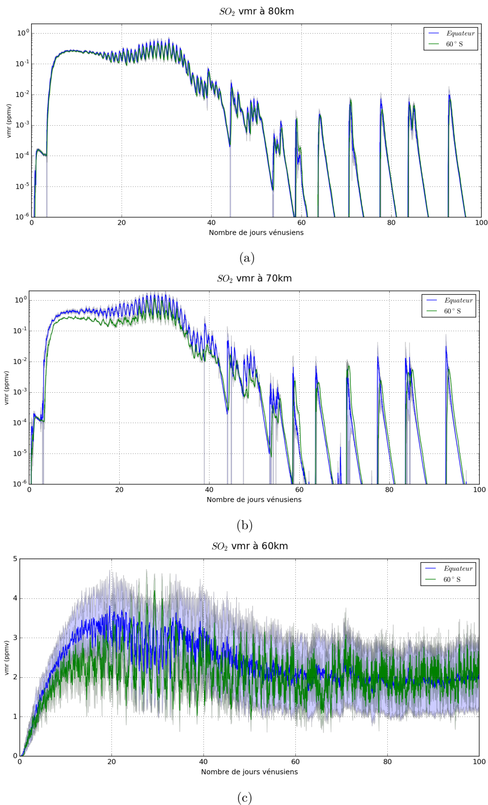
FIGURE 8.64 – Série temporelle du rapport de mélange de SO_2 à l'équateur et 60^\circ S à (a) 80 km, (b) 70 km et (c) 60 km. Les enveloppes de couleurs claires représentent la déviation standard en longitude du rapport de mélange de SO_2 .
