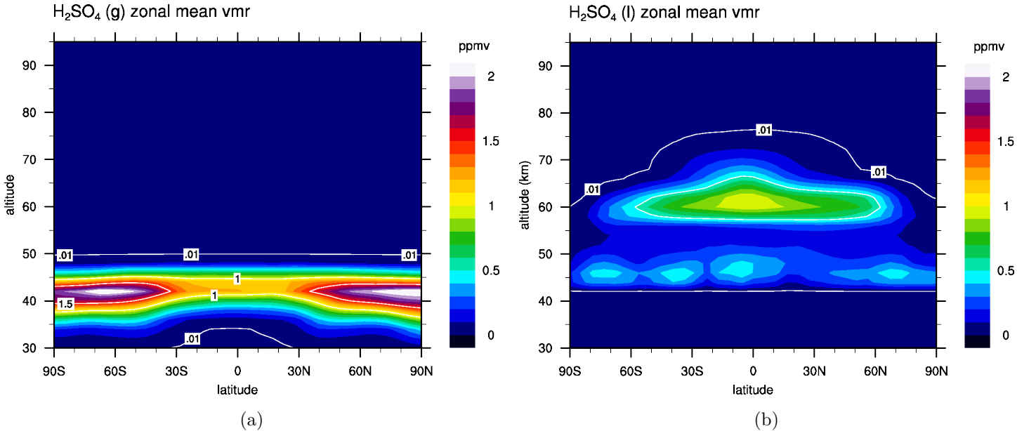
FIGURE 8.73 – Moyennes zonales de la vapeur d'acide sulfurique \text{H}_2\text{SO}_{4(g)} et de sa partie condensée \text{H}_2\text{SO}_{4(l)} avec \text{SO}_2 initialisé à 10 ppmv dans l'atmosphère profonde.
