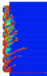
Figure 67. Distribution d'endommagement obtenue par simulation fine de l'essai de pull-out (Lu, 2013)
