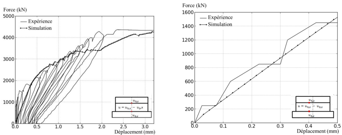
Figure 43. Evolution de la force en fonction du déplacement relatif. Comparaison entre la simulation utilisant le modèle de liaison acier-béton et l'expérience avec le capteur de déplacement (gauche) et entre la simulation et l'expérience obtenue par corrélation d'image (droite) (Mang et al, 2016)
