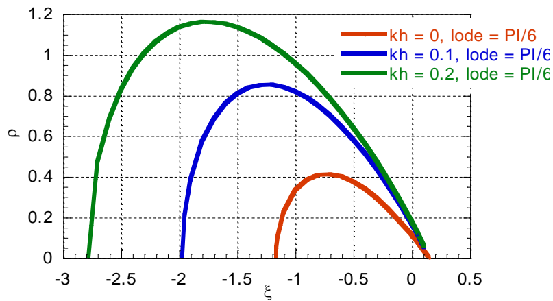
Figure 10. Surface seuil du modèle de plasticité. Evolution avec le paramètre d'érouissage « kh ». Représentation dans le repère des invariants de contrainte normalisés.
