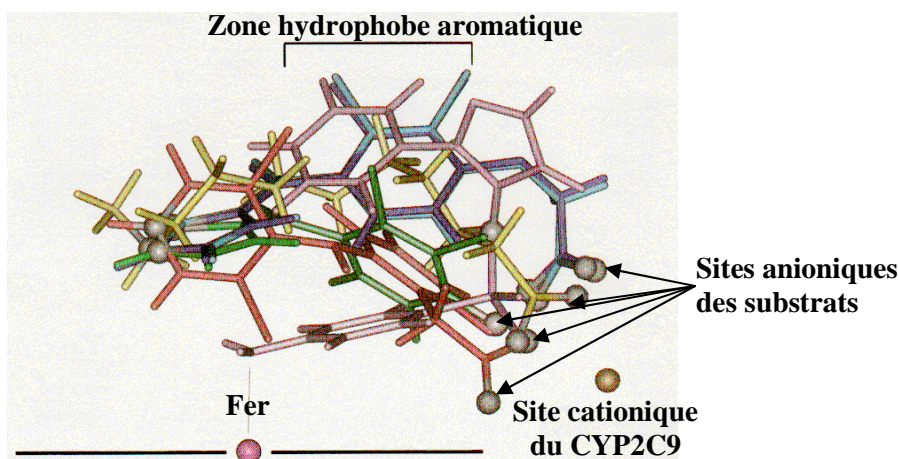
Figure 27 : Superposition de six ligands du CYP2C9 (Acide tiénilique et deux dérivés, diclofénac, acide laurique, sulfaphénazole) d'après (Poli-Scaife et al., 1997).
