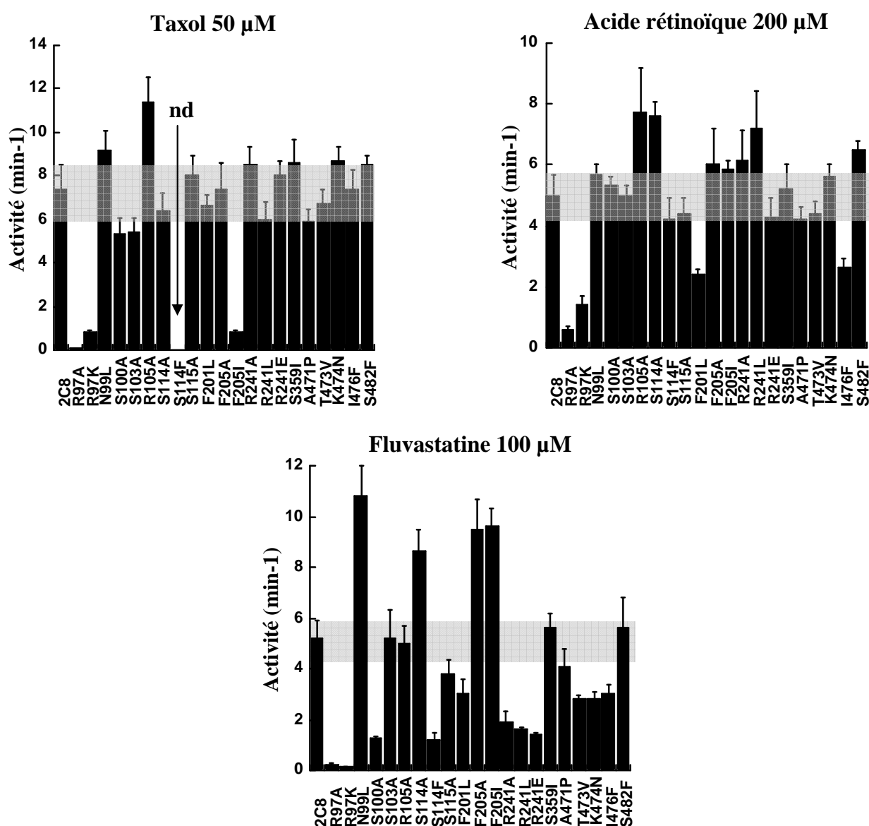
Figure 57 : Activités d'hydroxylation du taxol 50 µM, de l'acide rétinolique 200 µM, et de la fluvastatine 100 µM par le CYP2C8 et ses mutants (moyenne ± l'écart type sur trois mesures). La zone grisée permet de visualiser les valeurs non significativement différentes de celles du CYP2C8; nd = métabolite non détecté.
