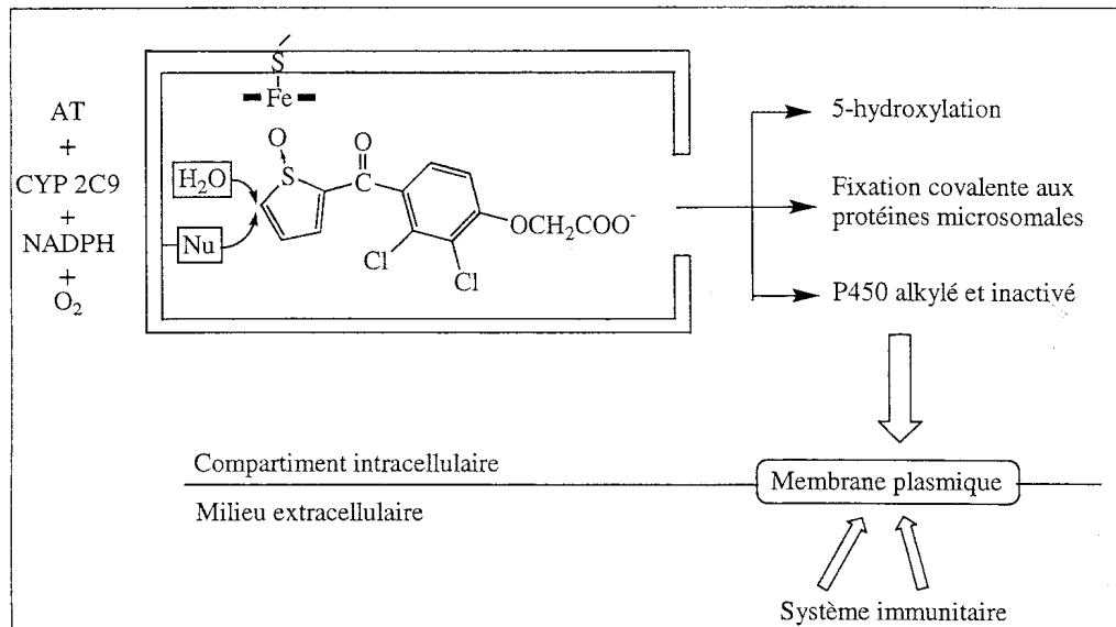
Figure 22 : Mécanisme proposé pour le métabolisme de l'acide tiénilique (AT), l'inactivation suicide du CYP2C9 et le début du phénomène hépatotoxique (d'après Lopez-Garcia et al., 1994 et Beaune et al., 1994).
