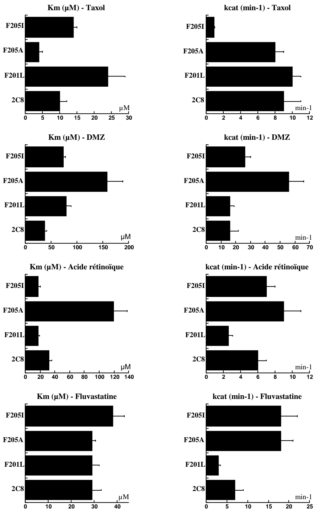
Figure 62 : Histogrammes permettant de visualiser les différences de Km et kcat entre le CYP2C8 et ses mutants en positions 201 et 205 pour 4 substrats : taxol, DMZ, acide rétinoïque et fluvastatine (données des tableaux 33 et 34).
