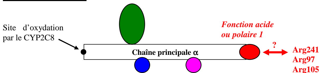
Figure 59 : Représentation schématique des interactions potentielles entre les fonctions acides ou polaires terminales des substrats et trois arginines du CYP2C8.
