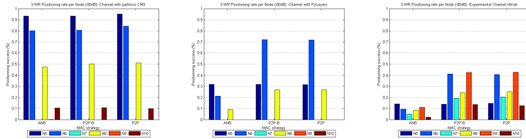
(a) P_{succ} avec le canal empirique (b) P_{succ} avec le canal simulé (c) P_{succ} avec le canal exp.
