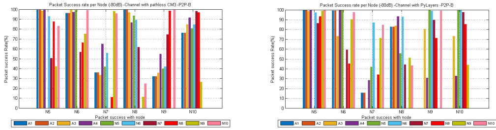
(a) Taux de réception de paquet avec le canal em- (b) Taux de réception de paquet avec le canal sim- piriqueulé
