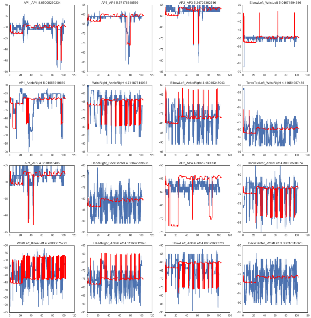
FIGURE 3.9 – Comparaison du RSSI (bleue) et la quantité d_{sh} (rouge) centrée pour les liens ayant le facteur de corrélation le plus grand.
