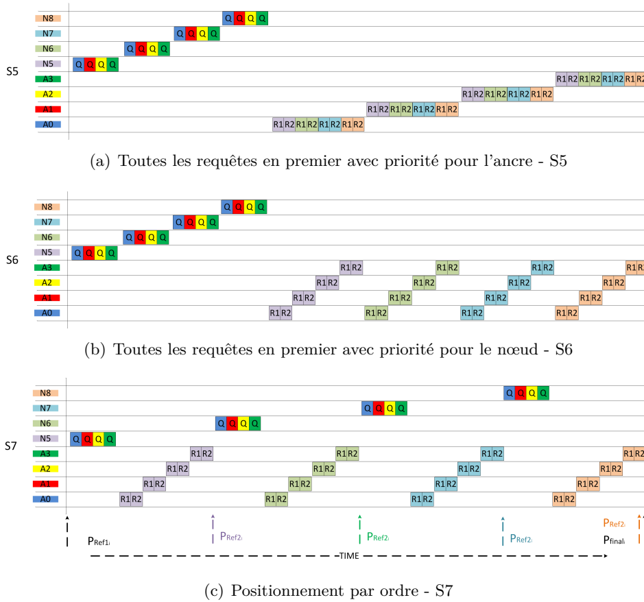
FIGURE 5.5 – Stratégies d'ordonnement pour quatre nœuds et quatre ancres. Dans ce schéma, chaque nœud a une couleur. Ainsi, la couleur de chaque paquet représente le nœud de destination.
