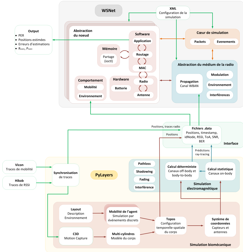
FIGURE 3.12 – Architecture du co-simulateur avec WSNNet et PyLayers.
