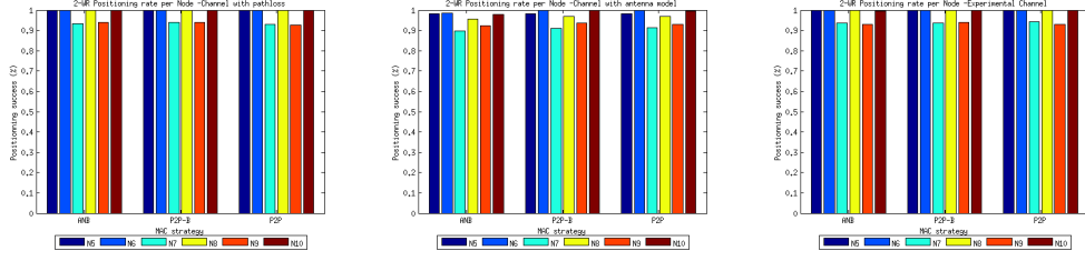
(a) P_{succ} avec le canal empirique (CM3) (b) P_{succ} avec le canal simulé (Pylayers) (c) P_{succ} avec le canal expérimental (HiKob)
