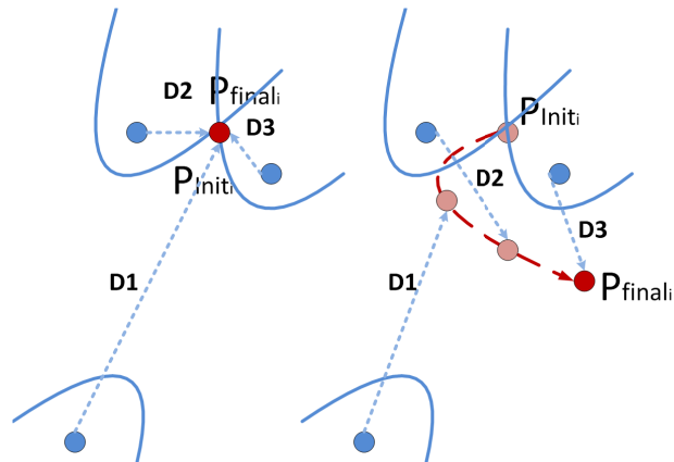
FIGURE 2.4 – Erreur sur l'estimation de la distance avec TDOA entre un nœud statique et un nœud mobile
