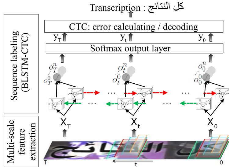
FIGURE 2: Schéma général de reconnaissance proposé.
