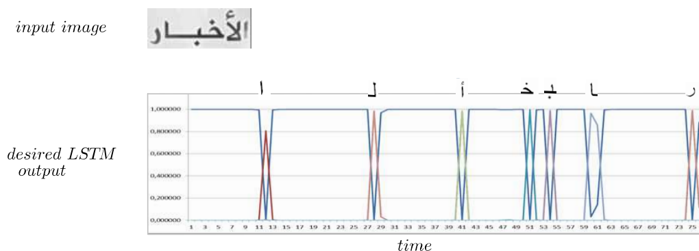
FIGURE 5: Les activations cibles en sortie du BLSTM à travers le temps. Chaque courbe correspond à l'évolution de la réponse du BLSTM pour une classe bien particulière (caractère ou BLANK). Le BLSTM donne, le plus souvent, un BLANK en sortie correspondant à la courbe bleu foncé.
