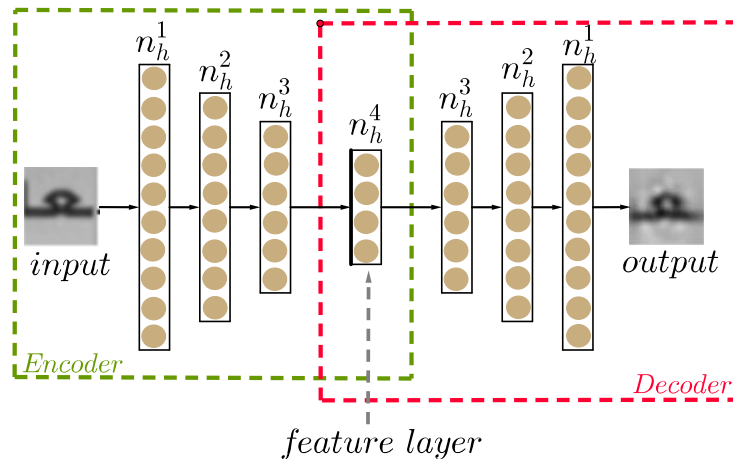
FIGURE 4: Auto-Encodage caractères basé sur le DBN.
