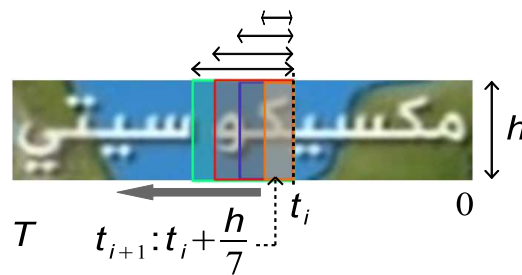
FIGURE 3: Procédure de scanning.
