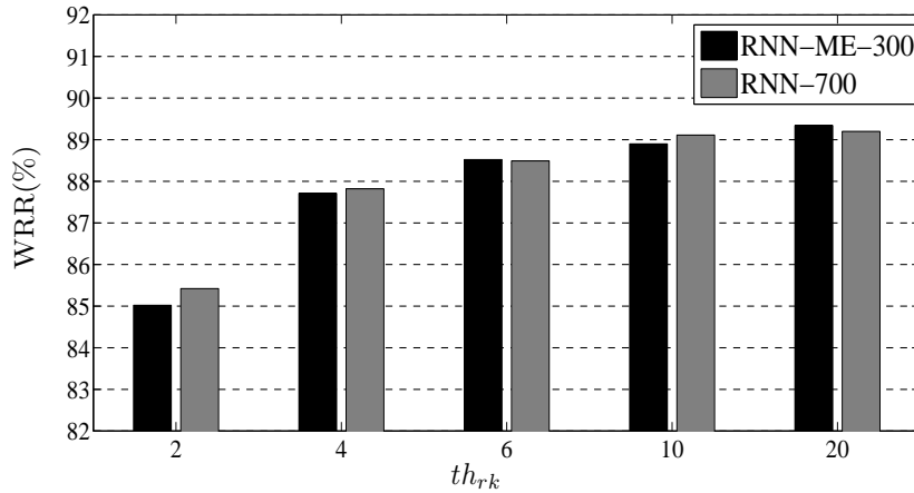
(a) WRR.
