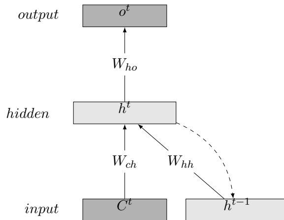
FIGURE 6: Modèle de langage à base de RNN.
