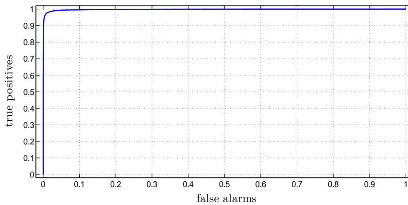
(b) HAARada.
