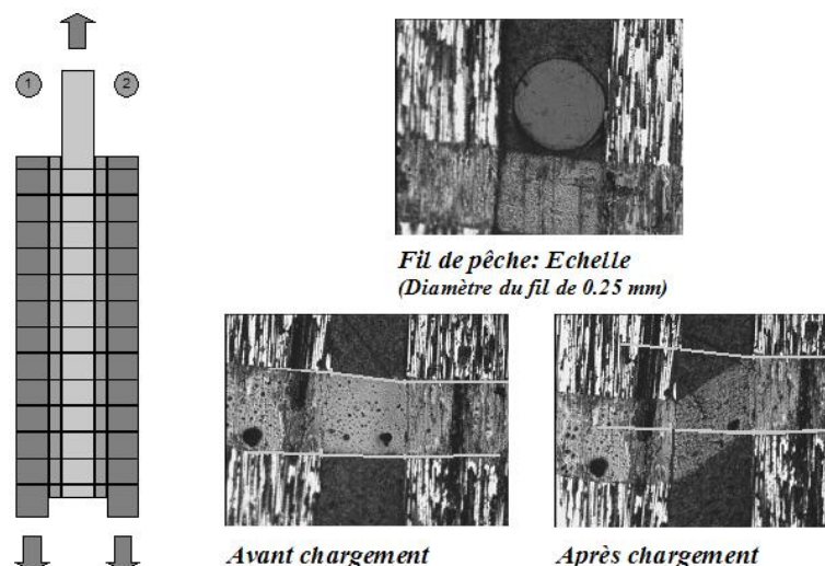
FIGURE 2.6: Schema du joint testé dans et exemple de photos de la déformation locale en cisaillement de la couche de résine obtenue avant et après un cycle de charge-décharge
