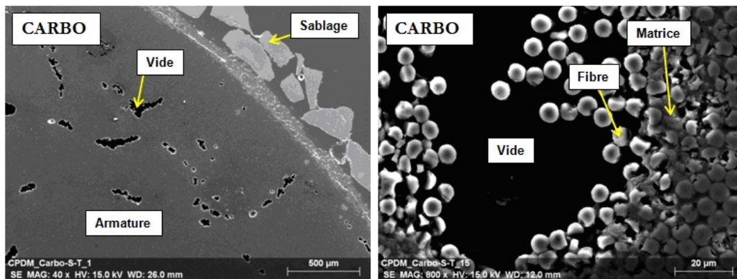
FIGURE 6.3: Observations au microscope électronique à balayage d'une section d'armature composite à fibre de carbone à deux grossissements différents Rolland (2015)
