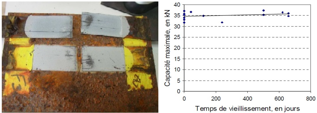
FIGURE 4.4: Photo des modes de rupture observés et évolution de la capacité de l'assemblage en cisaillement au cours du vieillissement en milieu humide Chataigner et al. (2011d)
