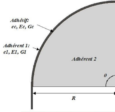
FIGURE 2.12: Schéma du joint courbe étudié
