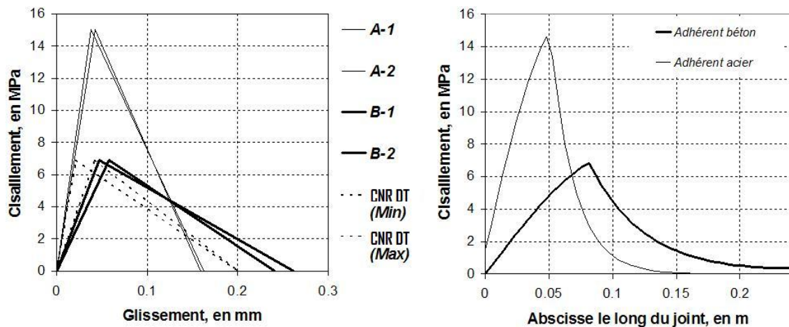
FIGURE 4.3: Détermination du modèle biblinnaire de zone cohésive pour le collage sur adhérent béton et acier, et profils de cisaillement ultime associés Chataigner et al. (2011a)
