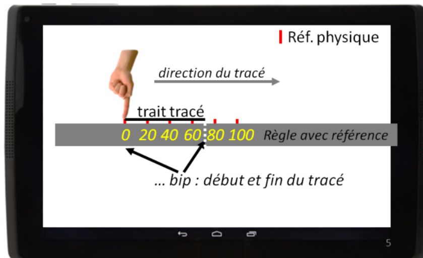
Figure 4-12 : illustration de la technique « Règle graduée ». Exemple d'utilisation : « je fais une double tape, j'entends un bip, je déplace doucement mon doigt vers la droite en passant sur les clous (réf. physiques). Lors de mon déplacement, j'entends un bip, j'estime la valeur transmise, m'aidant des références sur la règle».
