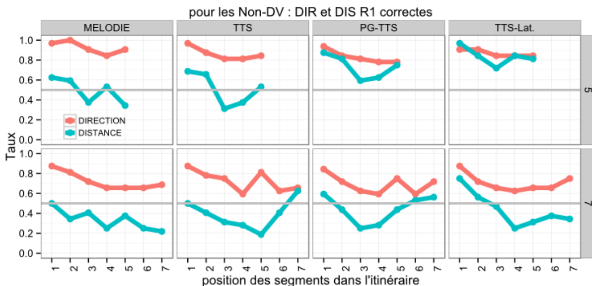
Figure 5-18 : Moyenne des items correctement restitués (R1) par les Non-DV, selon la position du segment dans l'itinéraire. Les graphiques illustrent les directions (rouge) et les distances (bleu) par technique et par taille d'itinéraire (5 en haut et 7 en bas). Seule TTS-Lat, pour la taille 5, résiste à l'effet de position. Rappelons que Mélodie est la seule technique utilisant le codage DURÉE pour la distance, les autres techniques utilisent la parole.
