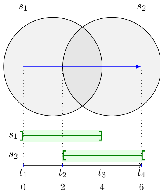
(a) Exemple avec 2 capteurs
