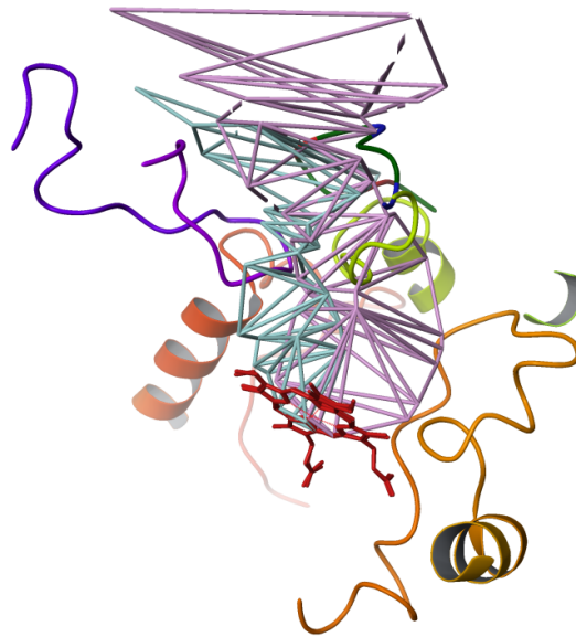
Figure 3.20 : Trajets S pour le CYP3A4 en forme apo (code 1TQN) et holo (code 4K9U). Pour le 1TQN, le trajet S, en bleu, est ouvert à CV=5\text{\AA} (petit site actif sous la boucle FF'). Pour le 4K9U, le trajet S, en violet, est ouvert à CV_{lim}=6.75\text{\AA} ; le trajet S et le site actif sont élargis par le mouvement de la boucle FF, et bordés par les structures secondaires de la forme apo; la boucle FF' de la forme holo est en couleurs foncées, suivant les propriétés physico-chimiques des acides aminés.
