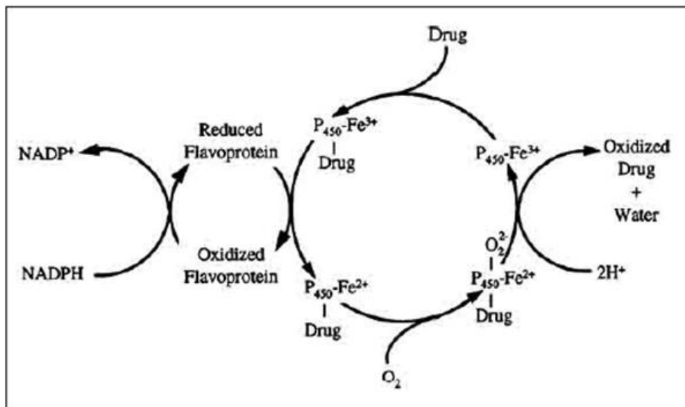
Figure 3.9 : Cycle catalytique du cytochrome P450. Image du haut extraite de http://enzymology.lab.ls.manchester.ac.uk/labgroups/leysgroups/ le 24/11/2014. Image du bas : figure 1, [Kalra 2007].
