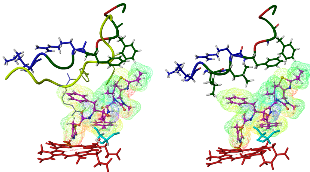
Figure 3.24 : Maillage de la surface de van der Waals du ritonavir ( 777\text{\AA}^2 ). Les sphères sont colorées suivant le potentiel électrostatique. Le ritonavir est en boules-bâtons, en magenta. La boucle FF' et les acides aminés du complexe 3NXU sont coloriés suivant leurs propriétés physico-chimiques. A gauche : superposition de la boucle FF' (en vert clair) des acides aminés R212, F213 et F215 (en tubes minces) de 1TQN (forme C). En pointillés noirs, la liaison H entre R212 et K208.
