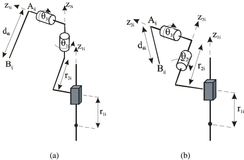
Figure 5.4 : Placement des repères des jambes : (a), i=1,2 et (b), i=3..6
