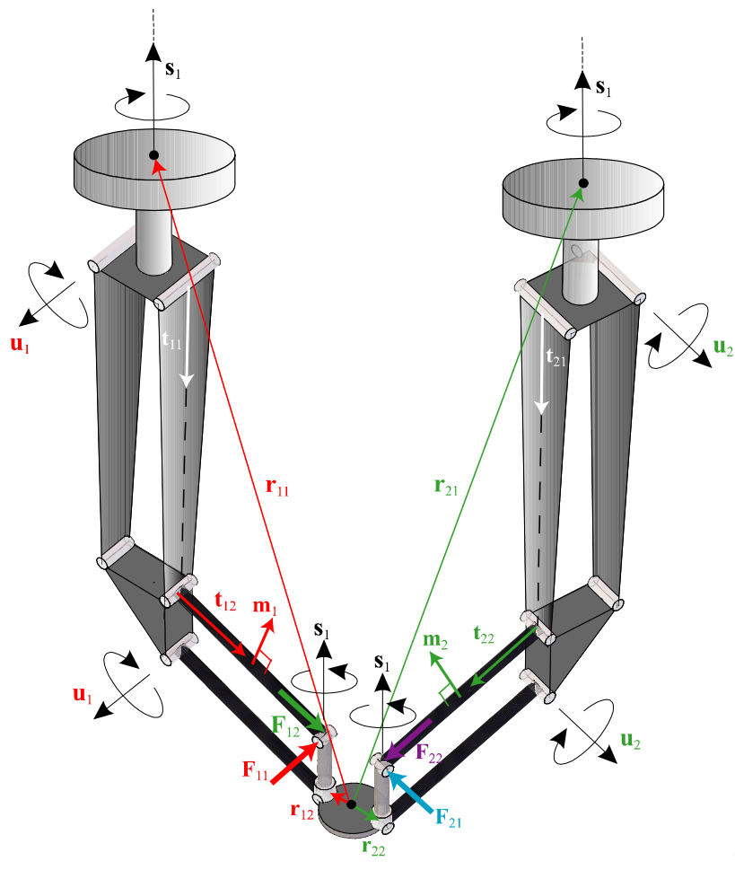
Figure 4.7 : vue de face(a) et représentation CAO (b) du McGill Schönflies-Mouvement Générateur (SMG)
