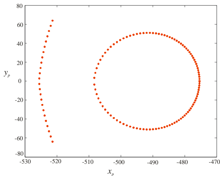
Figure E.1 : Courbes des singularités dans l'espace opérationnel
