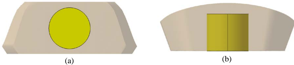
Figure 3.20 : Comparaison entre l'espace de travail 3-axes calculé par notre méthode ( L_{ul} = 50mm ) et celui fourni par Fatronik, (a) vue de dessus et (b) vue de gauche
