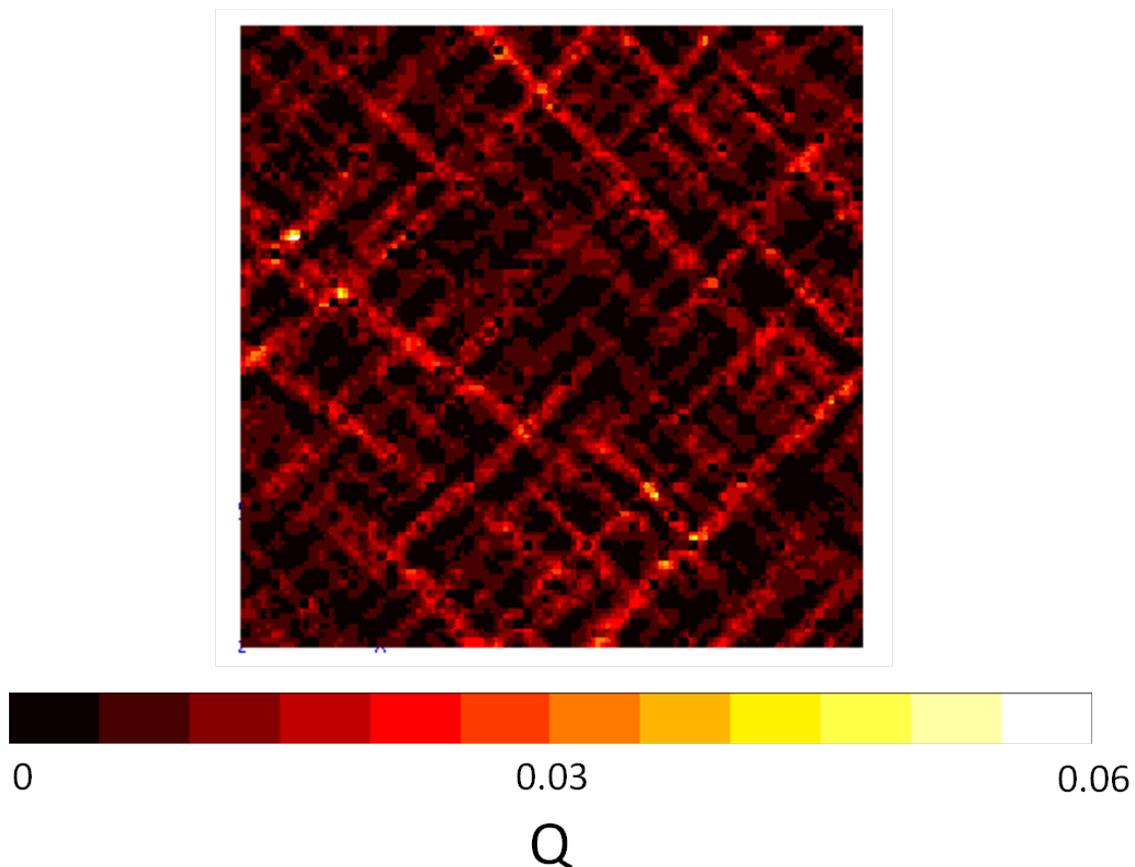
Figure 20 : Localisation de la dissipation d'énergie à la fin de la charge pour \log(\dot{\varepsilon}) = 3 . La localisation de la dissipation se fait sur les bandes de cisaillement à 45^\circ des axes propres du tenseur de déformation comme observé expérimentalement à plus grande échelle.
