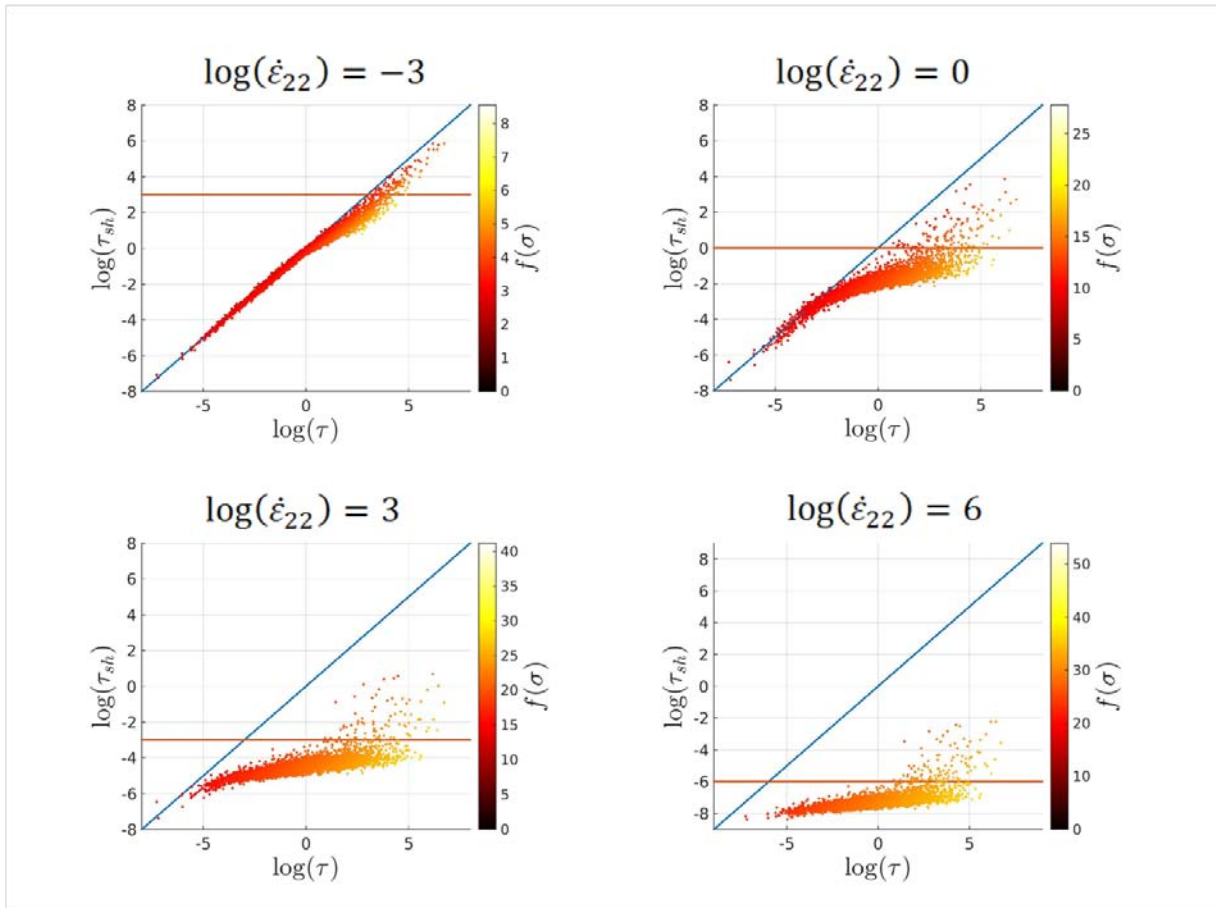
Figure 28 : Corrélation entre \tau_{sh} et \tau_i en fin de charge à \log(\dot{\epsilon}_{22}) = -3, 0 et 3 . Données correspondant à une déformation \square = 0.1
