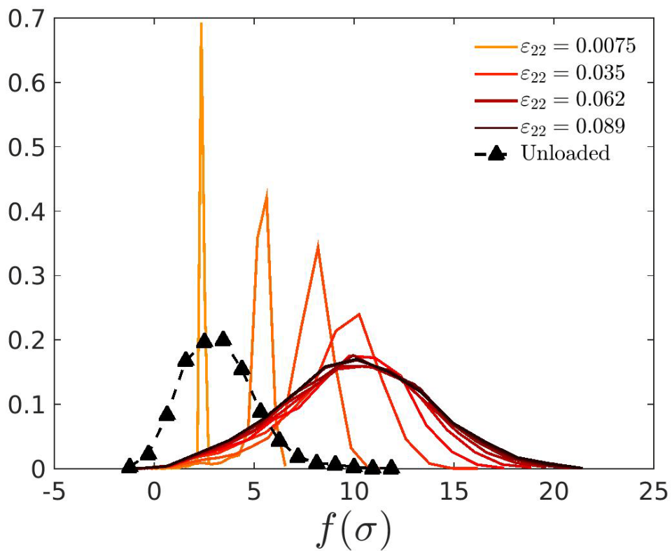
Figure 25 : Distribution de f(\sigma) au cours de la charge et après décharge. Cette distribution tend vers une Gaussienne e dont l'écart-type est égal à \Sigma\sigma\ln(10) = 4.6 \cdot 10^{-2} avec une précision de l'ordre de 0.02 et centré sur \langle f(\sigma) \rangle_{yield} .
