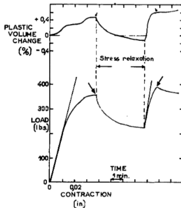
Figure 40 : Courbe de changement de volume et courbe de la contrainte en fonction de la déformation au cours d'une charge interrompu et reprise. 20
