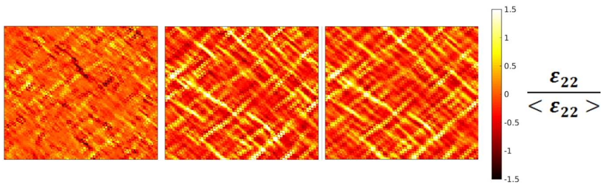
Figure 17 : Effet de la vitesse sur la différence de localisation de déformation. Des cartes de \frac{(\epsilon_{22,NL} - \epsilon_{22,lin})}{\epsilon_{22,macro}} sont tracées à \epsilon_{22,macro} = 0.1 pour les vitesses de déformation suivantes : \log(\dot{\epsilon}_{22}) = -3, 0 et 3 .
