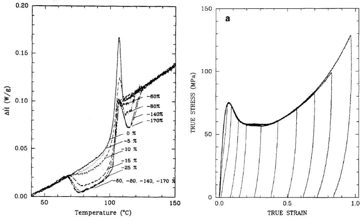
Figure 11: Courbes de flux de chaleur mesurées à 10K/min sur des échantillons de polystyrène vieilli puis ayant subi une déformation en compression allant de -5% à -170% (à 0.001 s -1 à T=T g -80K). Les déformations comprises entre 60% et 170% correspondent au régime de strain-hardening (figure de droite).
