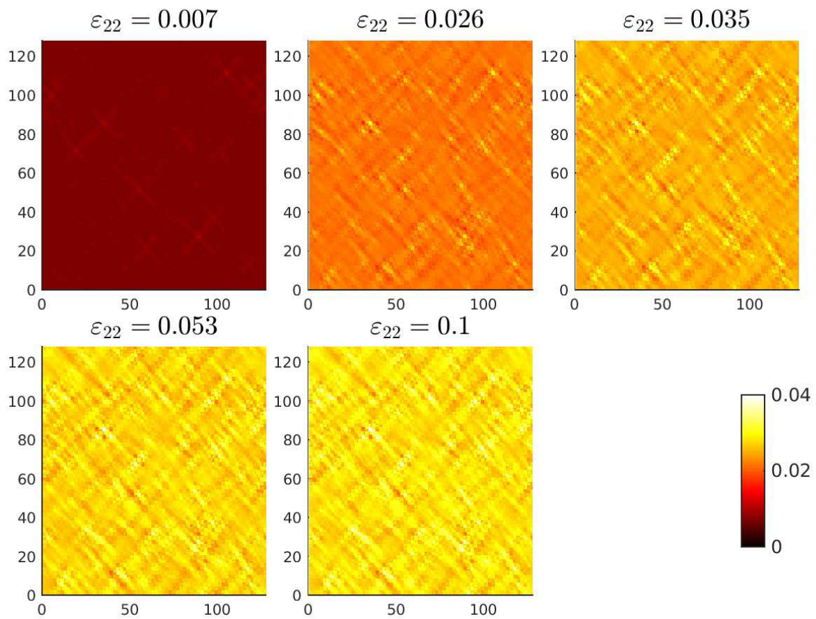
Figure 32 : Carte de la différence de déformation \varepsilon_{22} entre avant la décharge et après celle-ci. La différence de déformation est relativement homogène.
