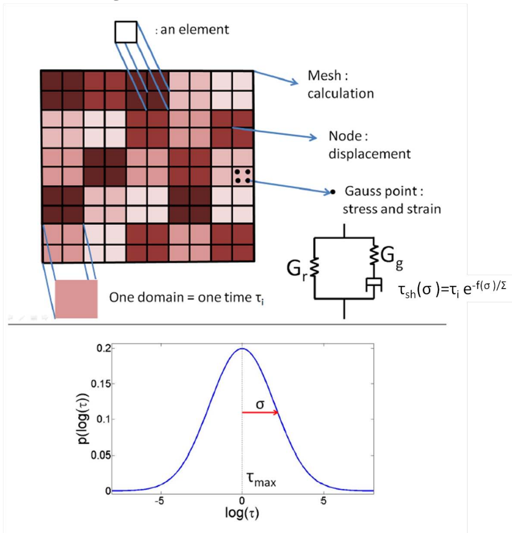
Figure 1 : Présentation du modèle. Le modèle utilisé dans ce chapitre est le même qu'au chapitre 2 mis à part que le temps de relaxation \tau_{sh} de l'élément de Maxwell est modifié par la contrainte locale. \tau_i est distribué aléatoirement sur les domaines selon une distribution log-normale d'écart-type \sigma .
