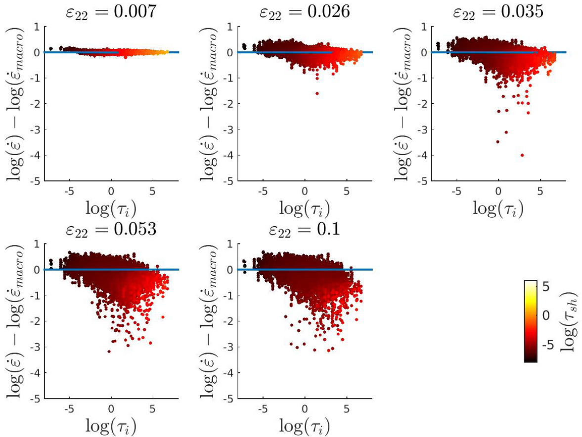
Figure 19 : Corrélation entre \log(\dot{\varepsilon}_{22}/\dot{\varepsilon}_{22,macro}) et \log(\tau_i) pour \log(\varepsilon_{22})=3 . Le trait horizontal bleu représente le taux de déformation macroscopique. On observe une augmentation du désordre en taux de déformation au sein du système. \varepsilon = 0.007 correspond au régime élastique. \varepsilon = 0.007, 0.035 et 0.053 correspondent respectivement à des points juste avant le seuil, au seuil et au début du plateau. \varepsilon = 0.1 correspond au plateau en contrainte bien établi. (cf. Figure 6)
