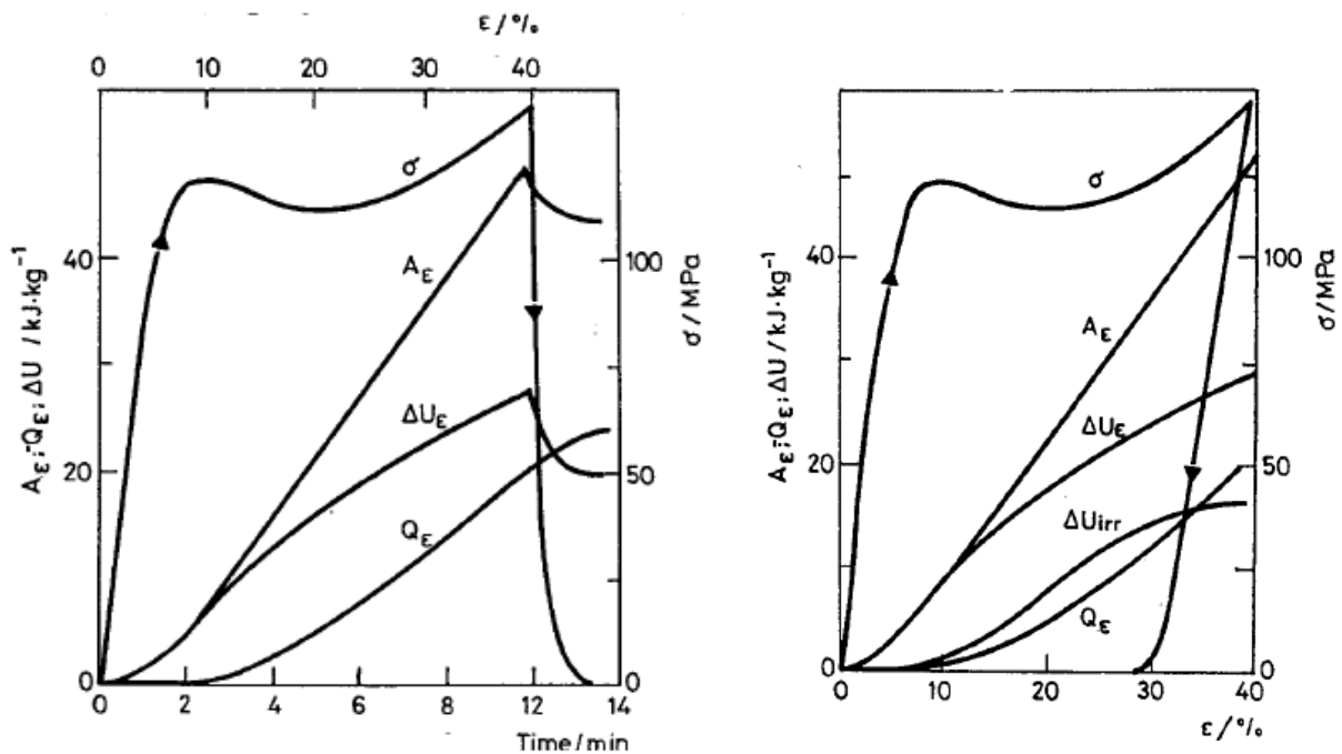
Figure 8 : Evolution de A_\epsilon , Q_\epsilon , \sigma , \Delta U_\epsilon en fonction du temps ( à droite) et en fonction de la déformation ( figure de gauche) pour du EAN (epoxy-aromatic amine network). \frac{d\epsilon}{dt} = 3.10^{-2}min^{-1} et T=298K . Mesures réalisées en imposant un test en compression uniaxiale. T_g=417K à 1Hz
