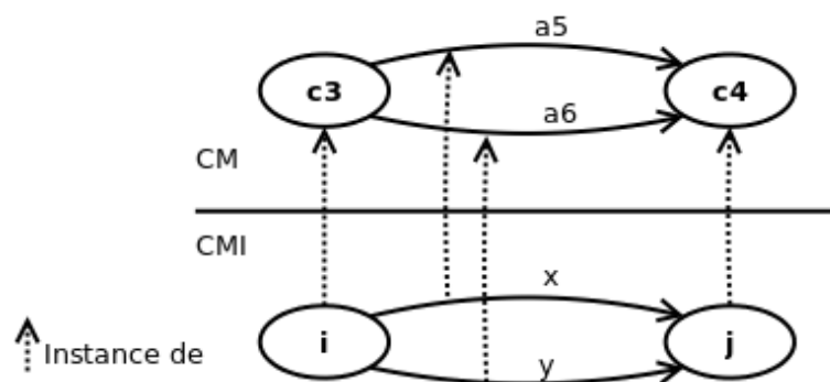
FIGURE 5.13 : Exemple de CMI satisfaisant la contrainte \psi_c(C, c_3)
