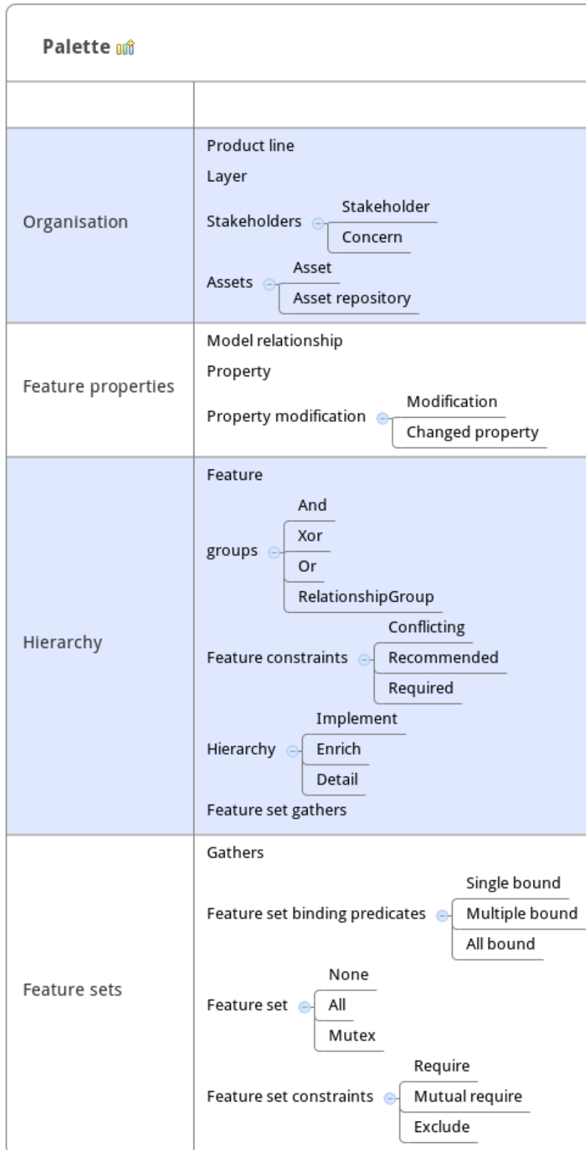
FIGURE 4.21 : Organisation de l'ensemble des éléments de la palette
