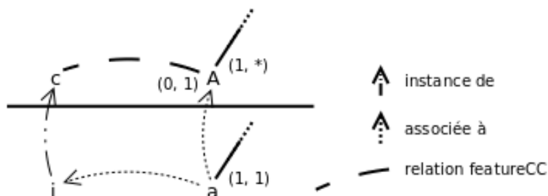
FIGURE 5.17 : Exemple d'intersection entre les intervalles des multiplicités de la caractéristique A et de la fonction featureCC reliant A au concept c dont i est l'instance.
