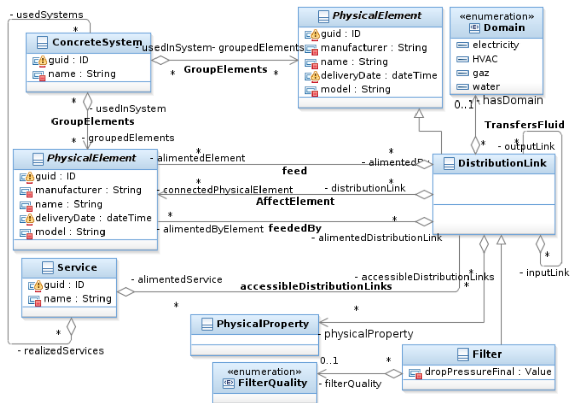
FIGURE 2.8 : Éléments permettant la distribution d'énergie dans un bâtiment
