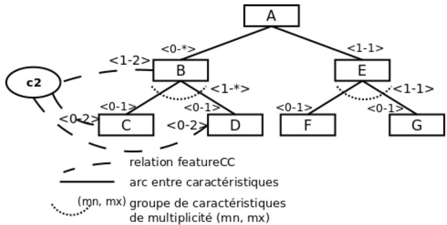
FIGURE 5.11 : Modèle générique de caractéristiques utilisant le formalisme des modèles de caractéristiques avec multiplicité [Czarnecki et al. , 2004b] étendu par la liaison avec les concepts du domaine (ici c_2 ).
