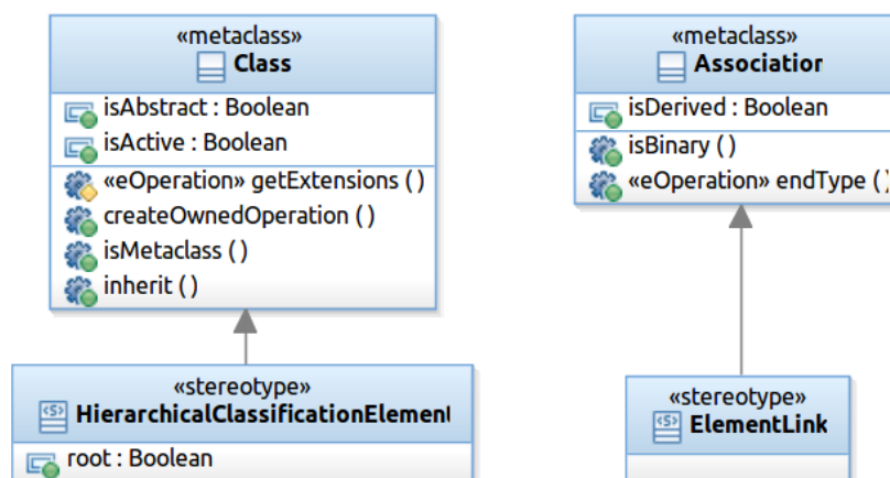
FIGURE 4.18 : Profil UML décrivant la navigabilité entre les classes du contexte
