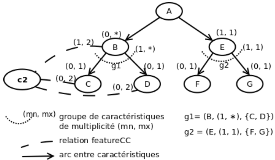
FIGURE 5.10 : Modèle générique de caractéristiques représenté sous la forme d'un graphe orienté
