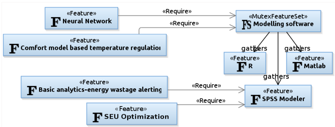
FIGURE 6.10 : Contraintes de sélection entre les caractéristiques d'optimisation et les composants logiciels
