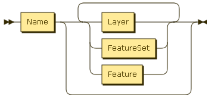
FIGURE A.12 : Layer
