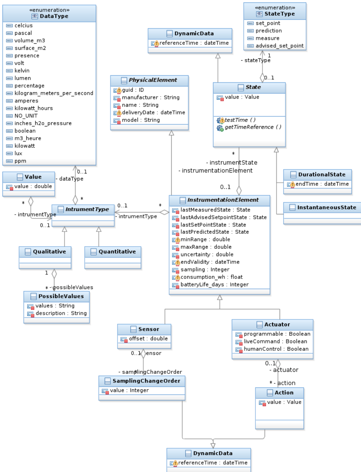
FIGURE 2.7 : Instruments permettant la supervision d'un bâtiment
