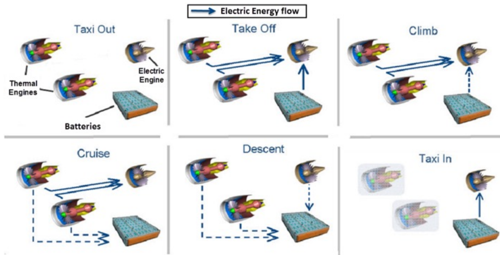
Figure 7.4: Stratégie de gestion des flux d'énergie. Les flèches bleues indiquent les flux d'énergie électrique.
