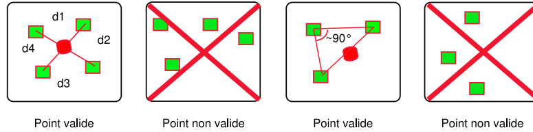
FIG. 3.13 – Test de l'algorithme des carrés.
