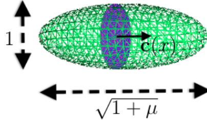
FIGURE 4.3.1 – Boule unité associée à \phi
