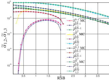
Figure 7.10: Comparaison entre les tests \delta^{0-1}(X) et \delta^Q(X) en ce qui concerne \tilde{\alpha}_{1,2} et \tilde{\alpha}_{1,3} comme les fonctions de RSB.
