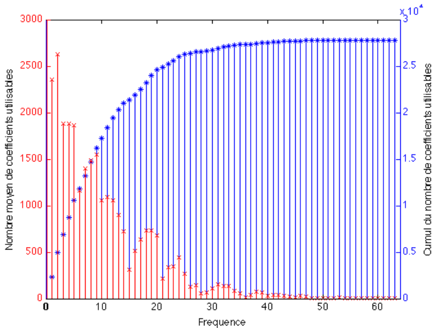
FIGURE 5.11 – Nombre moyen de coefficients utilisables des coefficients DCT AC par fréquence (x) et cumul (*) sur la base BOSS compressée avec facteur de qualité 50.
