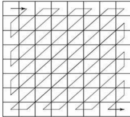
FIGURE A.1 – Mise en ordre zigzag.
