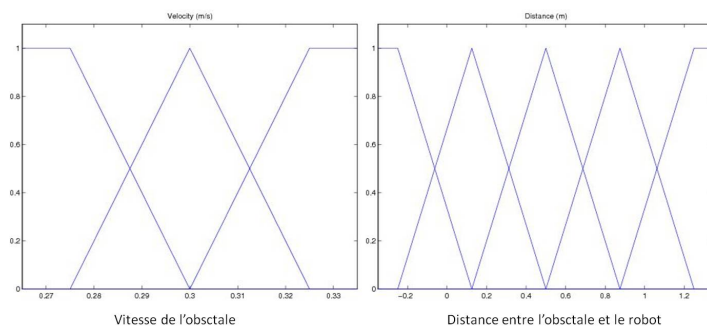
FIGURE 4.4.4: Fonctions d'appartenance utilisées pour la vitesse de l'obstacle ( v_{obs} \in [0..0, 3] ) et la distance entre le robot et l'obstacle ( d_{obs} \in [1..1, 2] ).
