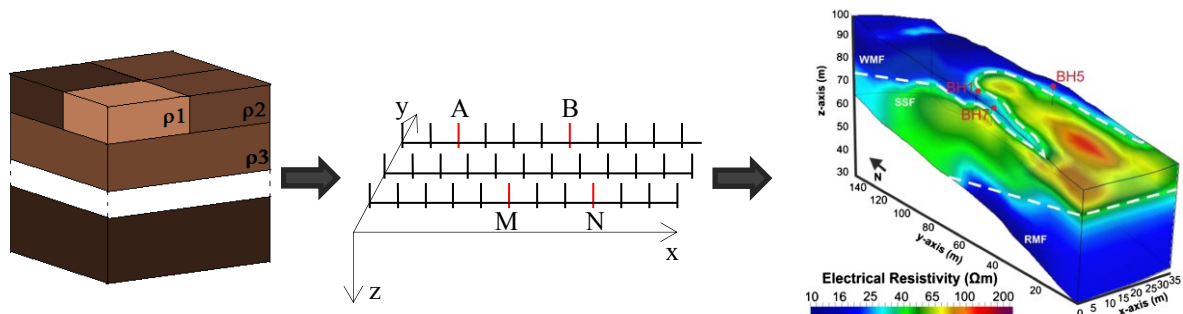
Figure 10. Représentation schématique de la méthode d'imagerie électrique 3D avec la mise en place d'une grille d'électrodes. Des mesures inter-lignes permettent d'obtenir un résultat d'inversion 3D. [ Merritt et al. , 2014]
