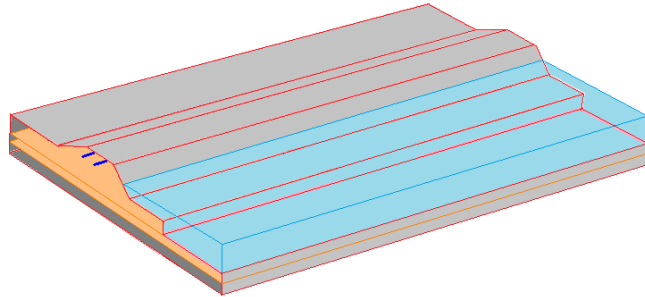
Figure 53. Schéma du modèle 3D représentant le tronçon de digue du val d'Authion avec l'emplacement des lignes d'électrodes (lignes bleues) sous la crête de digue. Les interfaces lithologiques sont représentées par des plans oranges et la Loire par un volume bleu clair.
