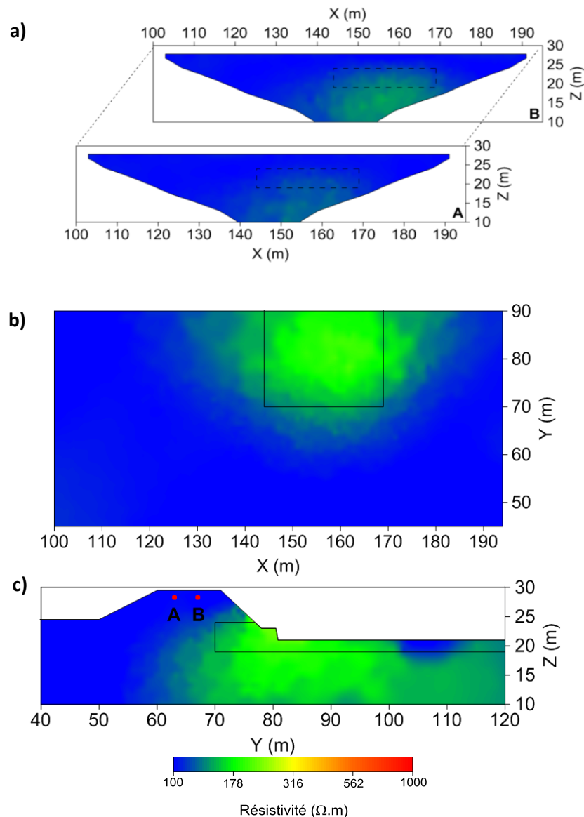
Figure 60. Coupes d'inversion 3D - de la levée en présence d'un corps résistif après 5 itérations (erreur RMS de 1.69%) : a) sections longitudinales de A- la ligne côté val (Y=63m) et B- la ligne côté Loire (Y=67m), b) vue aérienne de la levée à une altitude de Z=20m et c) une vue transversale de la levée à X=157m. Les lignes pointillées et continues marquent l'emplacement de la structure anormale résistive.
