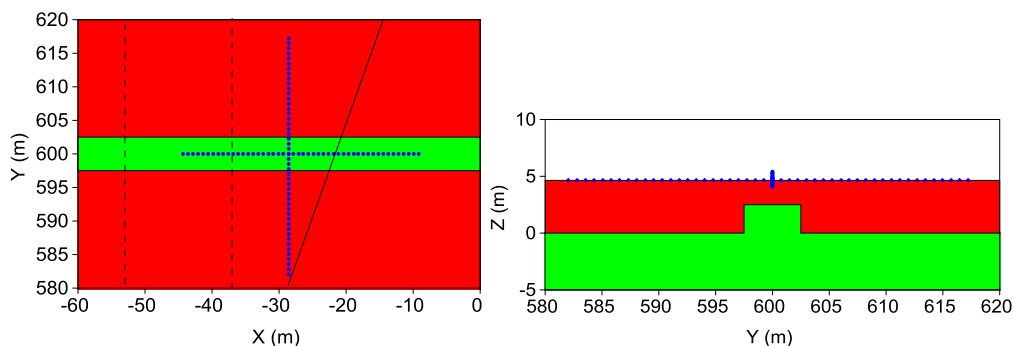
Figure 106. Vue aérienne (à gauche) et longitudinale (à droite) du modèle synthétique 3D de la dune grise, à l’aplomb de la remontée d’argile (en vert), avec la localisation des deux lignes d’électrodes T et L (points bleus) correspondant respectivement à la ligne transversale ( Y=600 m) et la ligne longitudinale ( X=-28.5 m).
