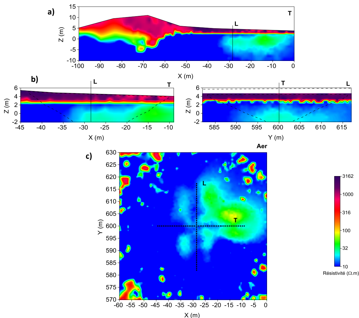
Figure 113. Modèle 'b', coupes d'inversion 3D - de la dune grise pour les mesures du 14 mars 2014 (lignes IRE croisées) après 7 itérations (erreur RMS de 28.7 %) : a) section transversale du milieu dunaire au niveau de la ligne transversale (Y = 600 m), b) Vues transversale à Y = 600 m et longitudinale à X = -28.5 m de la dune grise au niveau des lignes d'électrodes et c) vue aérienne de la dune grise à une altitude de Z = 1.5 m.
