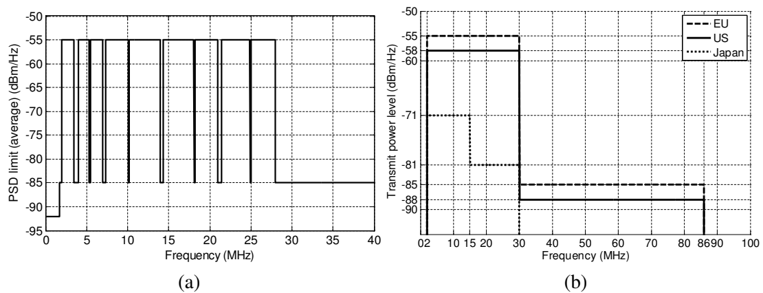
FIG. 4.2 – Niveau de DSP pour les systèmes CPL-BB. Illustration du notching permanent (a) et comparaison des réglementations en Europe, aux Etats-Unis et au Japon (b).
