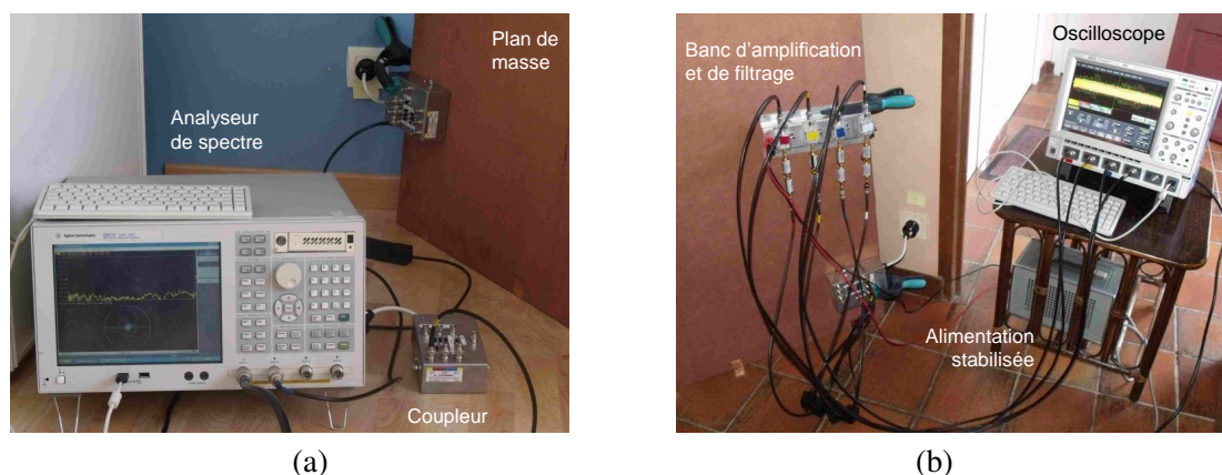
FIG. 3.3 – Equipements utilisés lors de la campagne ETSI STF 410. Mesure du canal (a) et mesure du bruit (b).
