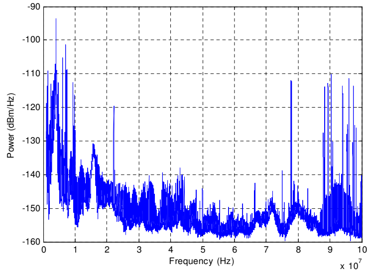
FIG. 2.6 – Exemple de bruit de fond CPL mesuré [102].
