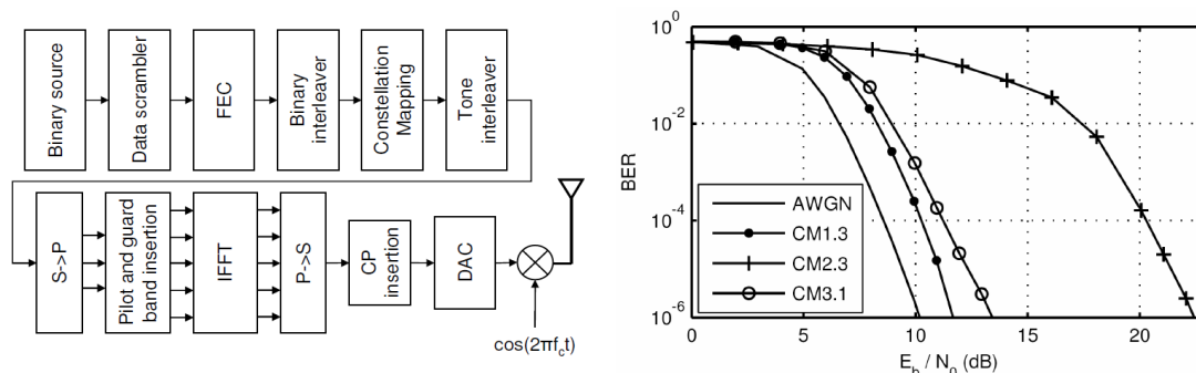
FIG. 2 – Système OFDM millimétrique proposé par France Telecom, et performances du système pour différents modèles de canal (CM1.3 : LOS, CM2.3 et CM3.1 : NLOS).
