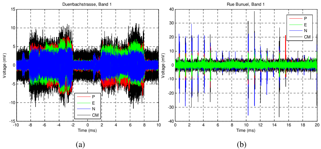
FIG. 3.13 – Signatures de bruit impulsif mesuré. Bruit impulsif périodique synchronisé (a) et bruit impulsif périodique asynchrone (b).
