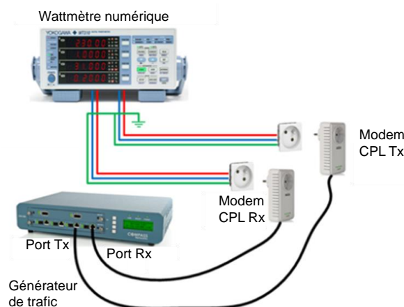
FIG. 6.3 – Montage expérimental de mesure de la consommation des modems CPL.
