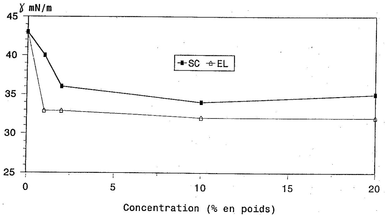
Graphique 25 : Tension superficielle obtenue par la méthode des angles de contacts, en fonction de la concentration en MF121 incorporée dans une matrice de PS. Support de W.
