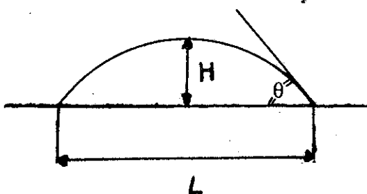
Fig.43 : Détermination de l'angle de contact.
