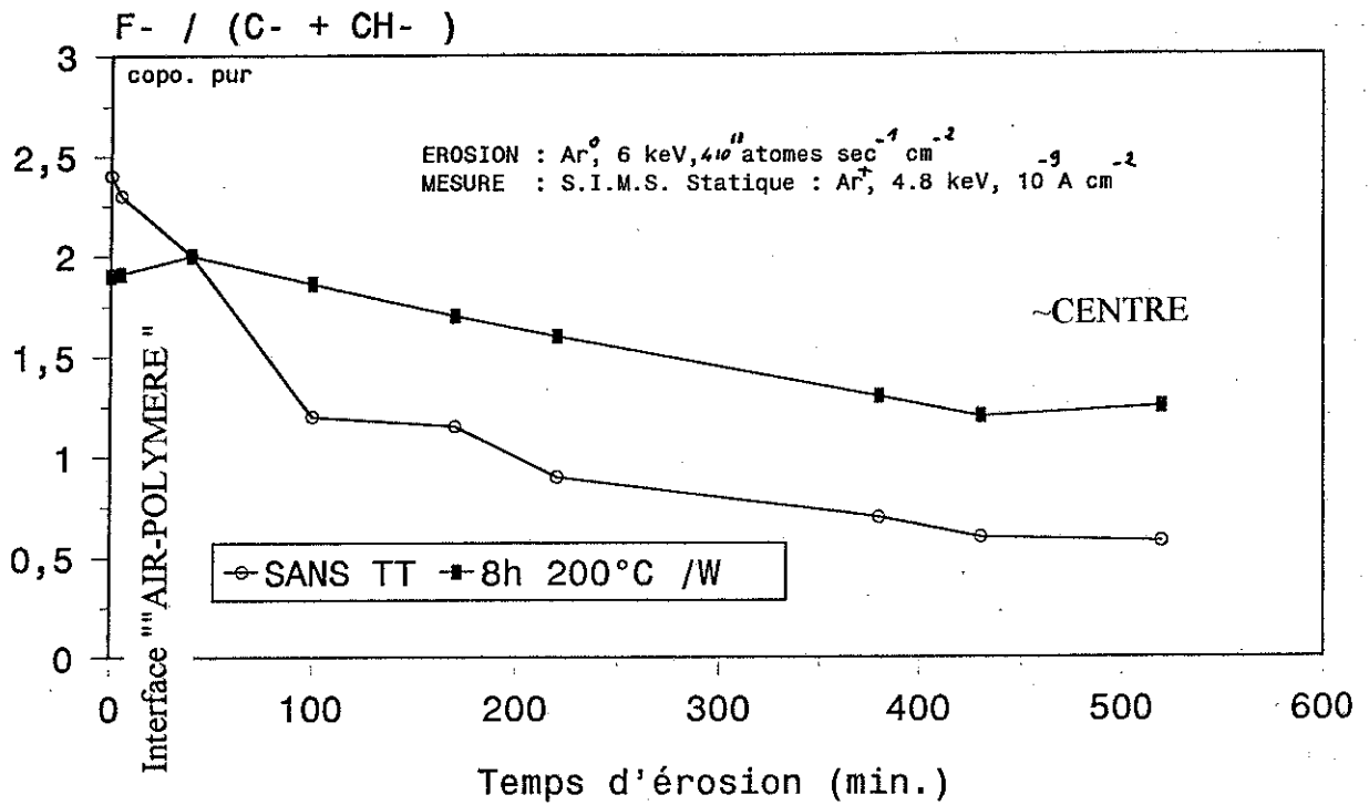
Graphique 5 : Profils de concentration semi-dynamiques de films contenant 10% en poids de MF121 incorporé dans une matrice de PMMA. Films déposés par E.L. sur un support de W (solvant : THF)
