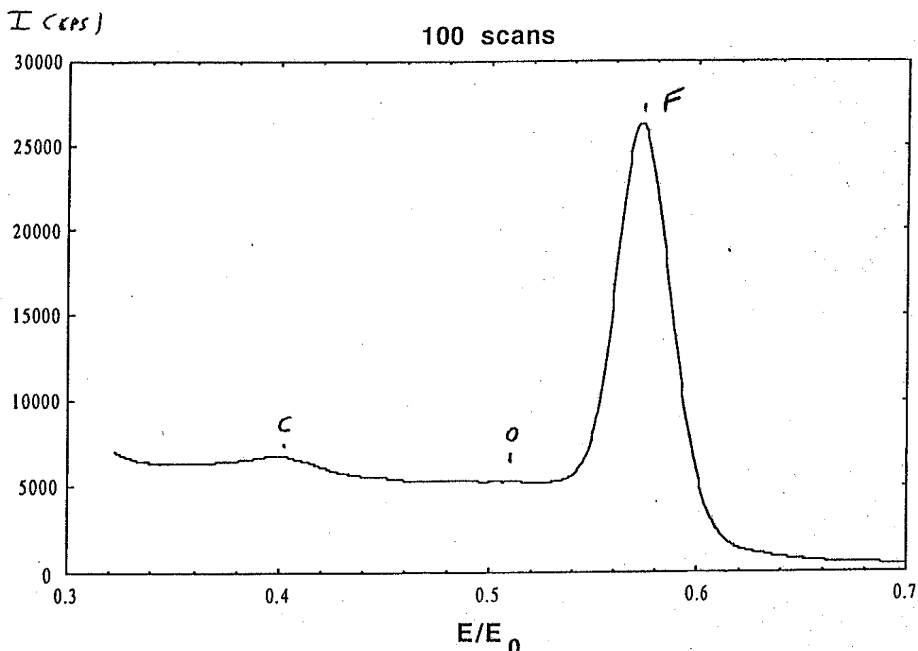
Graphique 50 : Spectre I.S.S. du copolymère MF111
