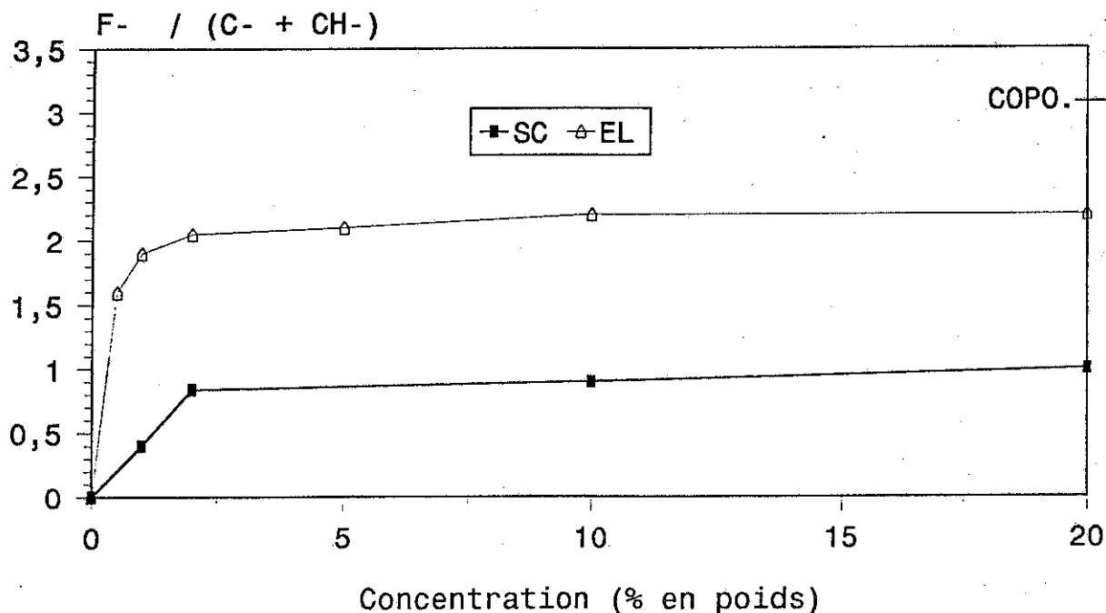
Graphique 21 : Rapport des intensités ioniques secondaires F - , C - , CH - (intensité de F - normalisée) à l'interface "air-polymère" en fonction de la concentration de MF121 incorporé dans une matrice de PS. Support W.
