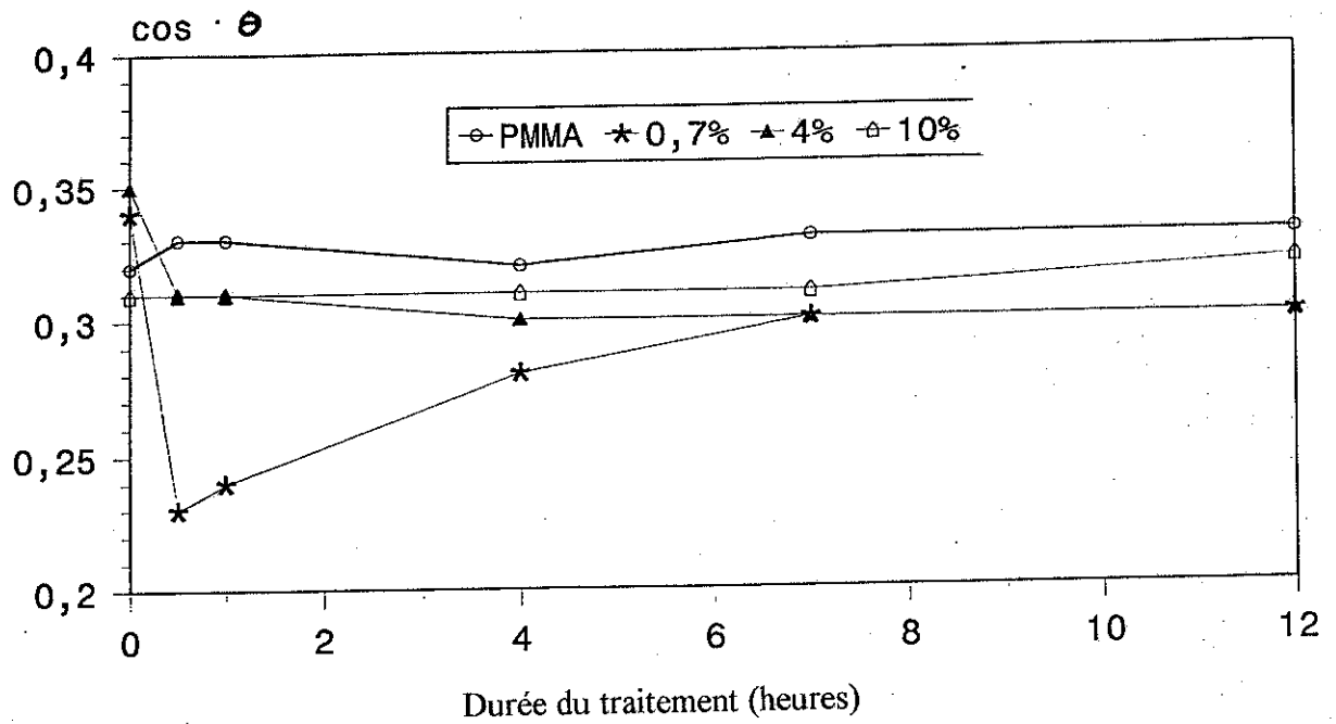
Graphique 68 : Angle de contact "eau-polymère" en fonction de la durée du traitement thermique (200°C, air). Plaques contenant divers % de MF73 incorporé dans une matrice de PMMA et formées par "malaxage-pressage".
