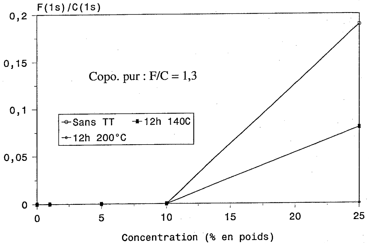
Graphique 34 : Rapport F/C obtenu par E.S.C.A à l'interface "air-polymère" en fonction de la concentration en MF121 incorporé dans une matrice de PMMA. Plaques préparées par "malaxage-pressage". Influence du traitement thermique (air).
