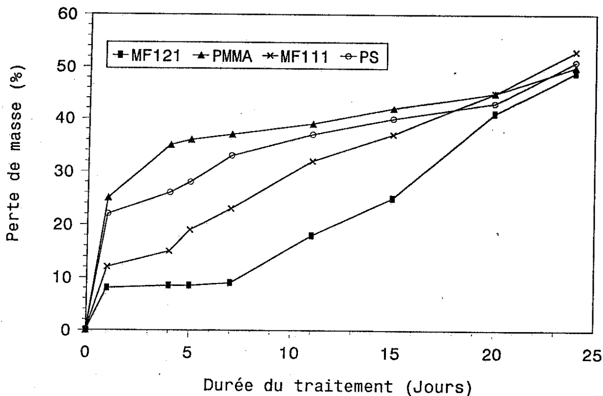
Graphique 16 : Thermogravimétrie à 200 °C en présence d'air
