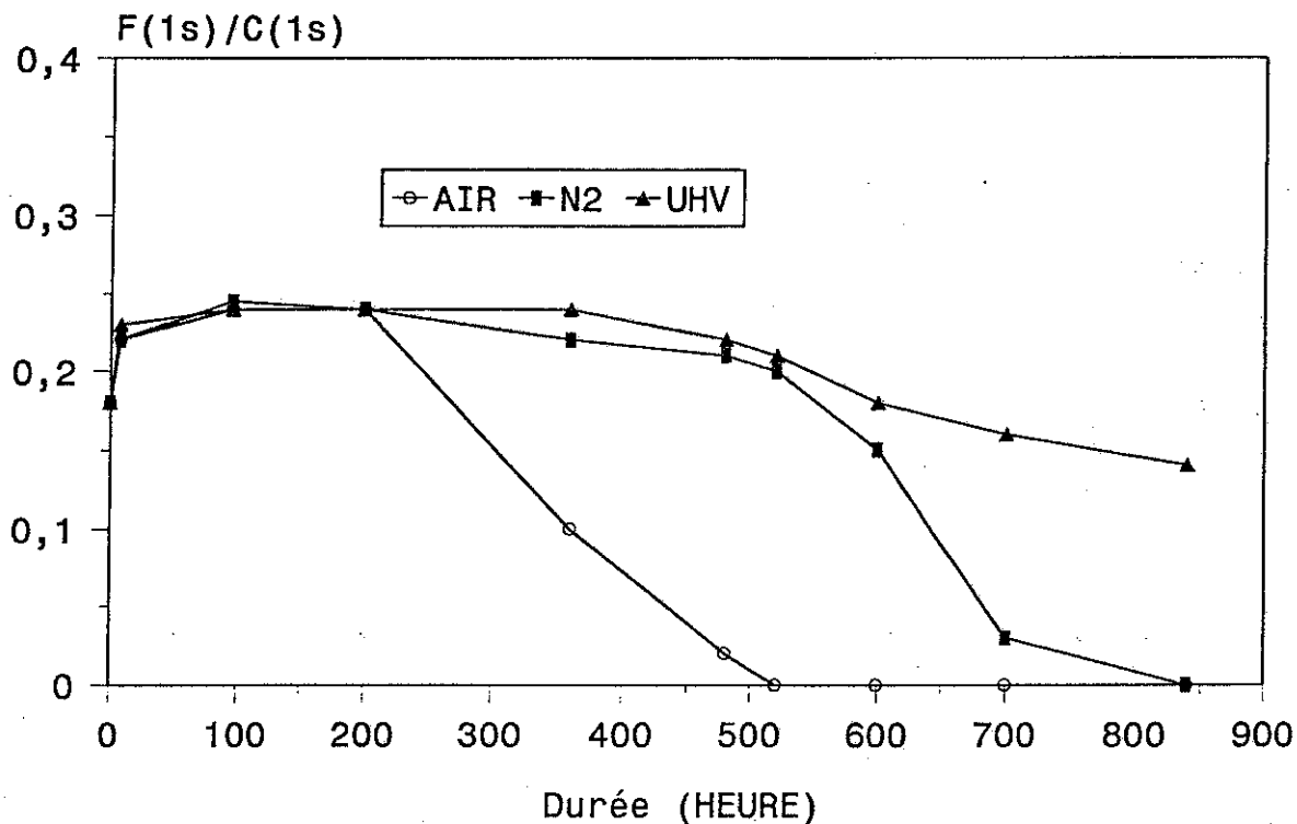
Graphique 32 : Rapport F/C obtenu par E.S.C.A à l'interface "air-polymère" en fonction de la durée du traitement thermique (200°C). Films déposés par S.C., contenant 10 % poids de MF121 incorporé dans une matrice de PS. Support W.
