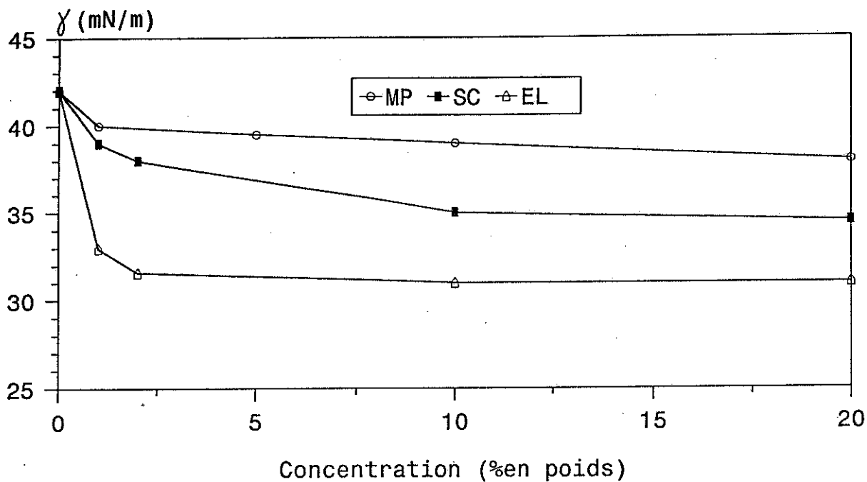
Graphique 11 : Tension superficielle obtenue par la méthode des angles de contact, en fonction de la concentration de MF121 incorporé dans une matrice de PMMA. Les échantillons sont soumis à un traitement thermique à 200°C pendant 8h. dans une étuve à air.
