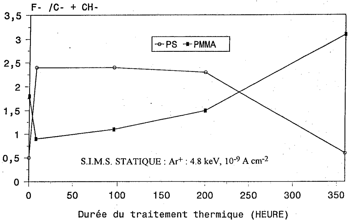
Graphique 14 : Rapport des intensités ioniques secondaires F - , C - , CH - (intensité de F - normalisée) en fonction de la durée du traitement thermique (200°C, air). Films contenant 10 % en poids de MF121 incorporé dans une matrice de PMMA ou de PS. Films déposés par S.C. Support W.
