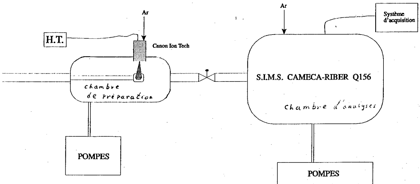
Fig. 49 : Schéma du dispositif utilisé en S.I.M.S. semi-dynamique
