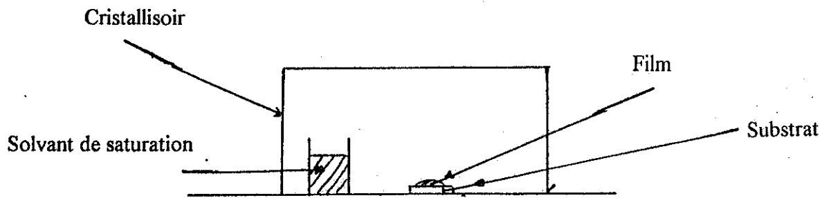
Fig.37. :Dispositif utilisé lors de la formation des films E.L.L.
