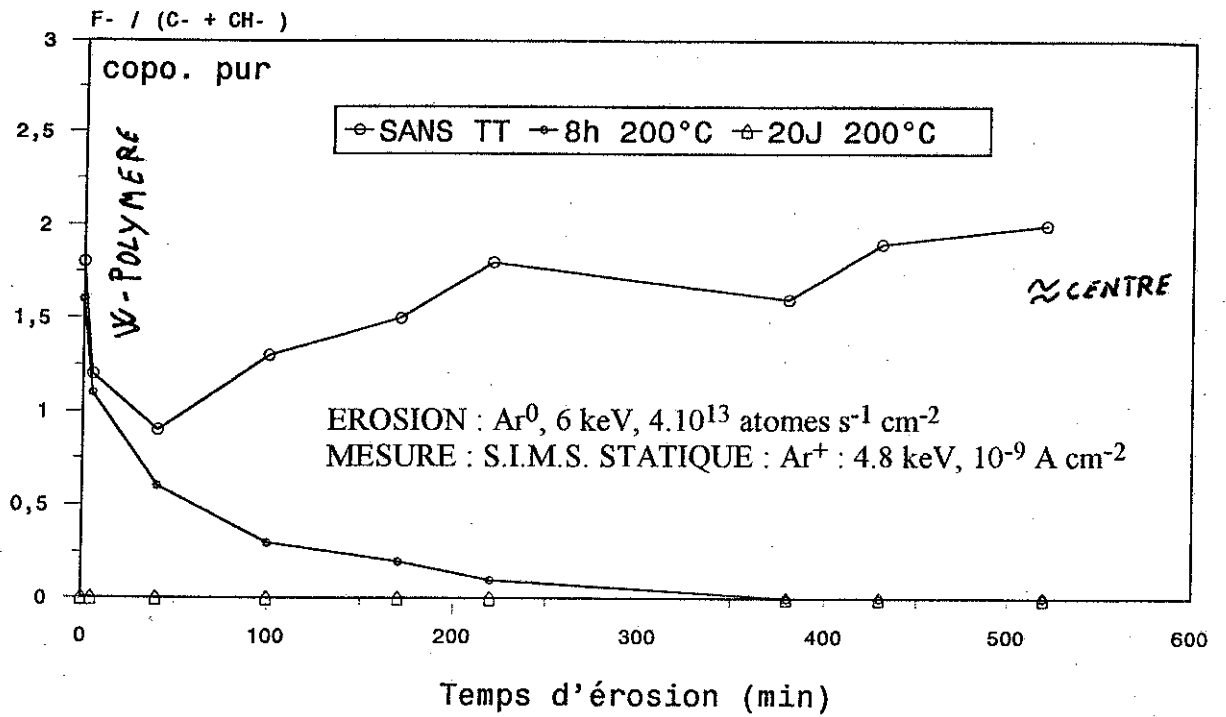
Graphique 28 : Profils de concentration semi-dynamiques, de films contenant 10 % en poids de MF121 incorporé dans une matrice de PS . Films déposés par E.L. sur un support de W. Influence de la durée du traitement thermique.
