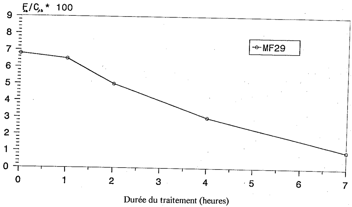
Graphique 74 : Rapport F/C obtenu par E.S.C.A à l'interface "air-polymère", en fonction de la durée du traitement thermique (200°C, air). Plaques contenant 5% en poids de MF29 incorporé dans une matrice de PS. Plaque formée par "malaxage-pressage"
