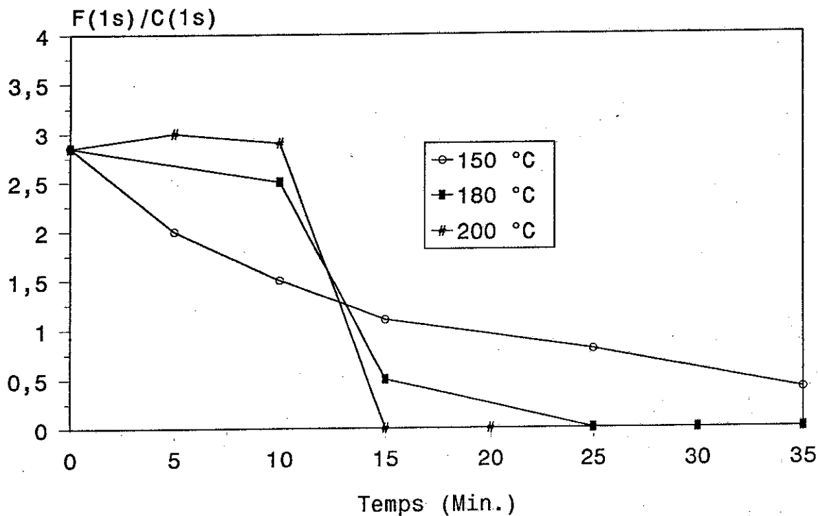
Graphique 12: Rapport F/C obtenu par E.S.C.A. en fonction de la durée et de la température du traitement thermique, sur des films contenant 10 % en poids de MF121 dans une matrice de PMMA. Films déposés par S.C. sur un support de W
