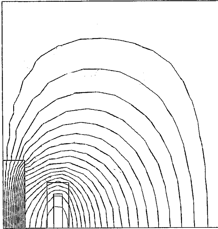
Figure III.17 Lignes équivalents du module de H .
