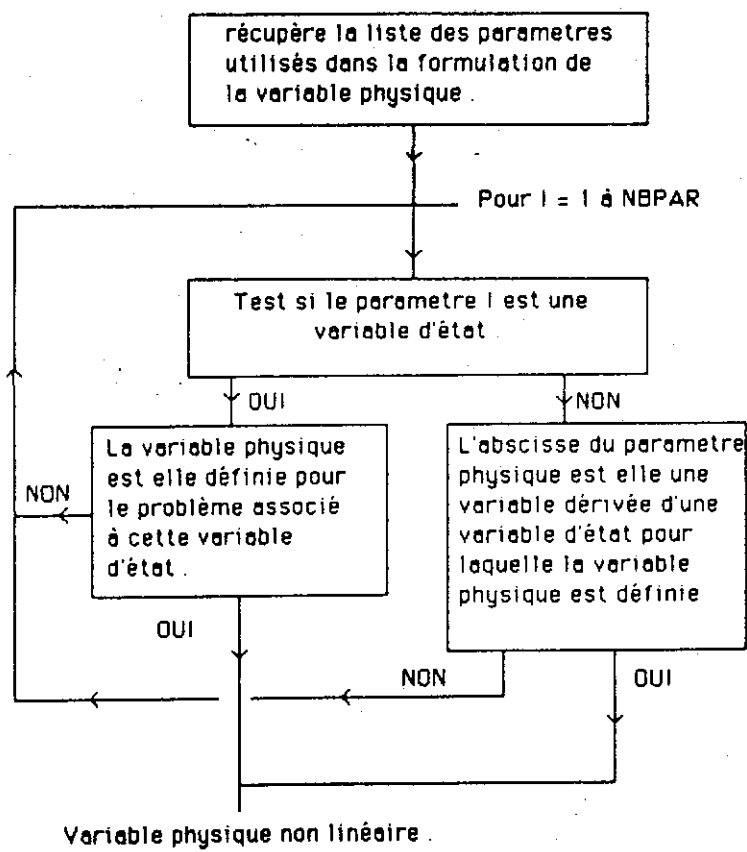
Figure II.15. Algorithme de test de la non linéarité d'une variable physique .
