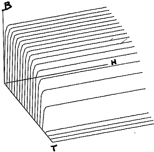
Figure 1.3 Surface de modélisation de la perméabilité magnétique .
