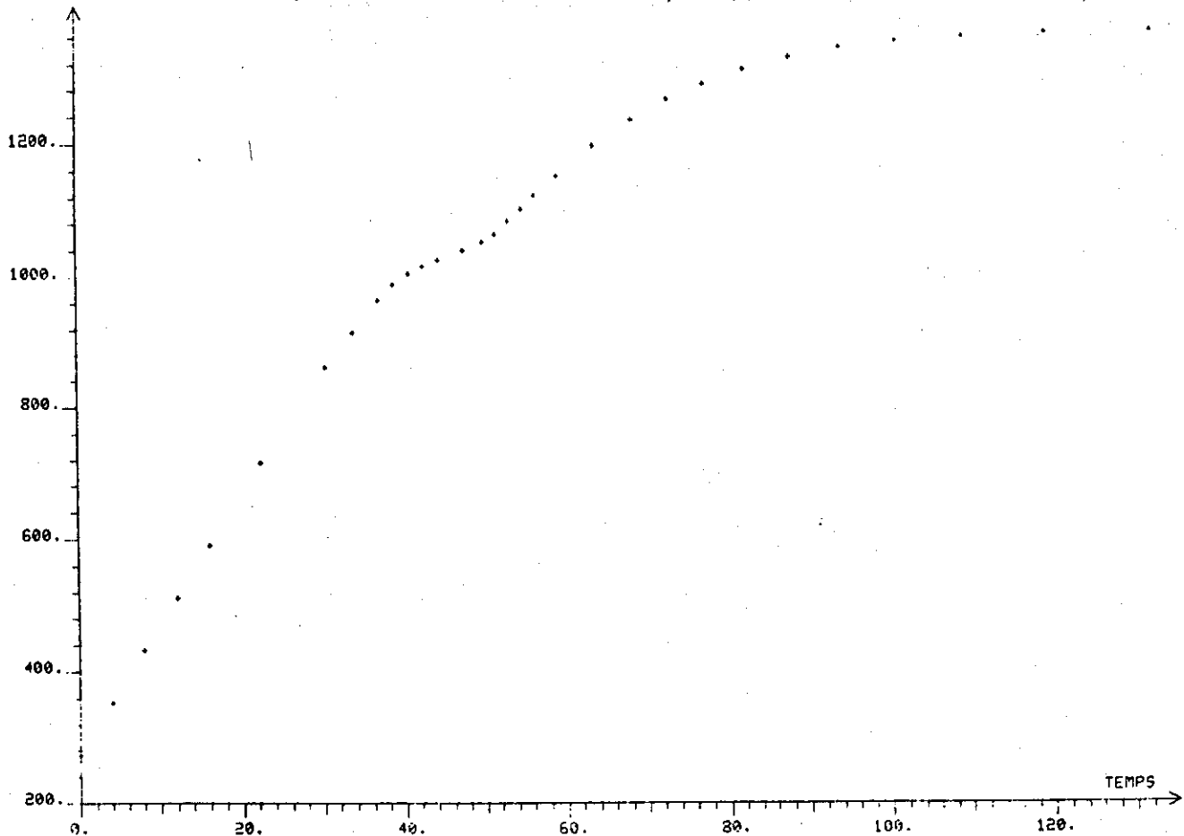
Figure II.1 Visualisation de l'évolution de la température avec passage du point de Curie. Chaque croix représente un instant de la simulation.
