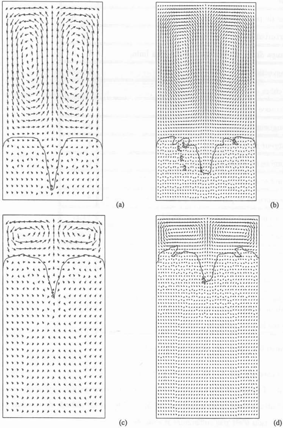
Figure 5-7: Cas 6. Cartes de vitesse et isovaleur de la fraction liquide \phi = 0.9 . .a) et b) t=5 min maillage 20 \times 30 ( v_{\max} = 13.28 \text{ mm/sec} ) et 40 \times 60 ( v_{\max} = 15.4 \text{ mm/sec} ) respectivement, c) et d) t=15 min, maillage 20 \times 30 ( v_{\max} = 3.0 \text{ m/sec} ) et 40 \times 60 ( v_{\max} = 1.7 \text{ mm/sec} ).
