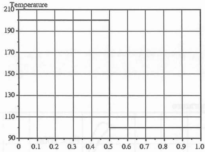
Figure A-2: Solution exacte, Température dans l'axe x.
