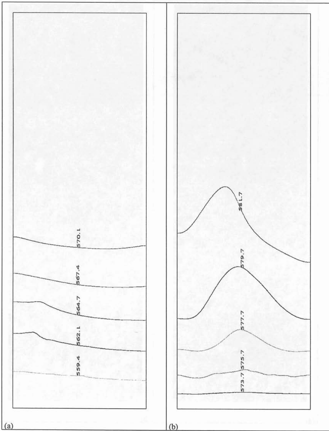
Figure 4-11: Isothermes a) cas 12, 20 minutes après le début de la solidification, b) cas 9, 5 minutes après le début de la solidification.
