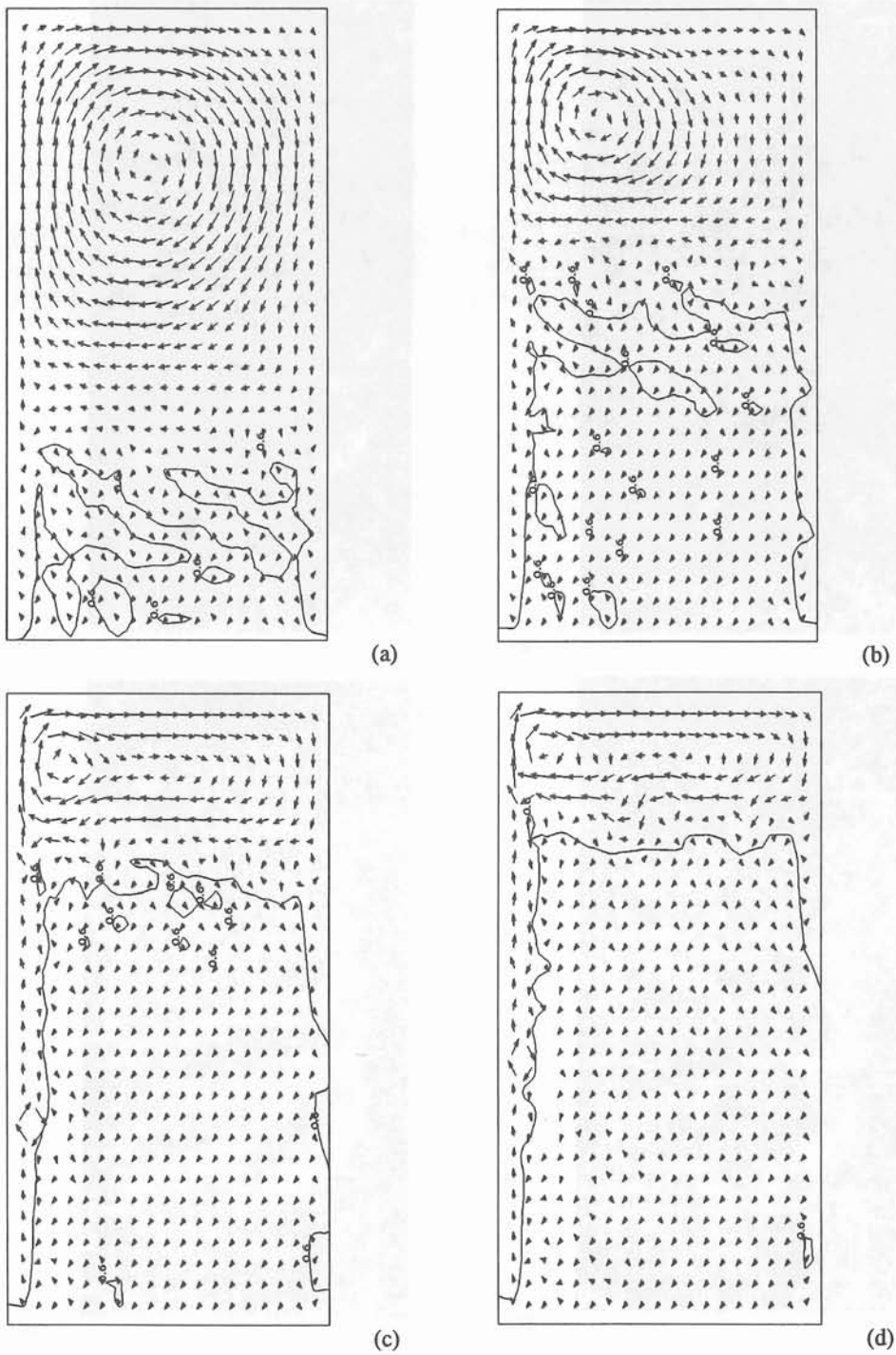
Figure 5-5: Cas 5B. Cartes de champ de vitesses et isovaleur de la fraction liquide \phi = 0.6 . a) 5 min ( v_{\max} = 7.6\text{mm/sec} ); b) 10 min ( v_{\max} = 4.3\text{mm/sec} ); c) 15 min ( v_{\max} = 2.5\text{mm/sec} ); d) 20 min ( v_{\max} = 1.7\text{mm/sec} ) après le début de la solidification.
