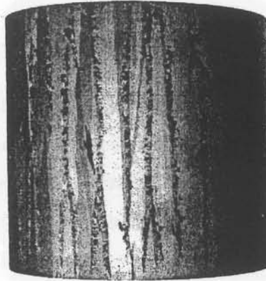
Figure 1-1: Ségrégations en canaux dans un lingot de Mar-M200 (diam. 4 in) d'après Giamei et al. [36].
