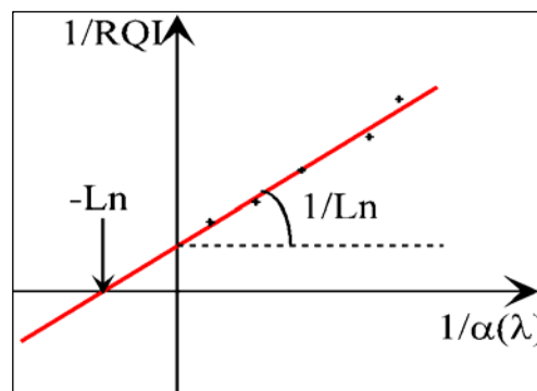
Figure C-4 Détermination graphique de la longueur de diffusion
