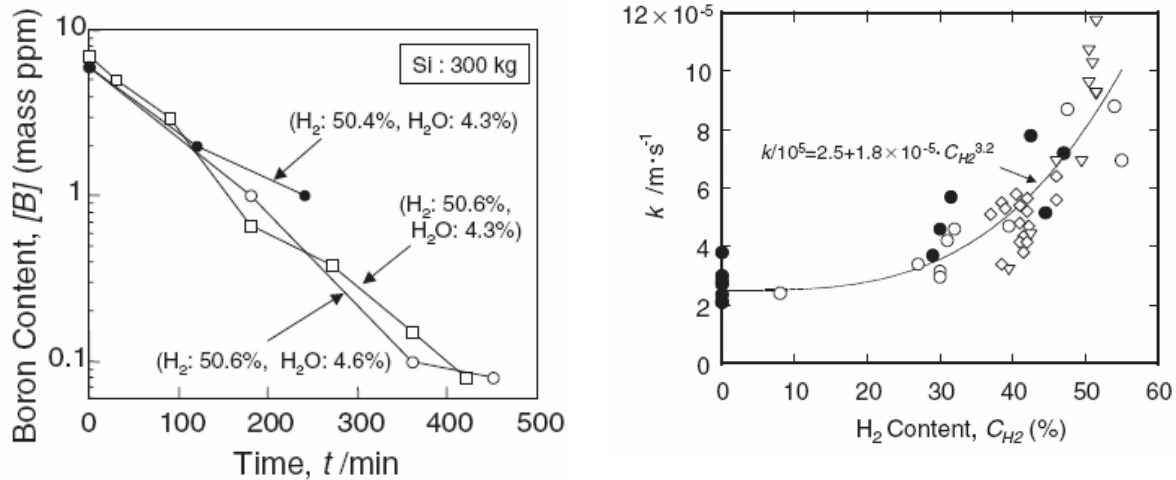
Figure IV-7 teneur en bore en fonction du temps de traitement (à gauche) et constante de vitesse de la réaction de volatilisation du bore en fonction du pourcentage d'hydrogène dans le plasma (à droite) [2]
