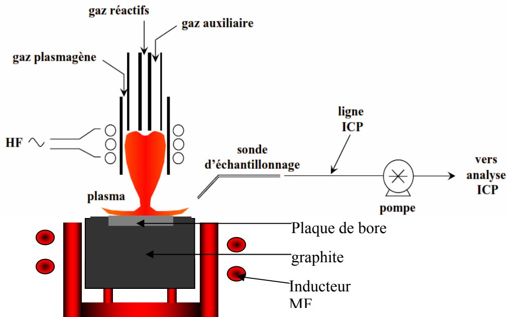
Figure V-38 Dispositif expérimental utilisé pour l'attaque du graphite par un plasma argon-oxygène-hydrogène.
