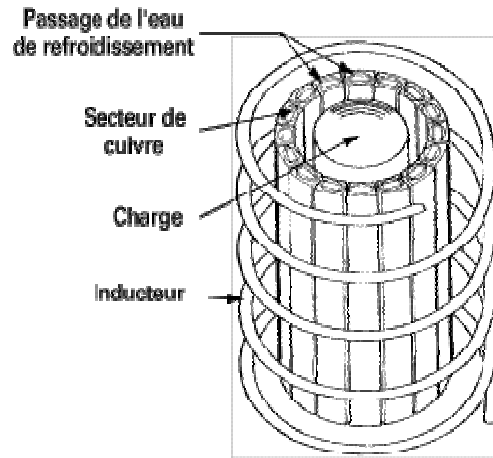
Figure V-7 Creuset froid sectorisé + inducteur [100]
