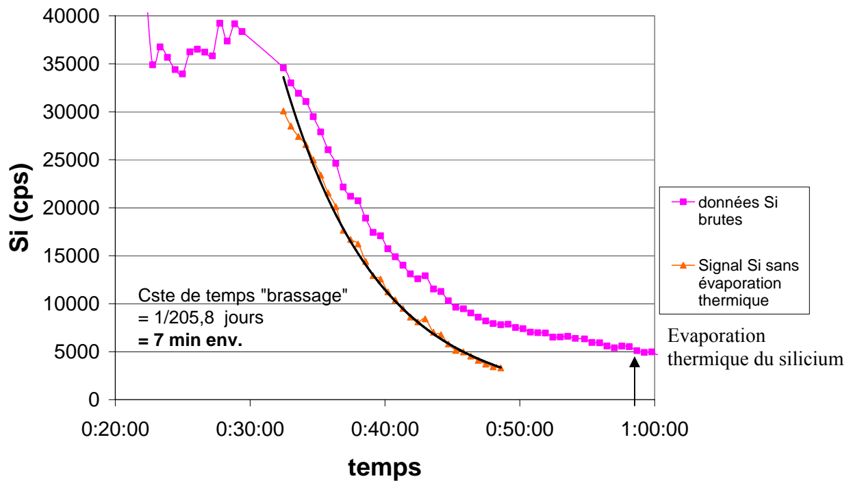
Figure V-20 Désoxygénation du silicium sous plasma d'argon.
