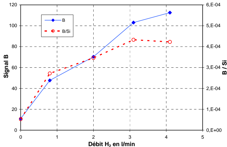
Figure IV-28 Effet du débit d'hydrogène sur l'évaporation du bore, à débit d'oxygène constant.
