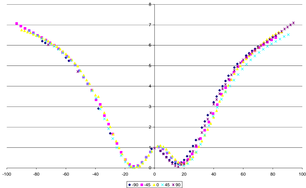
Figure V-29 Coupe de PS50 avec des angles de -90^\circ , -45^\circ , 0^\circ , 45^\circ , 90^\circ
