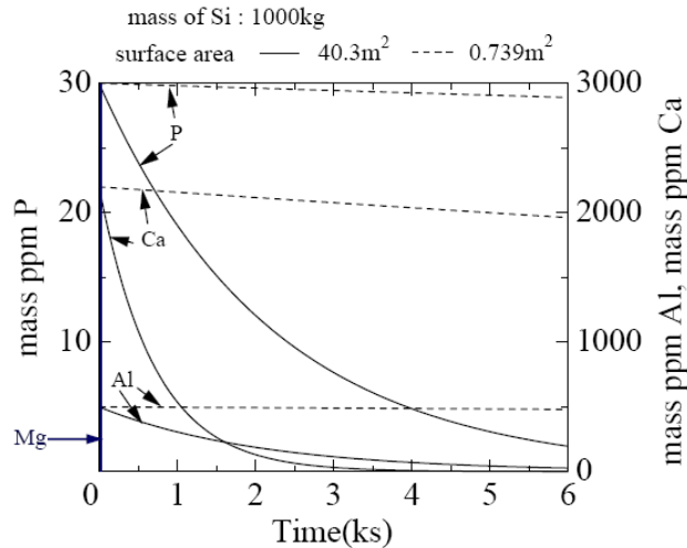
Figure IV-3 Relation entre le temps de traitement sous vide et la concentration en phosphore, aluminium et calcium pour un silicium calculs à 1823K [49]
