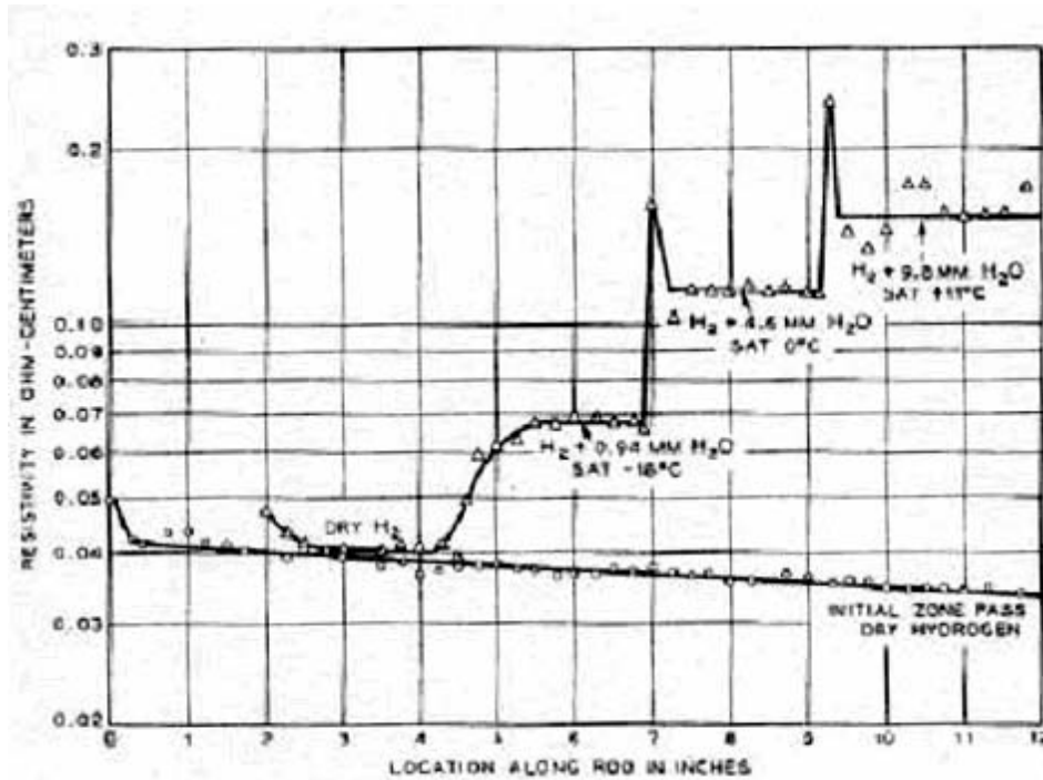
Figure IV-6 Volatilisation du bore avec de l'hydrogène sec ou humide, évolution de la résistivité du matériau en fonction des débits de H 2 O [76]
