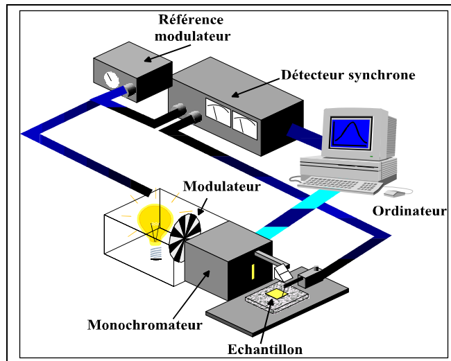
Figure C-5 Schéma synoptique de l'appareillage de mesure de longueur de diffusion
