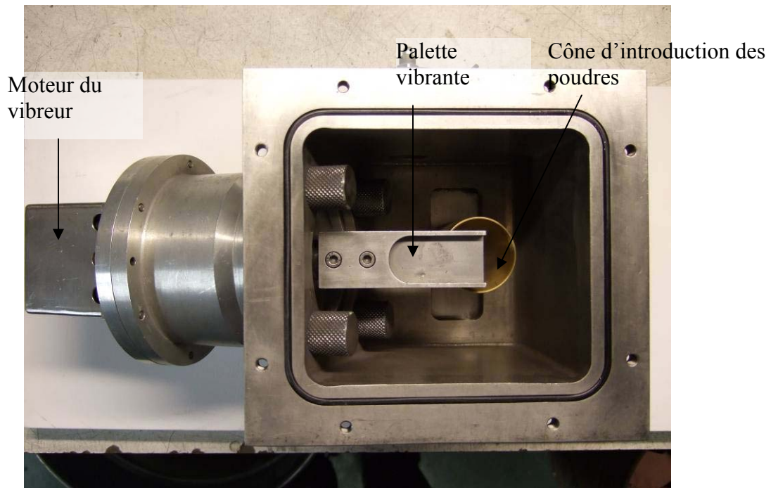
Figure V-9 Vue de dessus de la partie inférieure du distributeur de poudre
