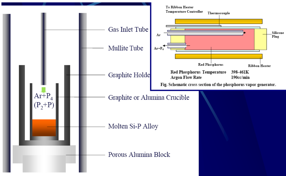
Figure IV-9 Dispositif expérimental de Miki et al. pour déterminer l'énergie de Gibbs de dissolution du phosphore [49]
