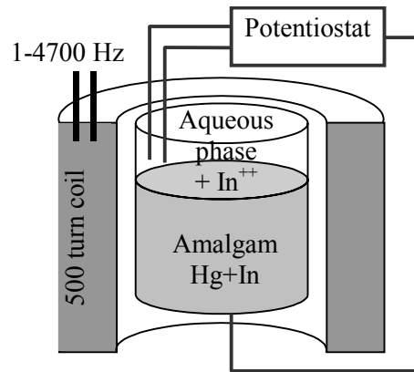
Figure V-11 étude du transfert de masse d'un mélange de mercure et d'indium [103]
