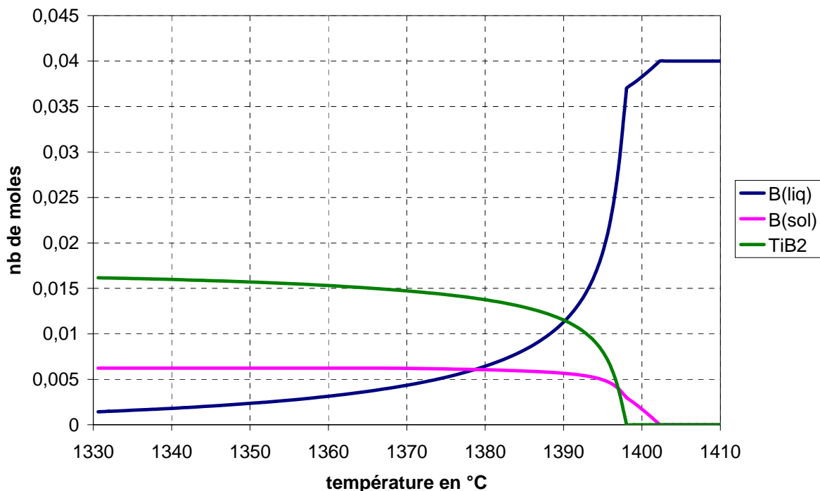
Figure IV-12 : forme du bore au cours d'une solidification de type SCHEIL, (calcul effectué avec les teneurs du tableau IV-1)
