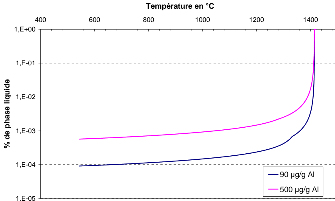
Figure IV-18 Effet de l'ajout d'aluminium sur la quantité de phase liquide en fonction de la température (teneur en Al = 90 ou 500 µg/g).
