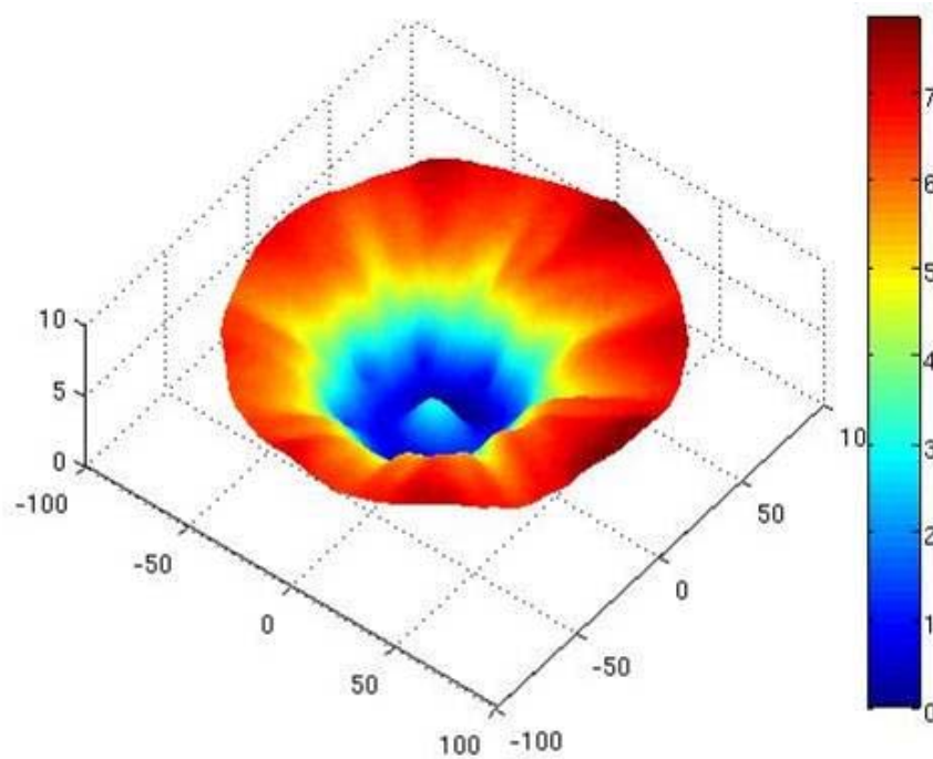
Figure V-27 Vue 3D du profil du disque de graphite gravé au cours de l'essai PS47
