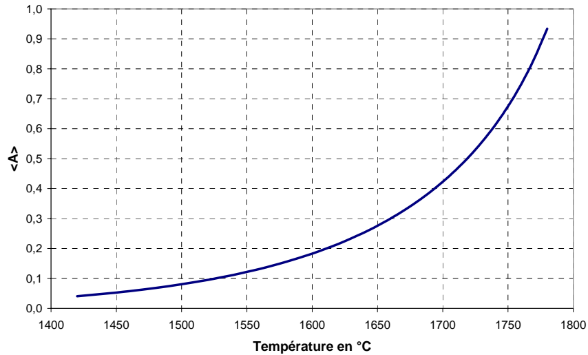
Figure IV-15 Seuil d'apparition de la couche de \text{Si}_3\text{N}_4 en fonction de la température (700 Si + 1 Ar + <A> \text{N}_2 )
