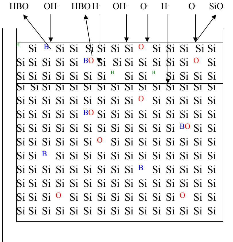
Figure IV-30 Schéma des réactions chimiques possibles à l'interface silicium liquide-plasma (Ar + H 2 + O 2 )
