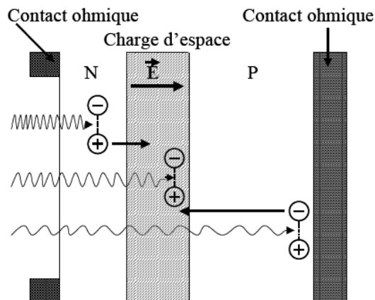
Figure III-15 Schéma de structure d'une cellule photovoltaïque
