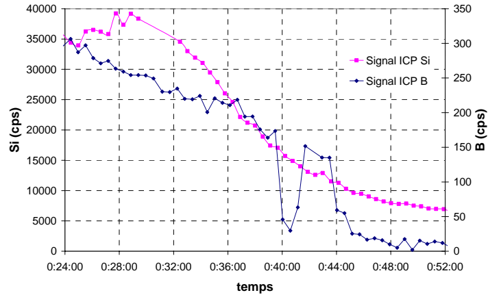
Figure IV-26 Evolution de l'intensité des signaux ICP-OES du bore et de l'oxygène pour un traitement sous Ar + H 2 .
