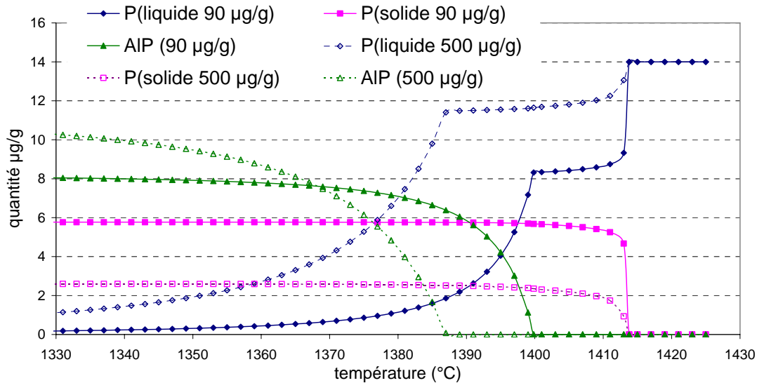
Figure IV-17 Effet de l'ajout d'aluminium sur la ségrégation du phosphore (teneur en Al = 90 ou 500 µg/g, teneur en P = 14 µg/g).
