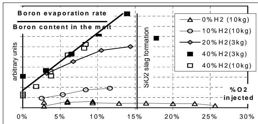
Figure IV-27. H 2 /O 2 effet sur l'évaporation du bore [81].
