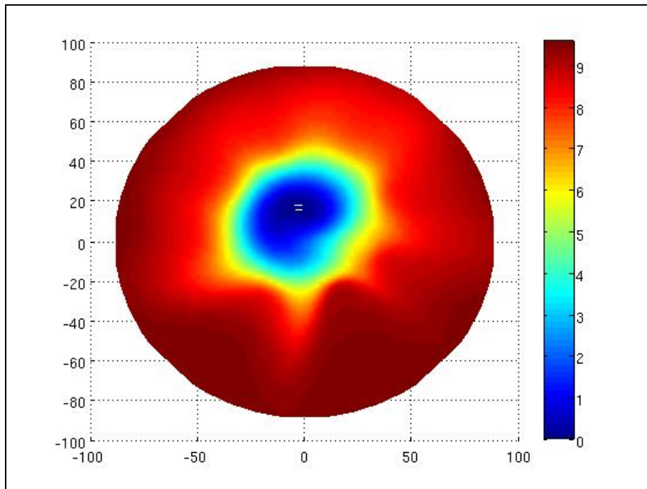
Figure V-28 Vue 2D du disque de graphite gravé au cours de l'essai PS53
