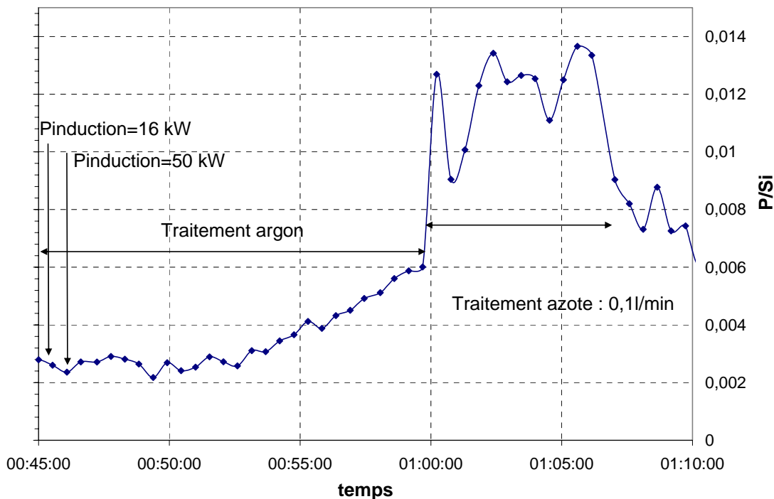
Figure IV-24 Evolution du rapport P/Si dans un creuset graphite de diamètre 55 mm
