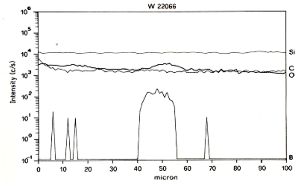
Figure VI-1 : Profils SIMS de B, C et O dans du silicium multicristallin d'après S.Pizzini [101].
