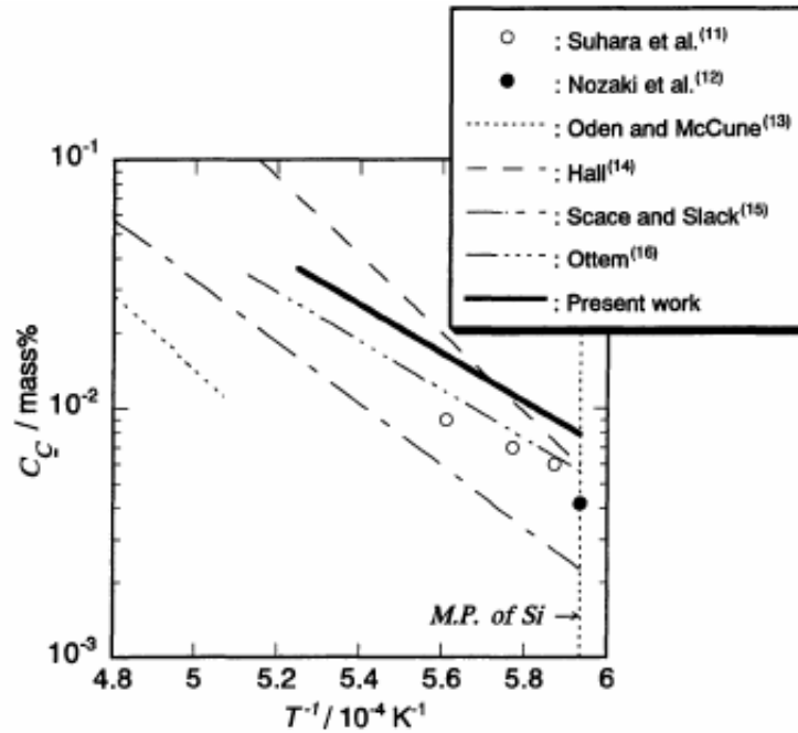
Figure IV-10 Solubilité du carbone dans le silicium en équilibre avec SiC [88].
