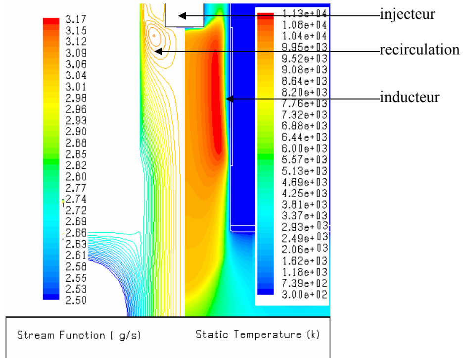
Figure V-40 Champ de vitesse et de température dans notre torche à plasma d'argon pur P_{\text{«réelle»}}=20 kW débit plasmagène 80 l/min [113].
