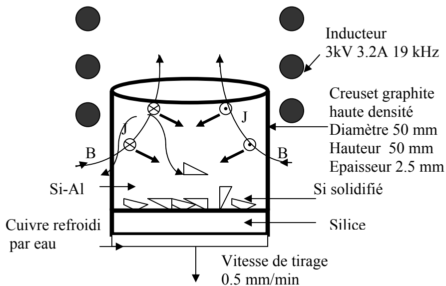
Figure IV-25 dispositif expérimental utilisé pour les essais de ségrégation
