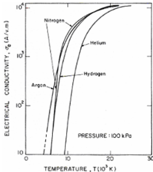
Figure V-3 Evolution de la conductivité électrique des plasmas (d'argon, hélium, azote et hydrogène) en fonction de la température [99]
