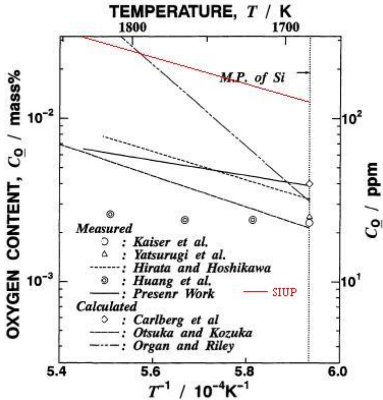
Figure IV-11 Evolution de la solubilité de l'oxygène en fonction de la température du silicium liquide [89]
