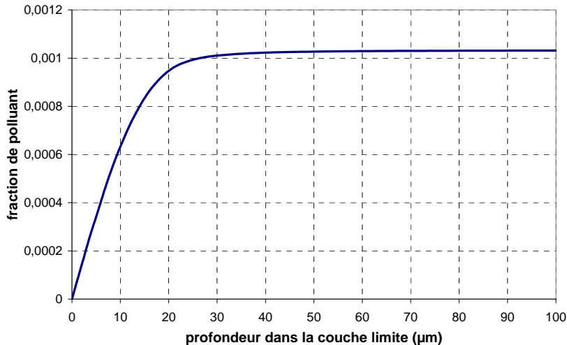
Figure V-14 Evolution de la fraction de polluant dans les 100 µm sous la surface du silicium liquide.
