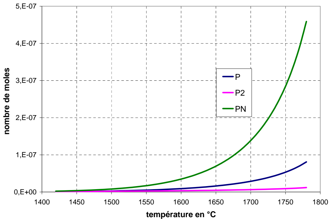
Figure IV-16 Phosphore évaporé en limite de formation de la couche de \text{Si}_3\text{N}_4 (700 Si + 0.0014 P + 1 Ar + <A> \text{N}_2 )
