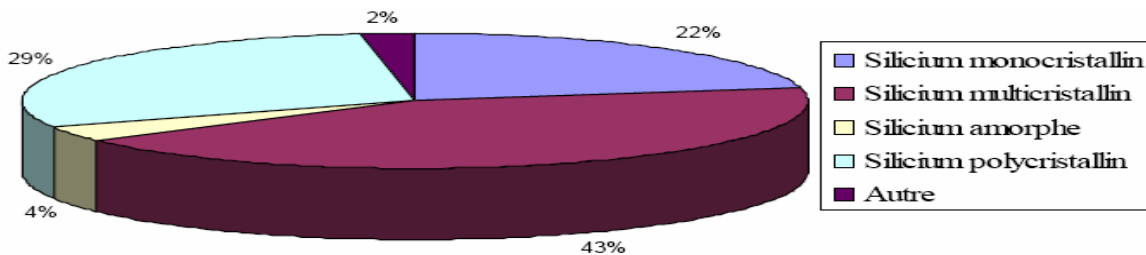
Figure 3 : Répartition en pourcentage de puissance électrique, des différentes filières de cellules photovoltaïques produites en 2005. D'après [3].
