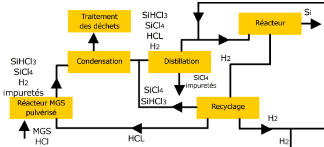
Figure III-7 Cycle de distillation du composé de silicium chloré [35]
