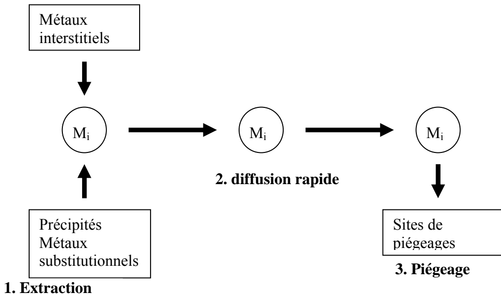
Figure III-16 Schéma du mécanisme de l'effet getter
