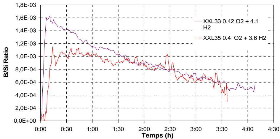
Figure V-43 Différentes cinétiques d'élimination du bore.
