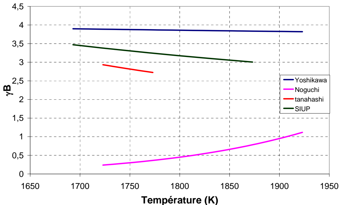
Figure IV-8 : Comparaison des coefficients d'activité du bore dans le silicium liquide proposés par différents auteurs.
