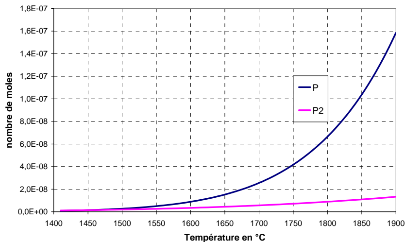
Figure IV-14 Forme du phosphore évaporé pour (700 Si + 0.0014 P + 1 Ar)
