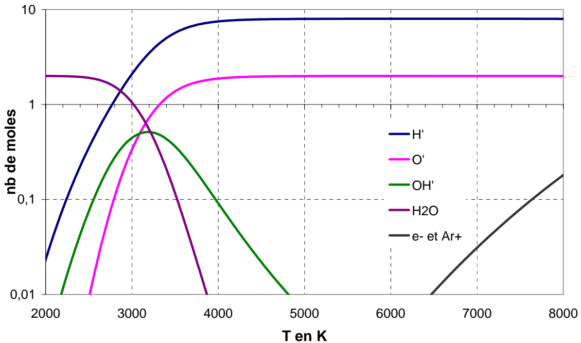
Figure IV-29 Espèces présentes dans un plasma. Calcul effectué avec 100 mol Ar + 4 mol H 2 + 1 mol O 2
