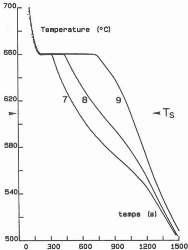
Figure 4. 17- Thermogramme dans un même plan horizontal ( z = 187 mm), alliage 1050 brassé à 600 A. T_S : température de solidus.
