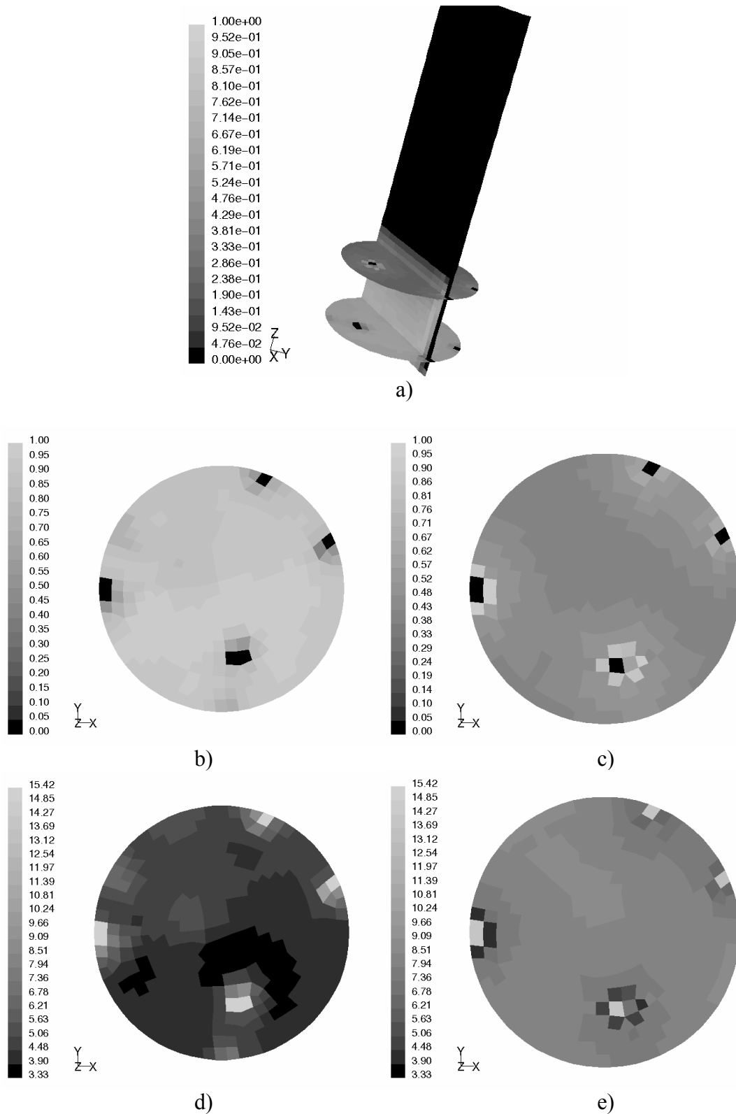
Figure 22: a) Fraction solide dans une section verticale ; b), c) Fraction solide et d), e) concentration moyenne dans deux sections transversales (situées à h = 1.5\text{mm} respectivement h = 7\text{mm} de la base du creuset), à t = 800\text{s} du début de la solidification.
