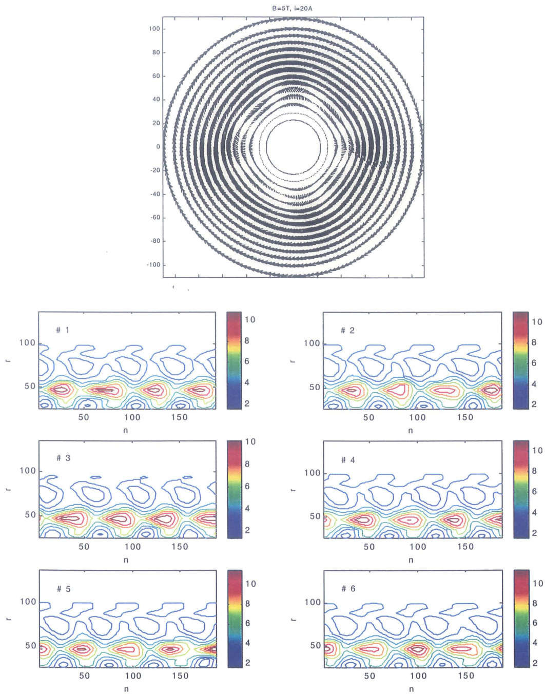
Figure 4.16 : Champ de vitesse sur un tour et champs de vorticité sur 6 tours obtenus pour B = 5 T et I = 20 A.
