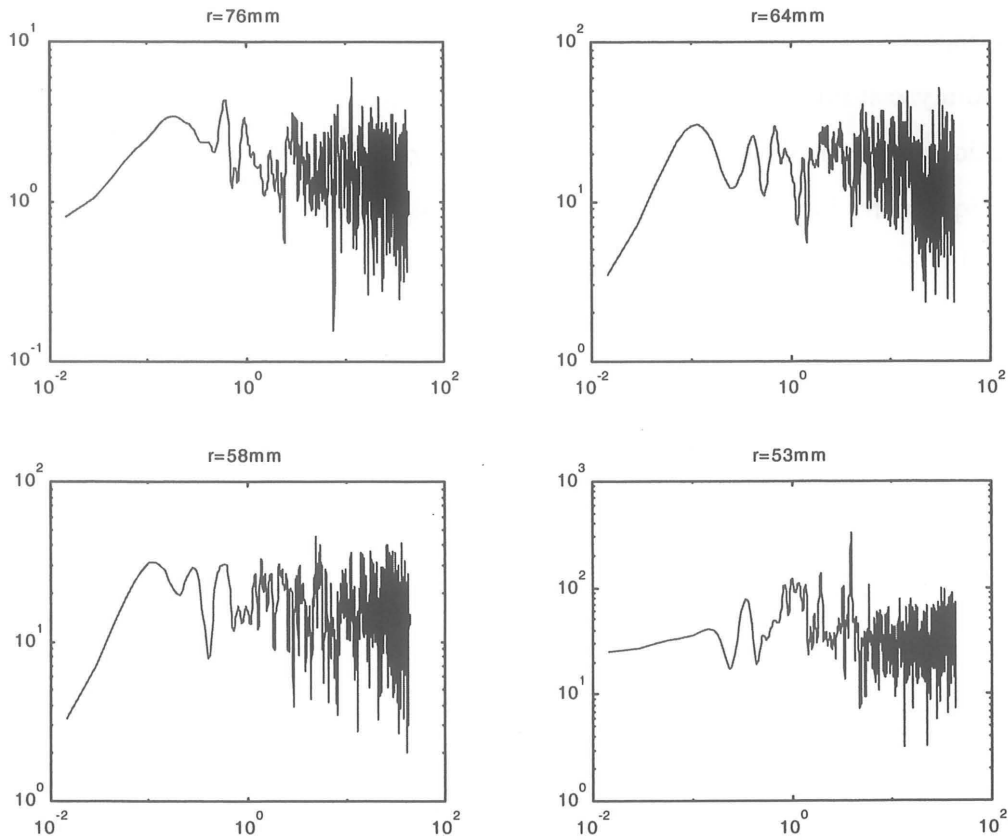
Figure 5.1 : Exemple de spectres de fluctuations de la température pour B = 1 \text{ T} et I = 30 \text{ A} en différents points dans la couche cisailée.
