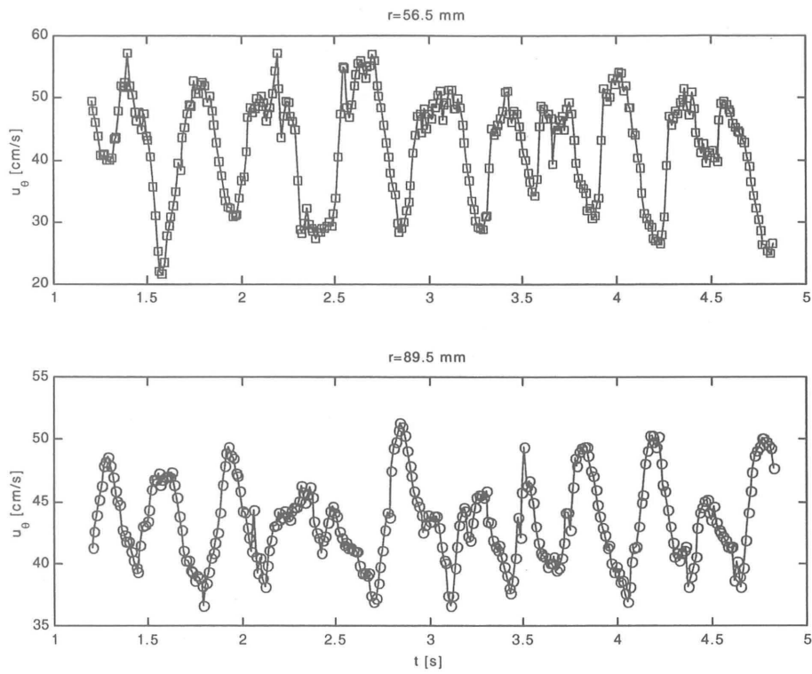
Figure 4.9 : Signaux de u_\theta mesurés à l'intérieur ( r = 56.5 mm) et à l'extérieur de la couche cisailée ( r = 89.5 mm).
