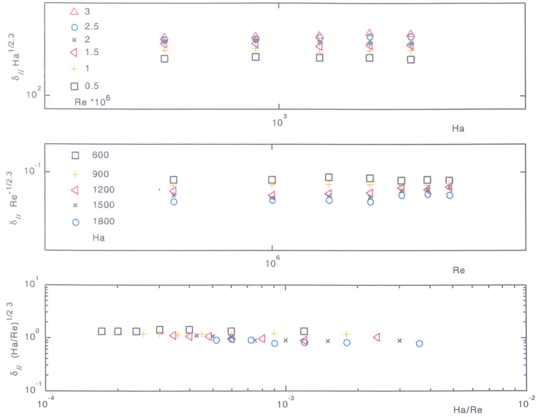
Figure 3.4 : Evolution de l'épaisseur de la couche cisailée libre \delta_{\parallel} en représentation Log-Log. (a) \delta_{\parallel} \times Ha^{1/2.3} en fonction de Ha , (b) \delta_{\parallel} \times Re^{-1/2.3} en fonction de Re et (c) \delta_{\parallel} \times \left(\frac{Ha}{Re}\right)^{1/2.3} , suggérant la loi \delta_{\parallel}/h \simeq 1 \times \left(\frac{Ha}{Re}\right)^{-1/2.3}
