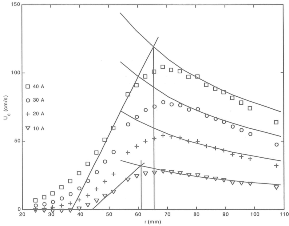
Figure 3.3 : Exemple de construction servant à définir l'épaisseur de la couche cisailée libre. B = 3 \text{ T} , R_i = 54 \text{ mm} et I = 10, 20, 30 et 40 \text{ A} .
