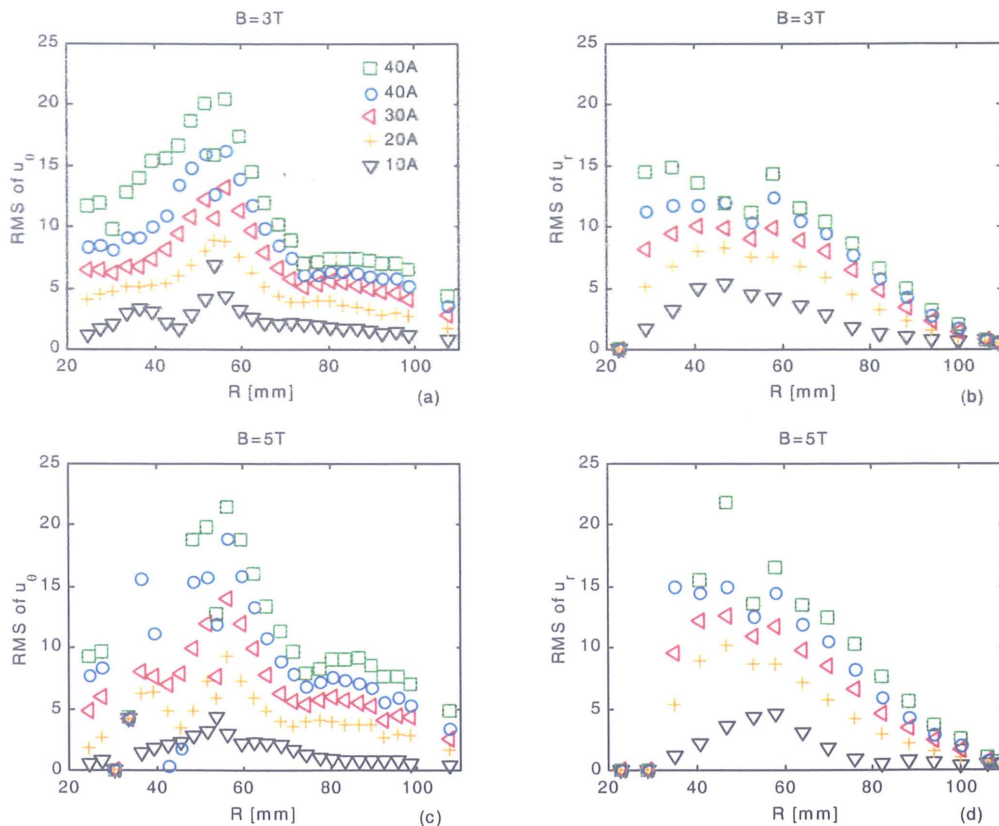
Figure 4.1 : Distributions radiales des RMS. (a et b) B = 3 \text{ T} , (c et d) B = 5 \text{ T} . R_i = 54 \text{ mm} .
