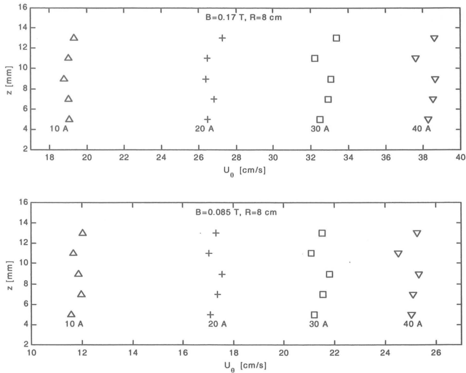
Figure 3.6 : Profils verticaux de la vitesse azimuthale.
