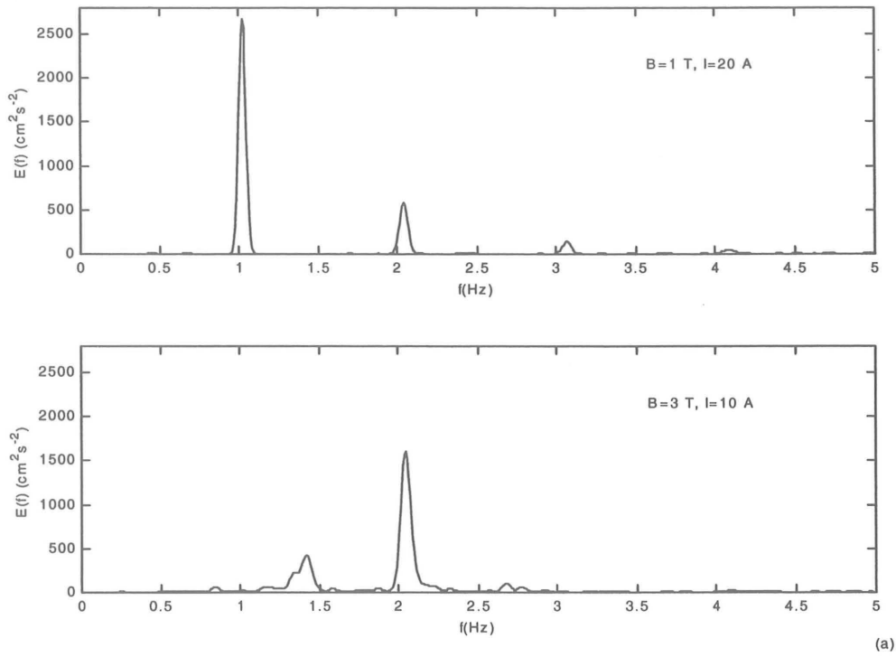
Figure 4.4 : Spectres temporels linéaires de u'_0 à r \simeq 68.5 mm. Les pics à basse fréquence sont la signature de structures cohérentes.
