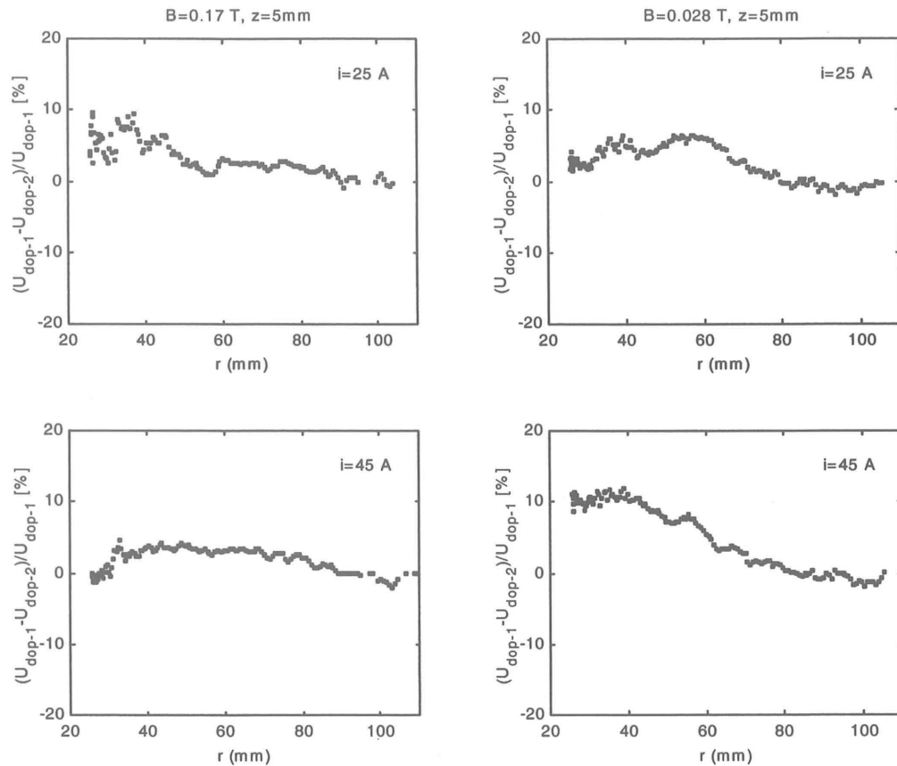
Figure 2.11 : Ecart relatif U_1 - U_2 / U_1 (%) entre deux séries de mesures pour deux valeurs de champ et deux valeurs du courant ( B = 0.17 et 0.028 T et I = 25 et 45 A).
